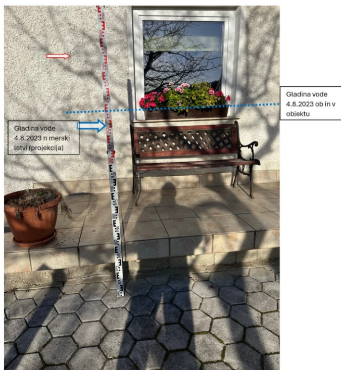
Slika 3: Objekt Letuš 110a. Sledi visoke vode 4. avgusta 2023. Globina vode znotraj objekta je bila višja od 0,8 m, zunaj objekta pa med 1,25 in 1,8 m. Z rdečo puščico je označena razpoka na objektu, ki je posledica diferenčnih deformacij temeljnih tal.
