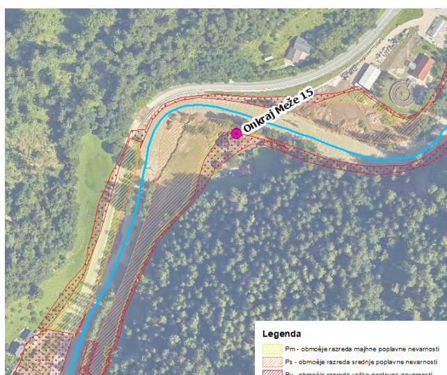
Slika 6: Situacijski prikaz objekta z inokraj Meže 15
