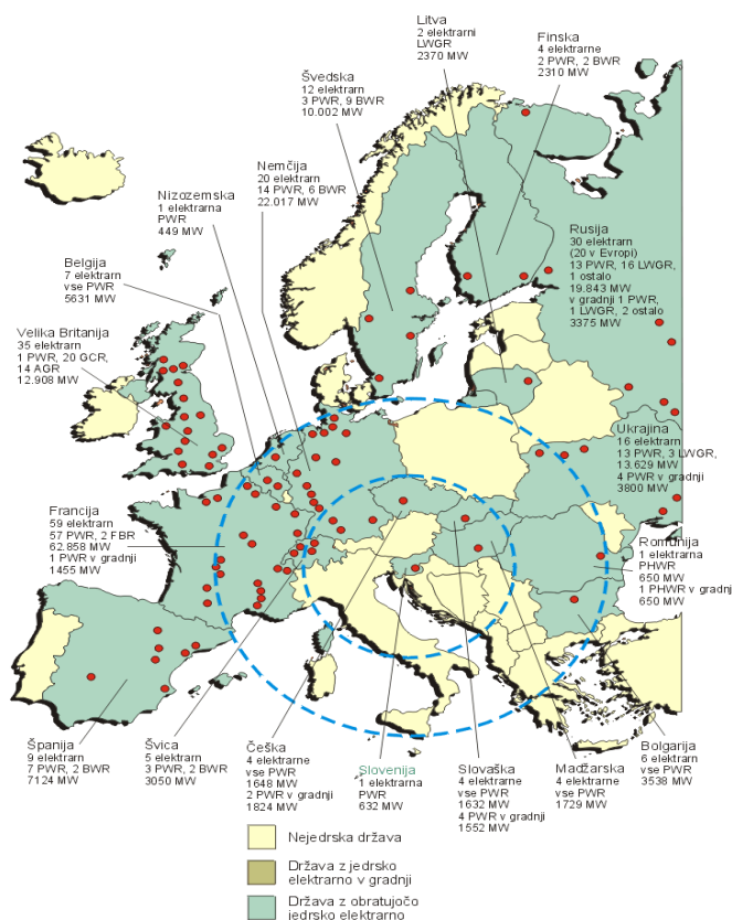
Slika 3: Jedrske elektrarne iz 1000 km območja oddaljene od SLO
