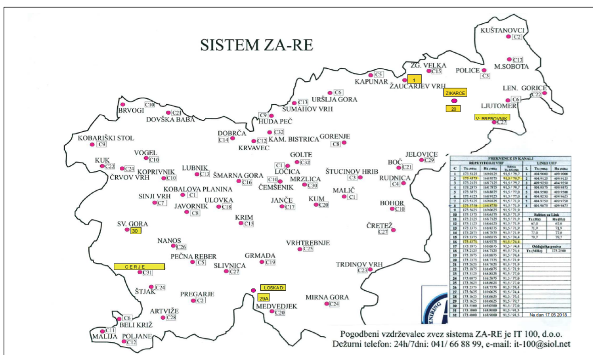
Slika 7: Repetitorske postaje s kanali sistema ZA-RE (2018)
