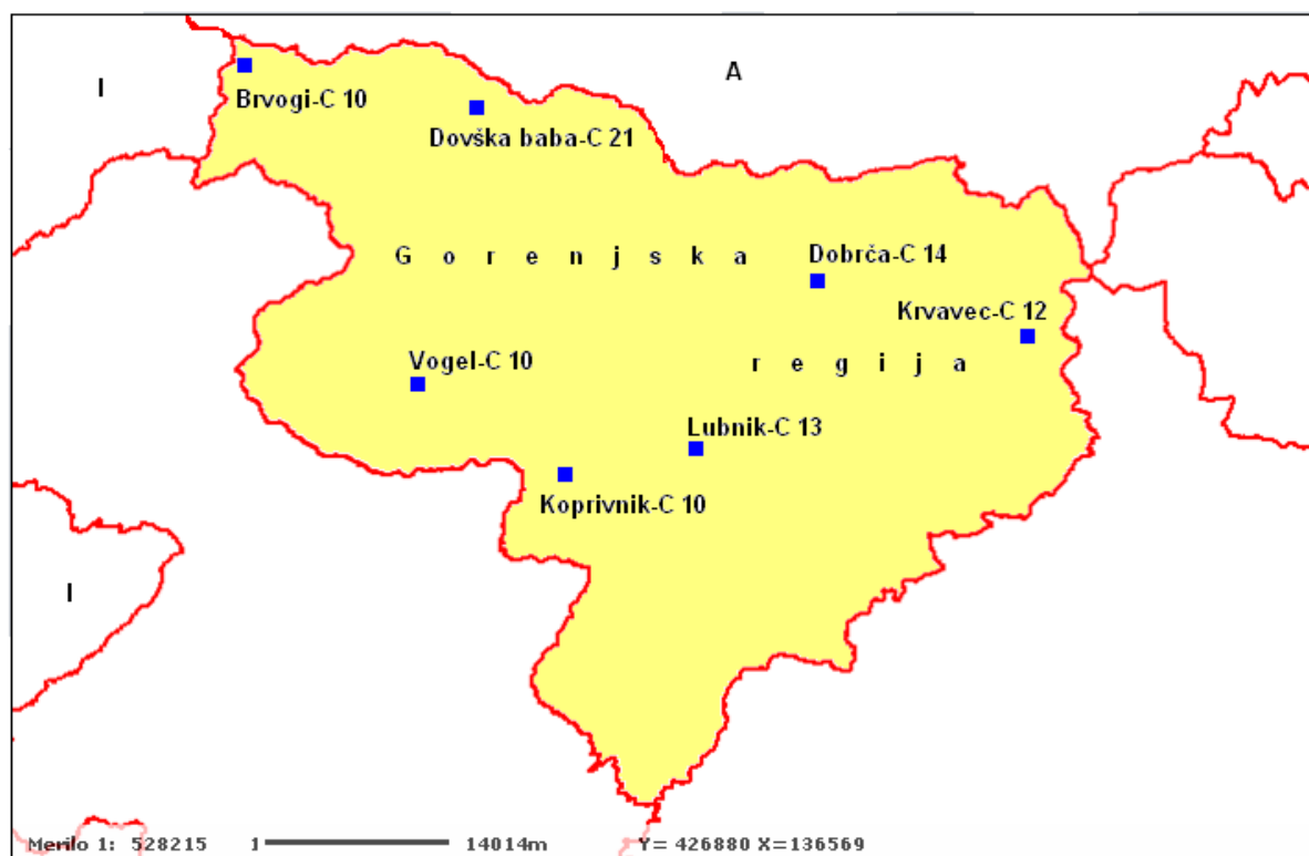
Slika 3: Repetitorske postaje s kanali sistema ZA-RE v Gorenjski regiji
