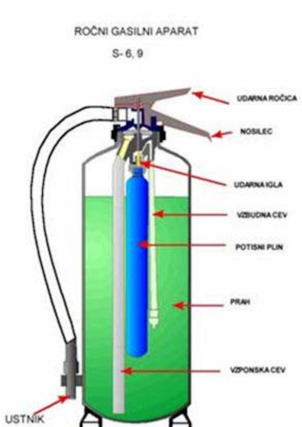
Slika 46: Ročni gasilnik
