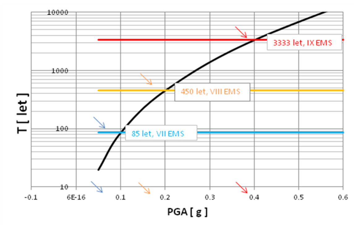
Slika 13: Krivulja potresne nevarnosti za Ljubljano
