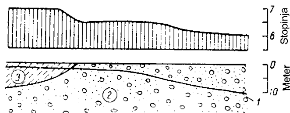
Slika 10: Sprememba stopnje intenzitete v odvisnosti od globine podtalnice v glinasto-peščenih sedimentih (1 – nivo podzemne vode, 2 – peščena glina)
