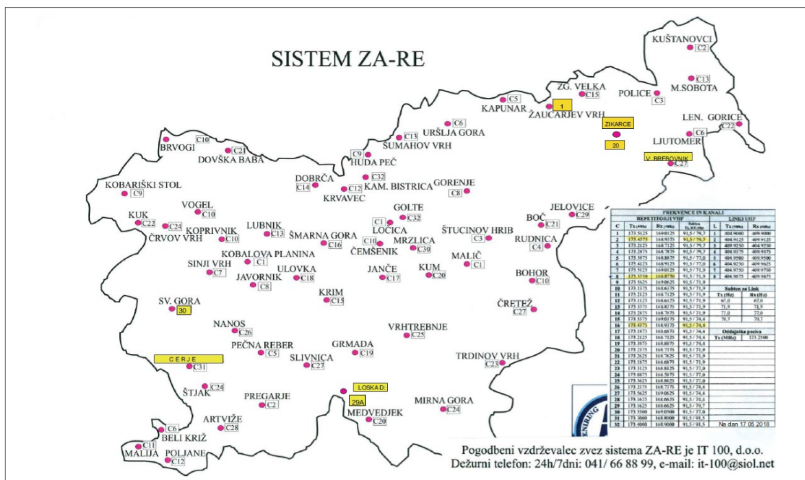
Slika 10: Repetitorske postaje s kanali sistema ZA-RE (URSZR, 2018)
