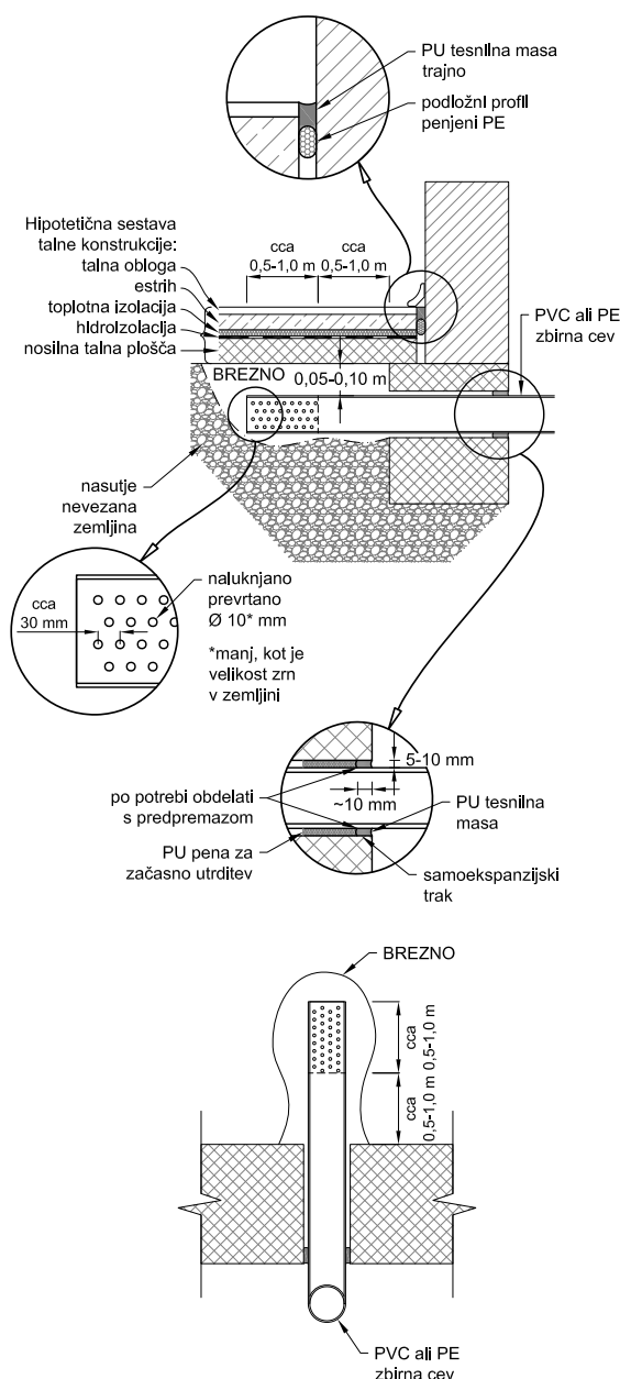
Slika 8: Sesalno brezno od strani – primer
