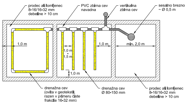
Slika 3: Variante zbirnih cevi za zbiranje radona (zanka, register, brezno)
