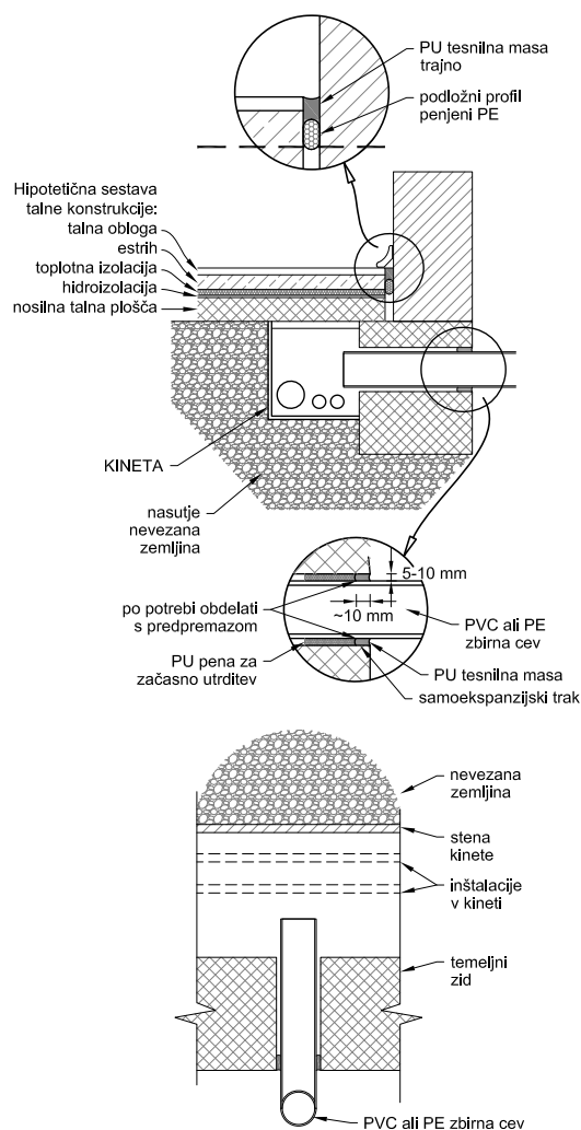
Slika 10: Preboj v kineto kot sesalno brezno – primer
