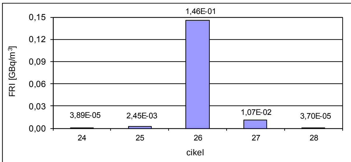
Slika 52: Faktor zanesljivosti goriva (FRI) za zadnjih pet gorivnih ciklov
