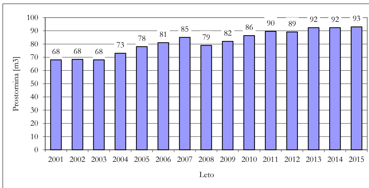
Slika 127: Prostornina paketov radioaktivnih odpadkov v CSRAO ob koncu posameznega leta v letih 2001 - 2015.
