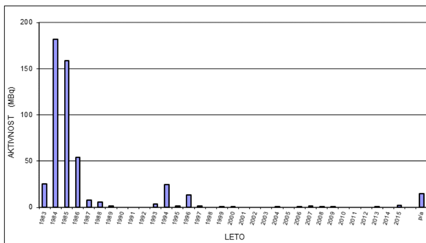
Slika 58: Aktivnost izpuščenega ^{131}\text{I} v tekočinskih izpustih
