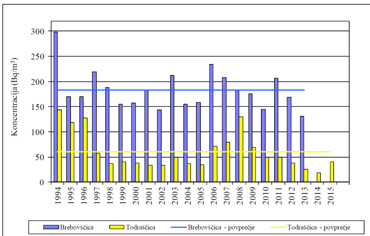
Slika 114: Povprečne letne koncentracije urana ^{238}\text{U} v vodotokih
