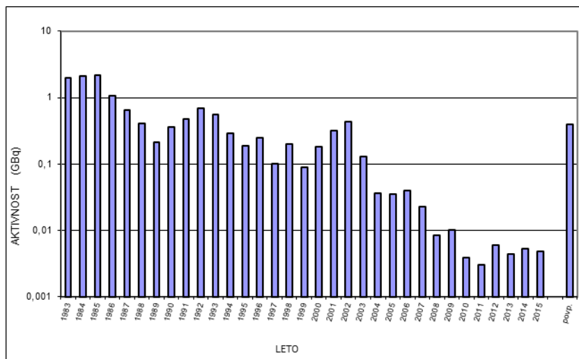
Slika 56: Aktivnost izpuščenega ^{60}\text{Co} v tekočinskih izpustih
