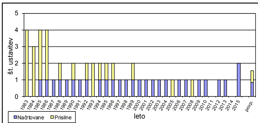
Slika 3: Normalne zaustavitve reaktorja – načrtovane in prisilne
