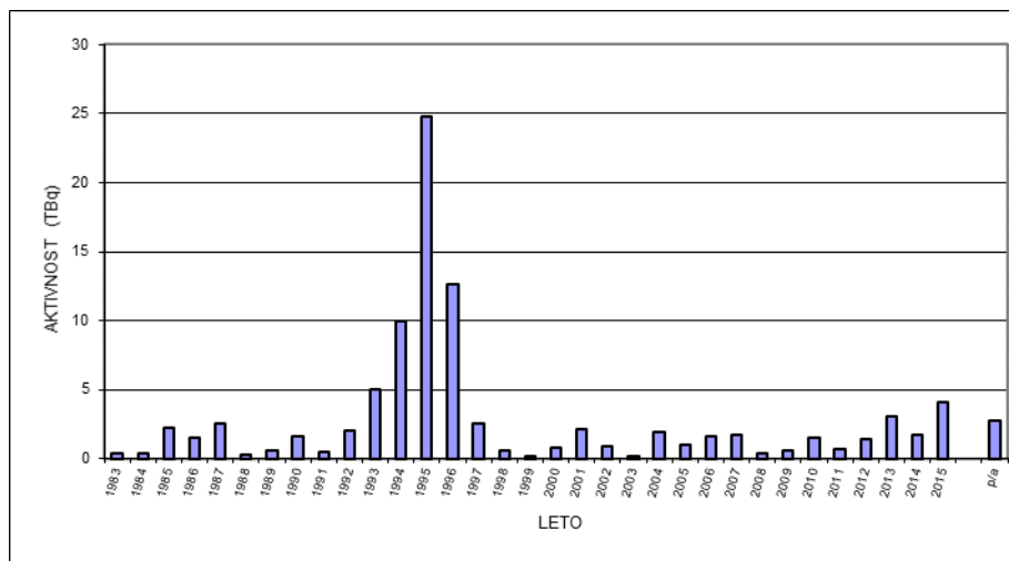
Slika 59: Aktivnost žlahtnih plinov v plinskih emisijah po posameznih letih obratovanja (ekivalent ^{133}\text{Xe} )
