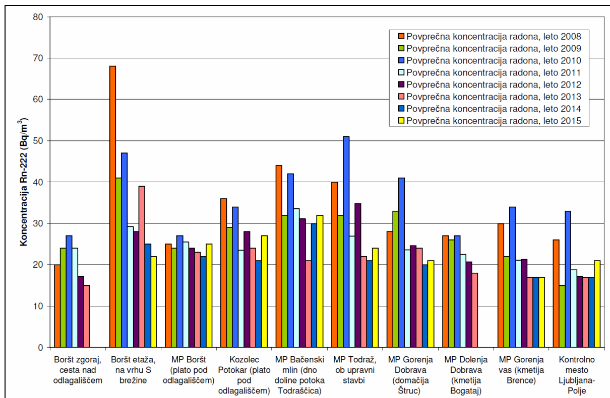
Slika 88: Povprečne letne koncentracije radona v vzdolžnem profilu Merilna postaja Boršt Bačenski mlin – Gorenja vas, izmerjene z detektorji sledi leta 2008-2015
