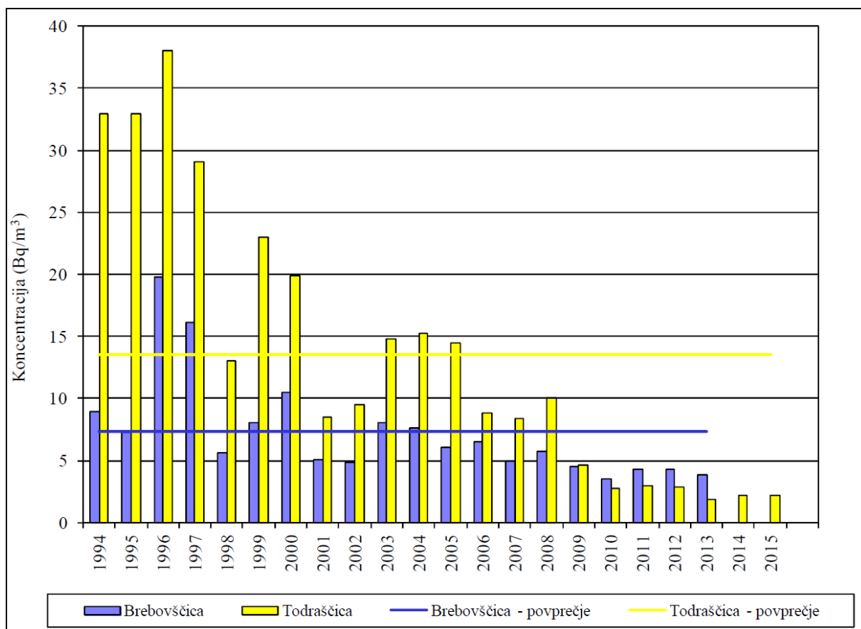
Slika 115: Povprečne letne koncentracije ^{226}\text{Ra} v vodotokih
