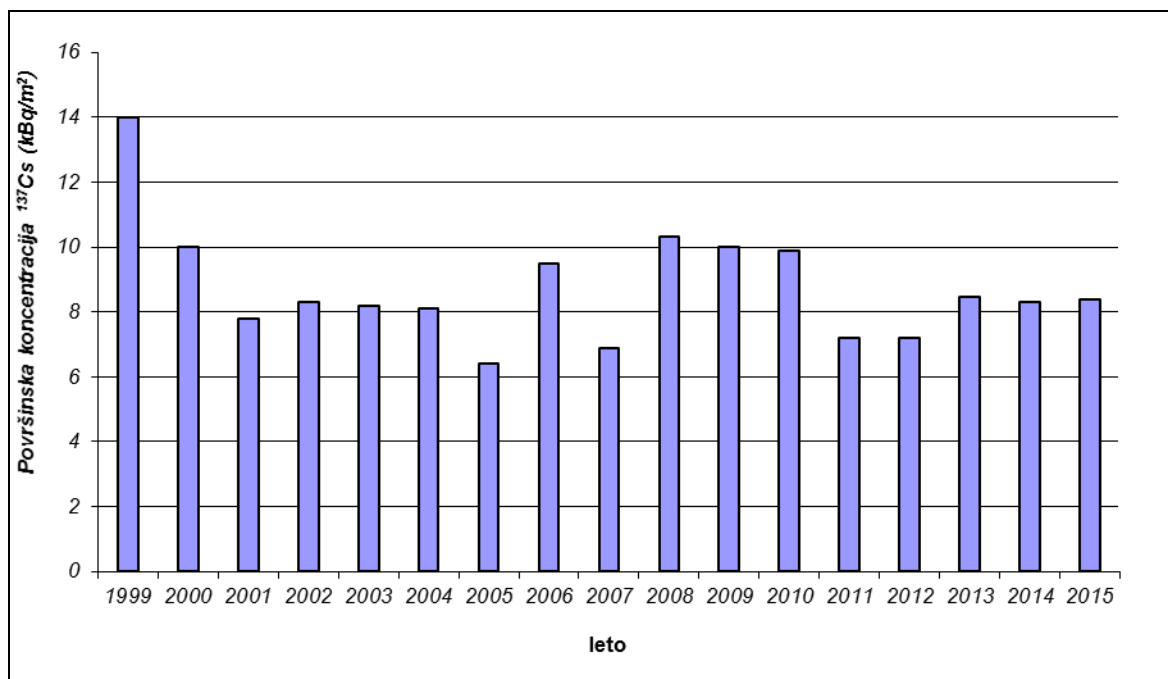
Slika 110: Rezultati kontaminacije tal s ^{137}\text{Cs} v plasti 0–15 cm v Ljubljani
