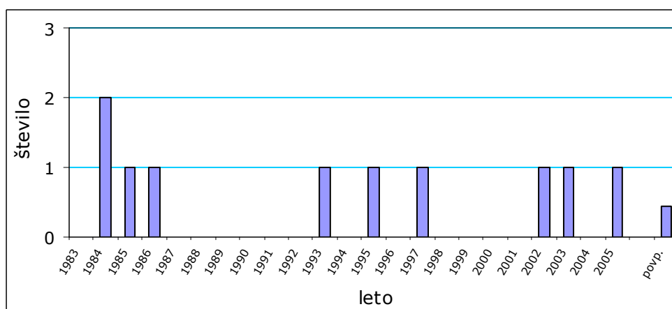
Slika 8: Število nenačrtovanih sprožitvev sistema za varnostno vbrizgavanje
