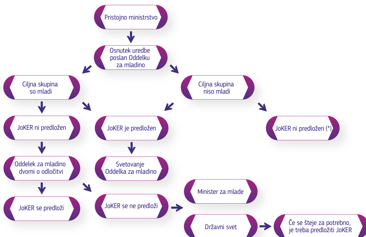
Slika 7: Belgija: JoKER
