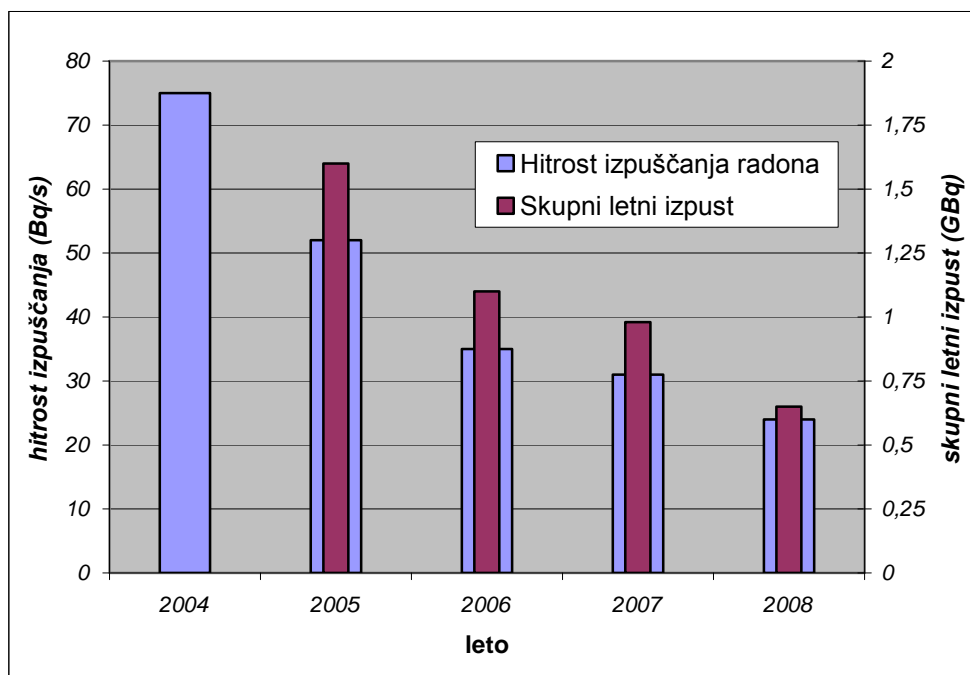
Slika 13: Emisije ^{222}\text{Rn} iz skladišča NSRAO v Brinju
