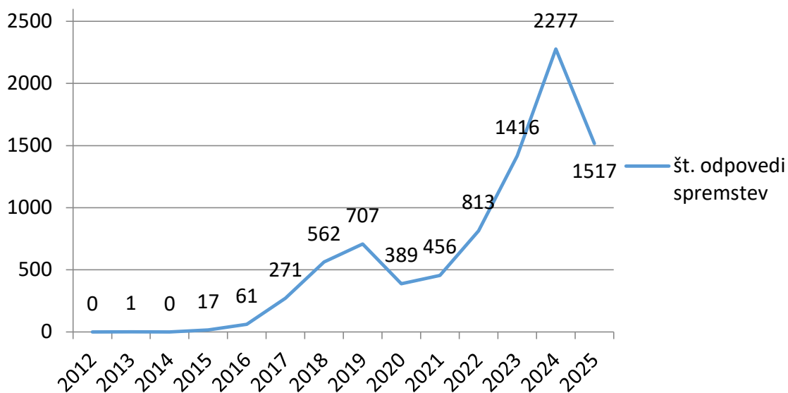
Graf odpovedi spremstev od 2012 do 2025
