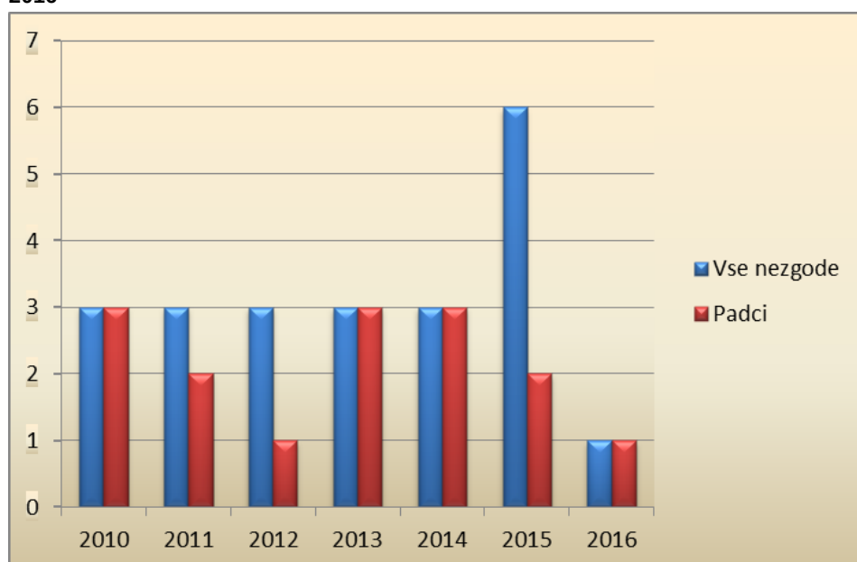
Graf 16: Število vseh smrtnih nezgod na deloviščih in delež smrtnih nezgod zaradi padca v globino, 2010–2016
