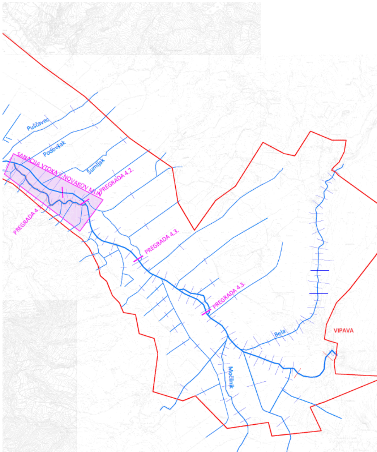
Slika: Območja hidravličnega modeliranja in lokacij prečnih prereзов projekta VIPava.
