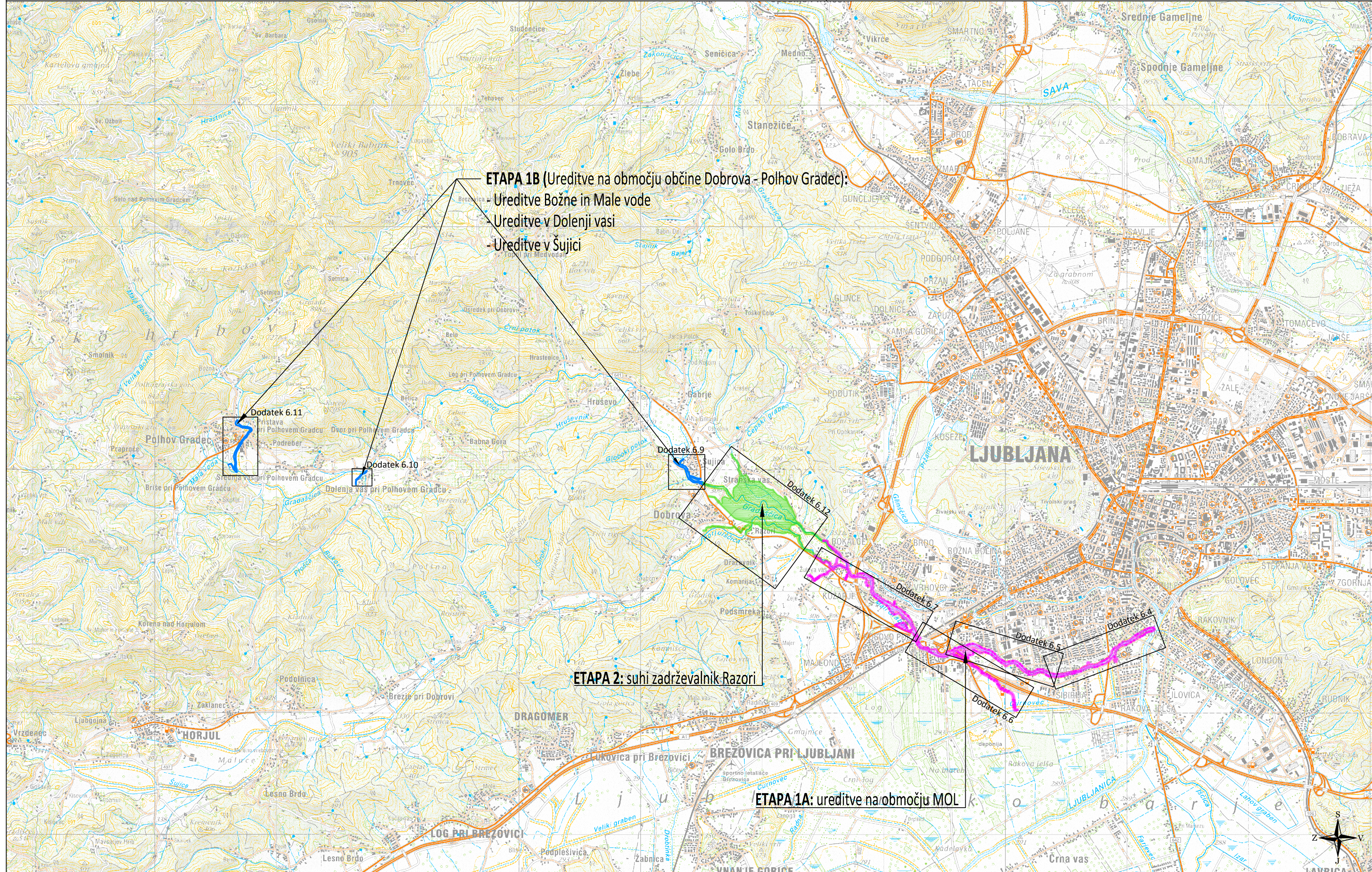
Dodatek 6.3: Protipoplavna ureditev porečja Gradašče Pregledna situacija vseh ureditev M 1:50.000
