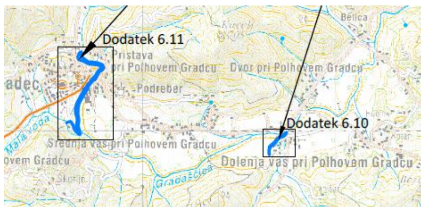
Slika 1: Pregledna situacija vseh ureditev celotnega projekta za zmanjšanje poplavne ogroženosti porečja Gradašče – v skladu z DPN
