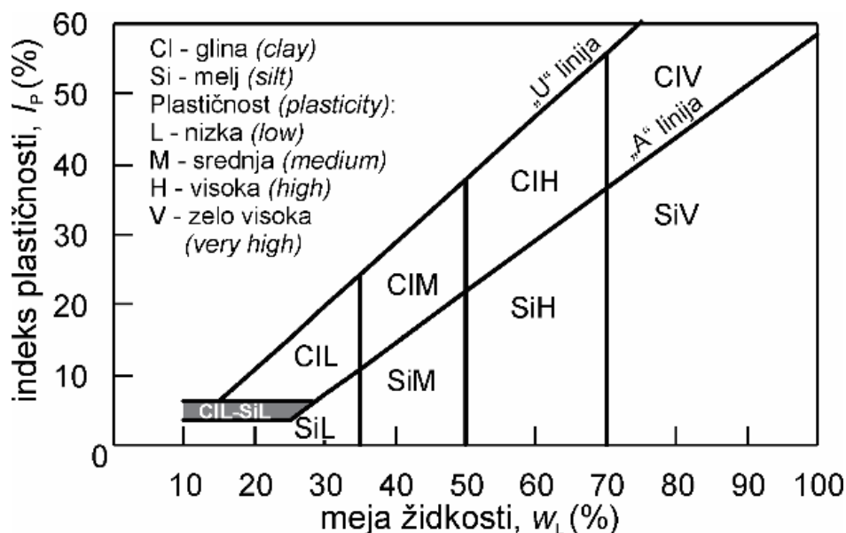
Slika R.3: Diagram plastičnosti (nekoč znan tudi kot AC diagram) z načeli razvrščanja drobnnozrnatih zemljin. Univerzalni diagram, podan tudi v TSPI PG. 05.201, a s spremenjeno terminologijo in simboli za oznake zemljin.
