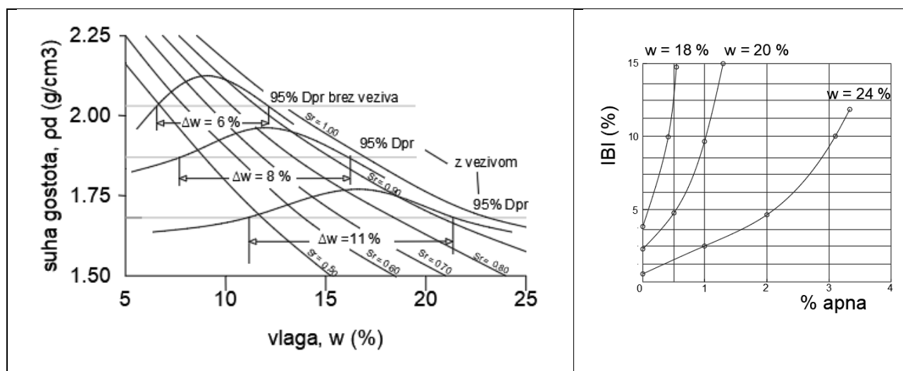
Slika R.4: Razlaga vpliva delovanja apna v glineni zemljini, levo: vpliv dodatka apna na položaj Proctorjeve krivulje v Proctorjevem diagramu in na razpon vgradljivosti ( \Delta w ); desno: informativni prikaz učinka apna na isto zemljino pri različnih vlažnostih.
