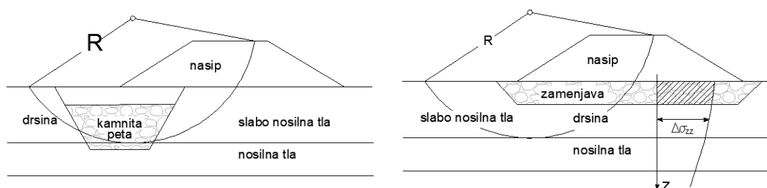
Slika 3.5: Shemi plitve sanacije temeljnih tal z zamenjavo. Levo: delna zamenjava s kamnito peto; desno: delna zamenjava v celotnem tlorisu pod nasipom. Zamenjava desno ni ekvivalent povoznemu platoju. Šrafirana je ploščina diagrama dodatnih napetosti ( \Delta A_{\infty} ), ki vpliva na zmanjšanje posedkov zaradi delne zamenjave materiala po enačbi \Delta p_{\infty} = \Delta A_{\infty} / E_{oed} .
