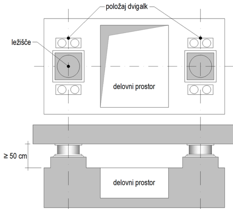
Slika 2.6: Shema delovnega prostora na vrhu stebra z ležiščema na betonskih podstavkih in lokacijami dvigalk. Betonski podstavki omogočajo normalno dostopnost do ležišč ob višini 50 cm in več med spodnjo površino prekladne konstrukcije in ležiščno polico ob pregledu ali zamenjavi ležišč.
