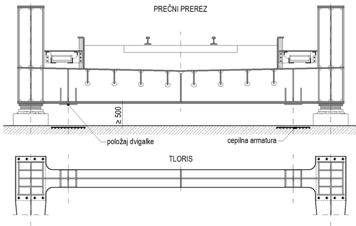
Slika 2.9: Ojačitve prečnika jeklenega ločnega nosilca z vešalkami nad drsnim ležiščem in v področju predvidenih dvigalk.
