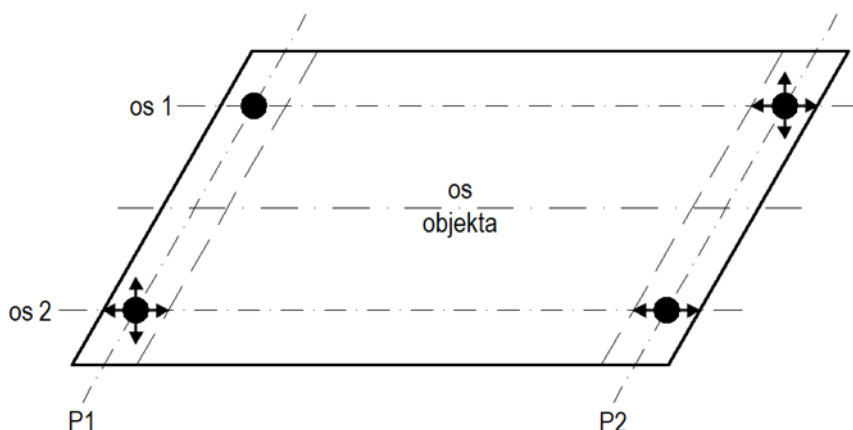
Slika 0.11: Shema podpiranja mostu preko enega polja s poševnimi podporami s točkovno zasučnimi ležišči. Fiksno ležišče v vzdolžni osi 1 na podpori P1 ter vodeno ležišče v vzdolžni osi 2 na podpori P2 na sta postavljeni na lokaciji z največjo tlačno silo
