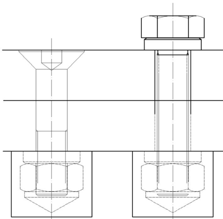
Slika 2.15: Skica vijačnega spoja z zaščitnim pokrovom pri betonski podlagi
