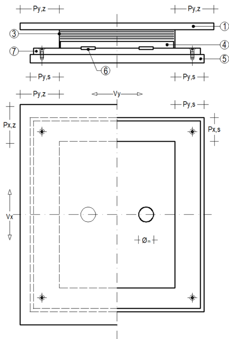
Slika 2.20: Skica vgradnje elastomernega ležišča s spodnjo in zgornjo sidrno ploščo, spodnjo vmesno ploščo privijačeno na sidrno ploščo in zavarovanja proti zdrsu (1 – zgornja sidrna plošča; 3 – ležišče; 4 – spodnja ležiščna plošča; 5 – spodnja sidrna plošča; 6 – mozni; 7 – vmesna plošča).
