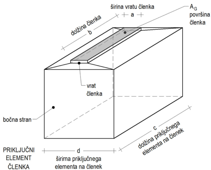
Slika 1.12: 3D skica elementov s poimenovanjem konstruktivnih delov betonskega členka.
