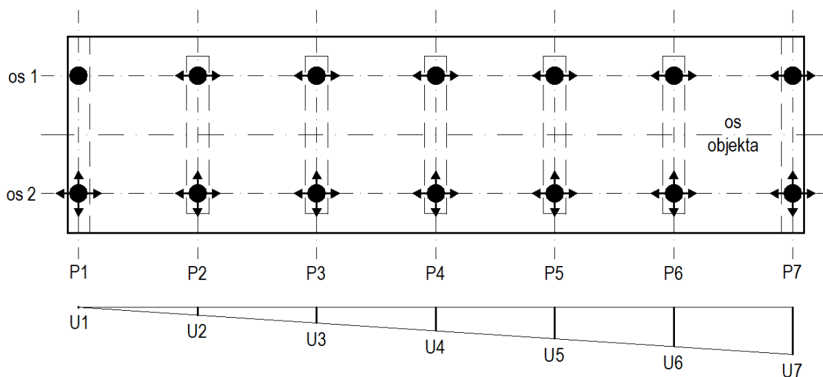
Slika 0.12: Shema podpiranja kontinuirane prekladne konstrukcije s fiksnim ležiščem v osi 1 na krajnem oporniku P1. Lokacija fiksnega ležišča je tudi fiksna točka konstrukcije, iz katere se meri dolžina raztezanja
