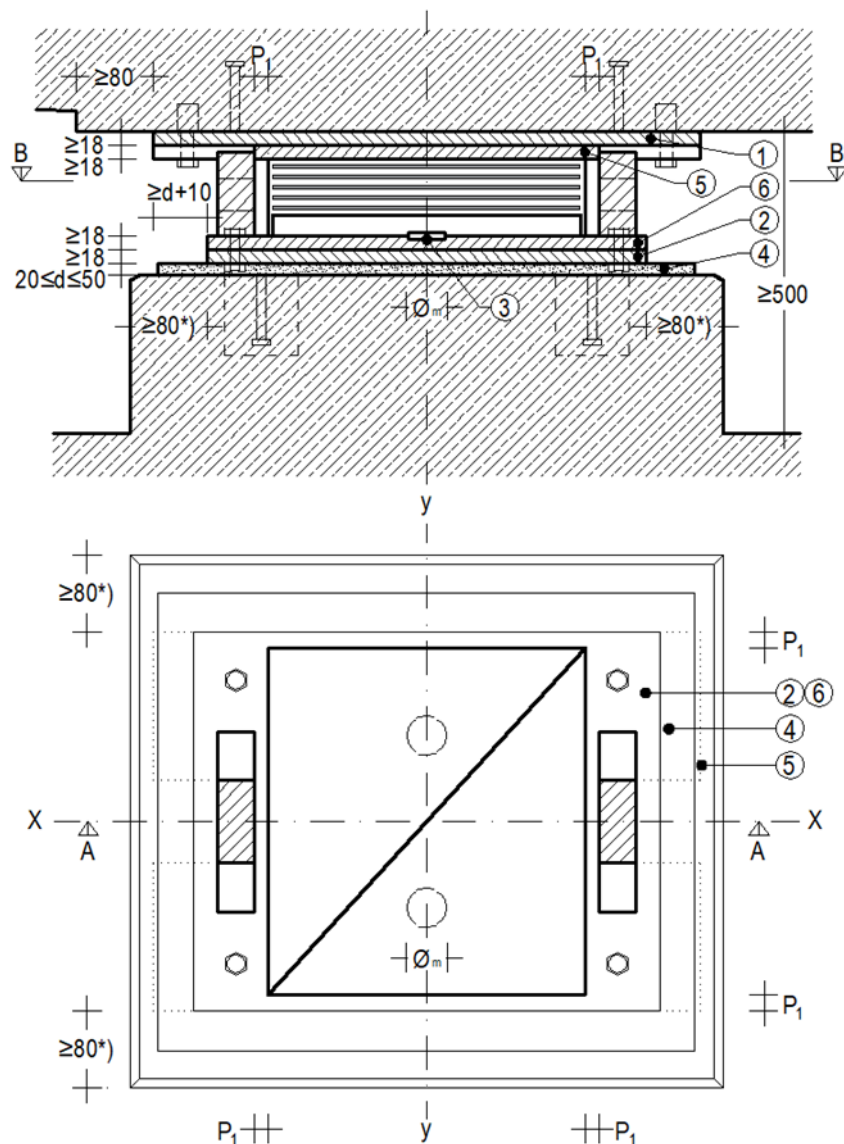
Slika 5.2: Prikaz vgradnje deformabilnega ležišča s pridrževalno konstrukcijo v obeh smereh ( p_1 \geq 25 mm; 1 – zgornja sidrna plošča; 2 – spodnja sidrna plošča; 3 – moznik; 4 – podlivna malta; 5 – zgornja ležiščna plošča; 6 – spodnja ležiščna plošča)
