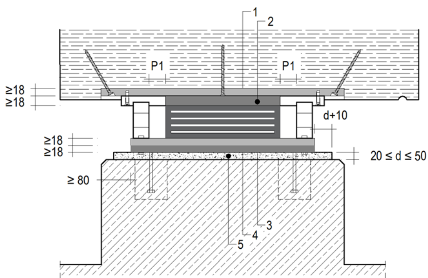
Slika 2.12: Vzдолžni prerez vgradnje in sidranja vzdolžno vodenega elastomernega ležišča tipa C v leseno prekladno konstrukcijo.
