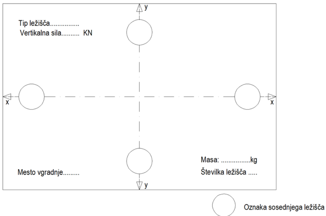
Slika 3.2: Oznake in podatki, ki morajo biti prikazani na zgornji površini fiksnega ležišča
