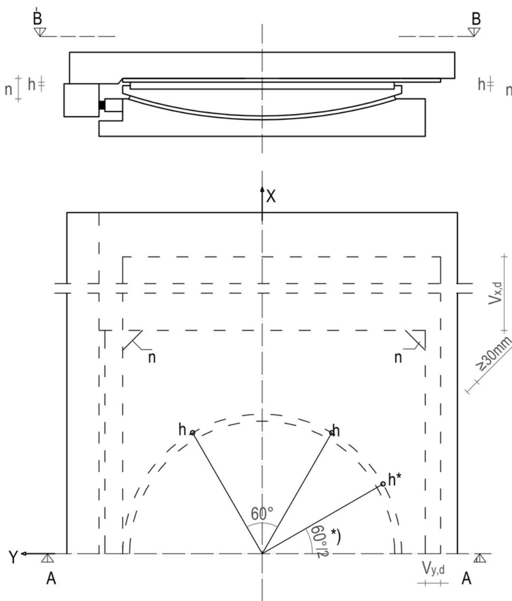
Slika 3.10: Merilne točke drsne špranje h in nagibne špranje n pri sfernem drsnem ležišču v osi glavnih pomikov za bočno vodeno drsno ležišče in vsestransko pomično ležišče
