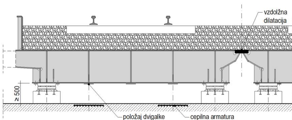
Slika 2.7: Ojačitve prečnika jeklene rešetkaste konstrukcije nad drsnim ležiščem in v področju predvidenih dvigalk.
