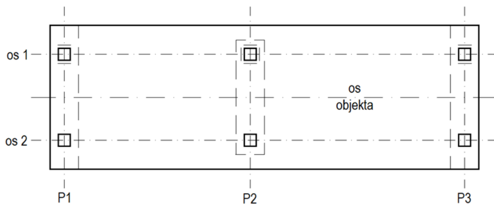
Slika 0.6: Shema elastičnega podpiranja mostu preko dveh polj s fiksnim ležiščem na vmesnem oporniku
