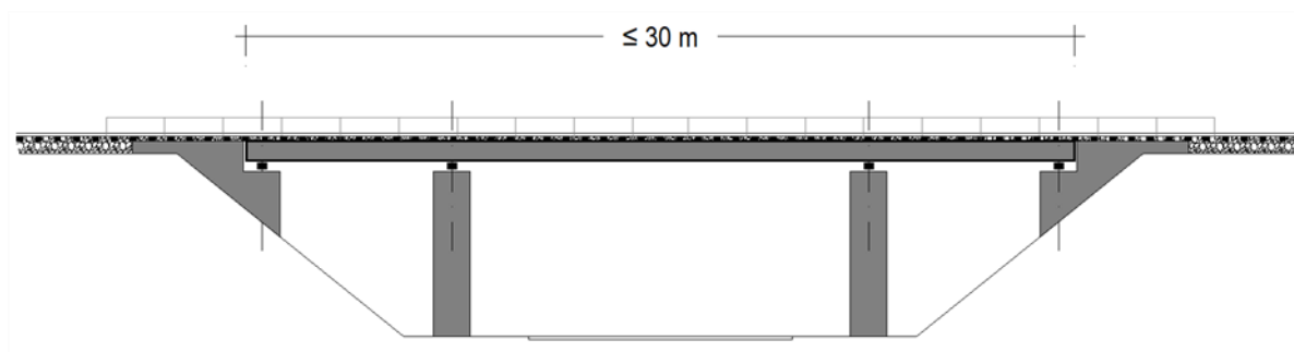
Slika 0.21: Shema elastičnega podpiranja v vzdolžnem prerezu železniškega premostitvenega objekta dolžine do 30 m preko treh polj.
