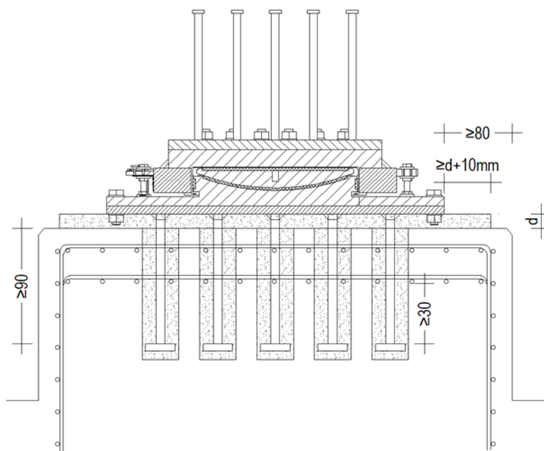
Slika 2.3: Shema sidranja ležišča s sidrno ploščo in čepastimi sidri v betonski podstavek z več slojno cepilno armaturo in podlivno malto.
