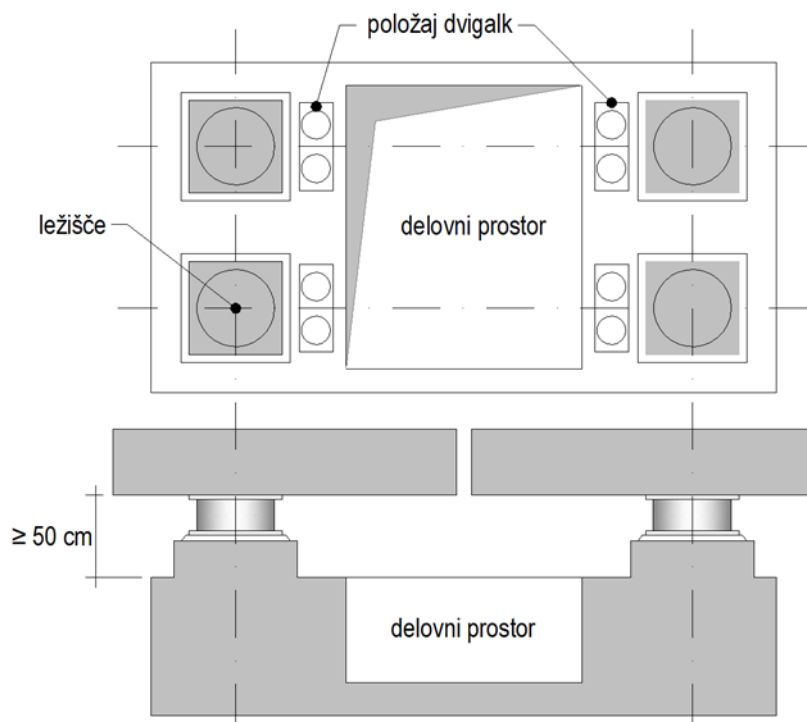
Slika 2.5: Shema delovnega prostora pod dilatirano prekladno konstrukcijo na vrhu stebra z ležišči na betonskih podstavkih ter z lokacijami dvigalk.
