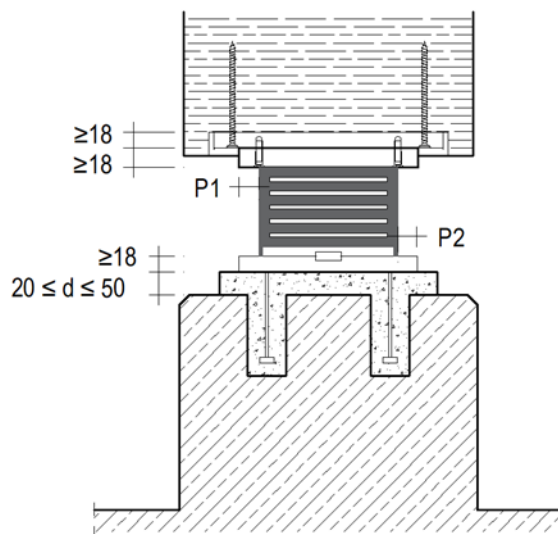
Slika 2.11: Prečni prerez vgradnje in sidranja elastomernega ležišča tipa B/C v leseno prekladno konstrukcijo.
