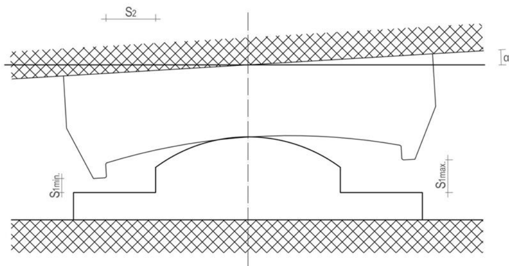
Slika 8.5: Meritve nagibnih špranj jeklenega točkovnega nagibnega ležišča.
