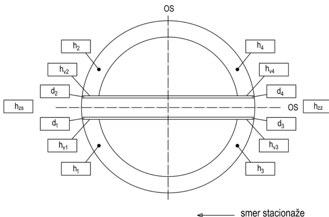
Slika 4.3: Prikaz meritev drsnih špranj h_1 do h_4 in h_{v1} do h_{v4} ob vodilu drsnega dela lončnega ležišča, bočne špranje d_1 do d_4 med vodilom in drsno ploščo ter vertikalni razmik med zgornjo površino vodila in drsne plošče h_{zs} in h_{zz} , ki so podane na notranjem kontrolnem listu
