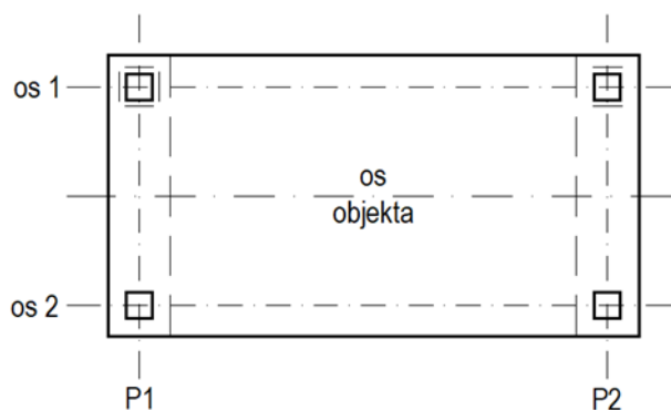
Slika 0.3: Shema elastičnega podpiranja mostu preko enega polja s fiksno točko v osi 1 na krajnem oporniku P1 na lokaciji fiksnega ležišča.
