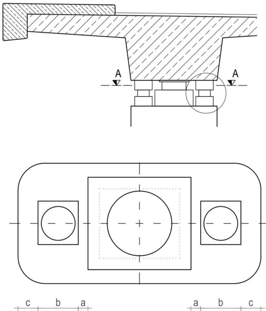
Slika 2.10: Shematični prikaz dvigalk ob ležišču s podložnimi ploščami in minimalnimi razmiki od robov betonske podporne konstrukcije.
