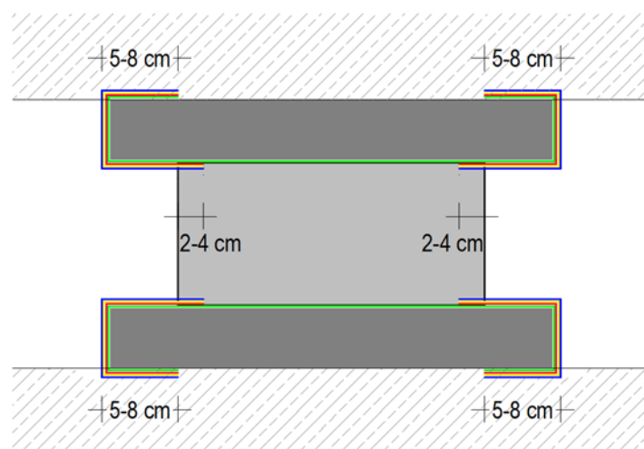
Slika 3.12: Izvedba protikorozijske zaščite ležiščnih plošč deformabilnega ležišča
