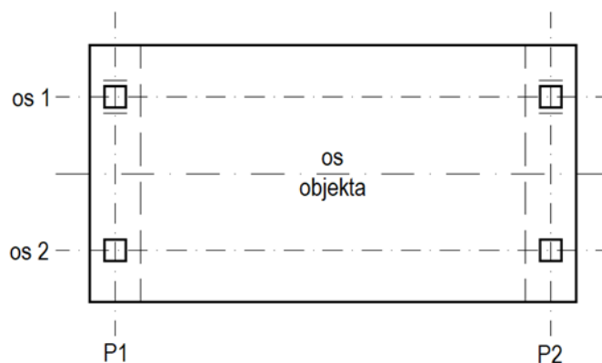
Slika 0.4: Shema elastičnega podpiranja mostu preko enega polja s fiksno točko v sredini razpetine mostu in preprečenimi pomiki v prečni smeri na obeh krajnih opornikih vzdolž ene vzdolžne osi podpiranja.
