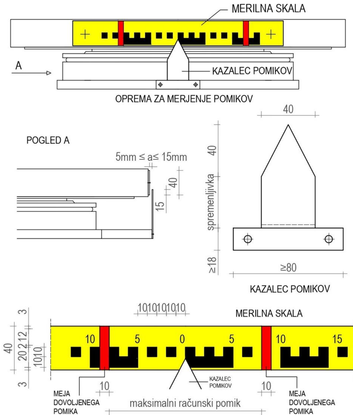
Slika 3.1: Primer merilne skale in kazalca pomikov za spremljanje položaja ležišča
