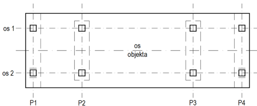
Slika 0.7: Shema elastičnega podpiranja kratkega mostu preko treh polj s preprečenimi pomiki v prečni smeri na obeh krajnih opornikih vzdolž ene vzdolžne osi podpiranja
