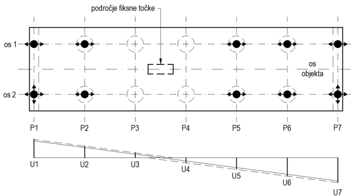
Slika 0.14: Shema podpiranja kontinuirane prekladne konstrukcije z vpetimi stebri v prekladno konstrukcijo v oseh P3 in P4. Lokacija fiksne točke konstrukcije, iz katere se meri dolžina raztezanja, je spremenljiva
