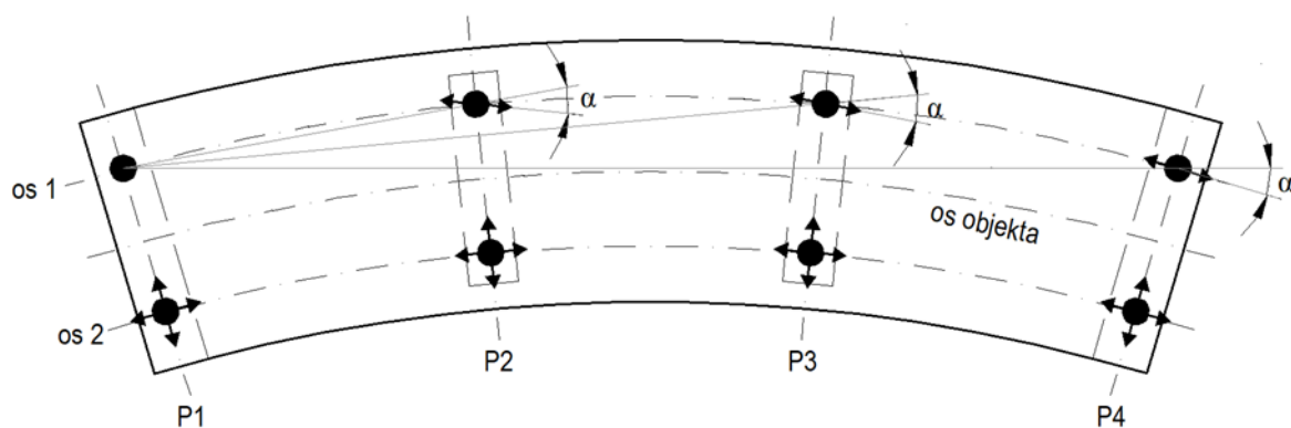
Slika 0.16: Shema polarnega podpiranja kontinuirane prekladne konstrukcije v krivini z vodenimi ležišči usmerjenimi pod enakim kotom glede na polarno smer. Kot je enak kotu med vzdolžno osjo in polarno smerjo na krajnem oporniku s pomičnimi ležišči.
