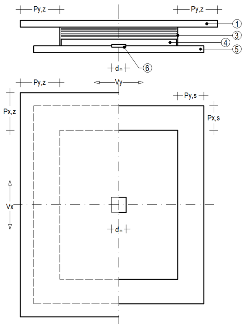
Slika 2.21: Skica vgradnje elastomernega ležišča s spodnjo in zgornjo sidrno ploščo, spodnja ležiščna plošča s sidrno ploščo povezana z moznikom (1 – zgornja sidrna plošča; 3 – ležišče; 4 – spodnja ležiščna plošča; 5 – spodnja sidrna plošča; 6 – moznik).
