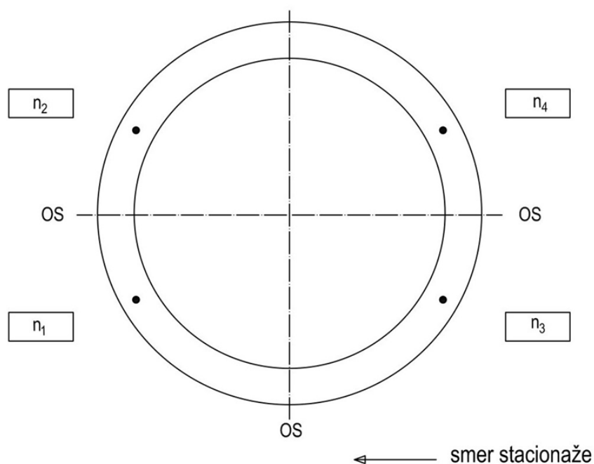
Slika 4.2: Prikaz meritev nagibnih špranj n_1 do n_4 lončnega ležišča, ki so podane na notranjem kontrolnem listu
