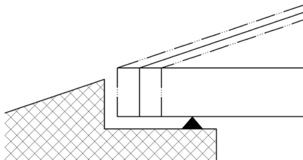
Slika 0.32: Shema pomikov objekta v vzdolžnem padcu pri horizontalni vgradnji ležišča. V tem primeru pri vzdolžnem pomiku ležišča nastane vzdolž dilatacije stopničasti zamik, ki je odvisen od velikosti horizontalnega premika in zasuka prekladne konstrukcije.
