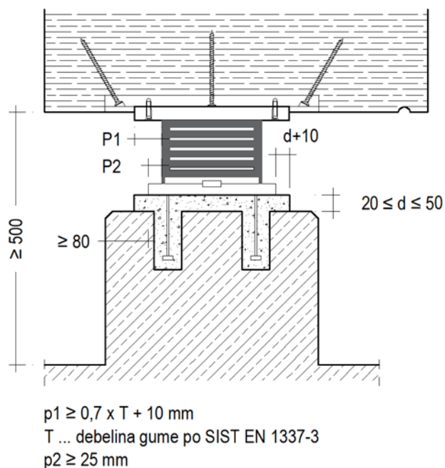
Slika 2.10: Vzдолžni prerez vgradnje in sidranja elastomernega ležišča tipa B/C v leseno prekladno konstrukcijo.
