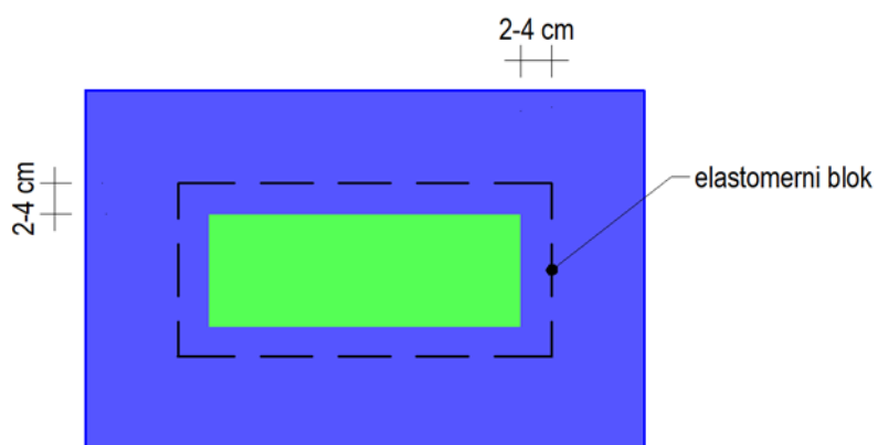
Slika 3.14: Izvedba protikorozijske zaščite kontaktne površine ležiščne plošče z elastomernim blokom
