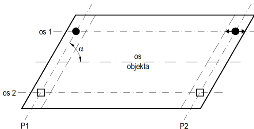
Slika 0.10: Shema elastičnega podpiranja mostu preko enega polja s poševnimi podporami s fiksno točko v osi 1 na krajnem oporniku P1 na lokaciji fiksnega ležišča. Fiksno ležišče je postavljeno na lokaciji z največjo tlačno silo. Ležišča v osi 1 so jeklena točkovna zasučna ležišča z jeklenim ohišjem in okroglim elastomernim ležiščem enake togosti kot okrogla ležišča v osi 2
