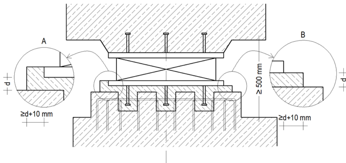
Slika 2.4: Shema podlitja spodnje sidrne plošče.
