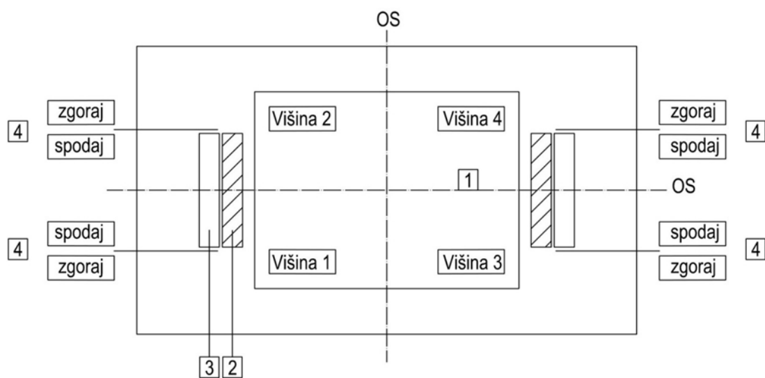
Slika 4.10: Prikaz meritev deformabilnega ležišča s preprečenimi pomiki v prečni smeri na notranjem kontrolnem listu
