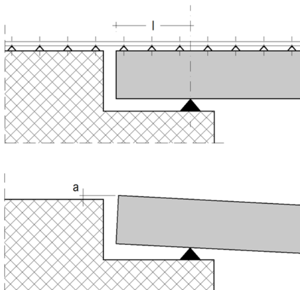
Slika 0.31: Shema položaja osi podpiranja ob dilataciji premostitvenega objekta z neprekinjenimi tirnicami. Razdalja med osjo podpiranja in robom prekladne konstrukcije l je velika, zato so pri zasuku vertikalni zamiki vzdolž dilatacije veliki in posledično lahko nastopijo velike obremenitve v tirnicah in pritrditvenimi elementi tirnice na pragove togega tira.
