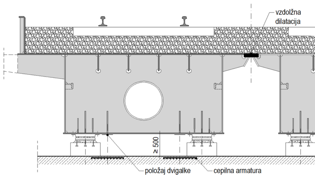
Slika 2.13: Ojačitve prečnika jeklene škatlaste konstrukcije nad drsnim ležiščem in v področju predvidenih dvigalk.
