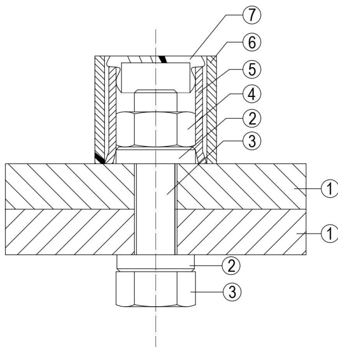
Slika 2.1: Primer izvedbe povezave sidrne in ležiščne plošče na betonsko konstrukcijo s prednapetimi vijaki. (Legenda: 1 – ležiščna oziroma sidrna plošča; 2 – podložka; 3 – vijak s šest robno glavo; 4 – šest robna matica; 5 – tulec iz jeklene pločevine; 6 – prožno 2 mm rebrasto pokrivalo; 7 – pokrivni čep)
