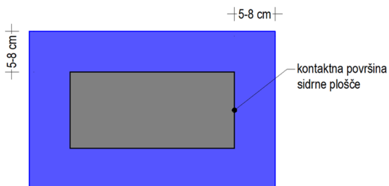
Slika 3.13: Izvedba protikorozijske zaščite kontaktne površine ležiščne plošče z betonom
