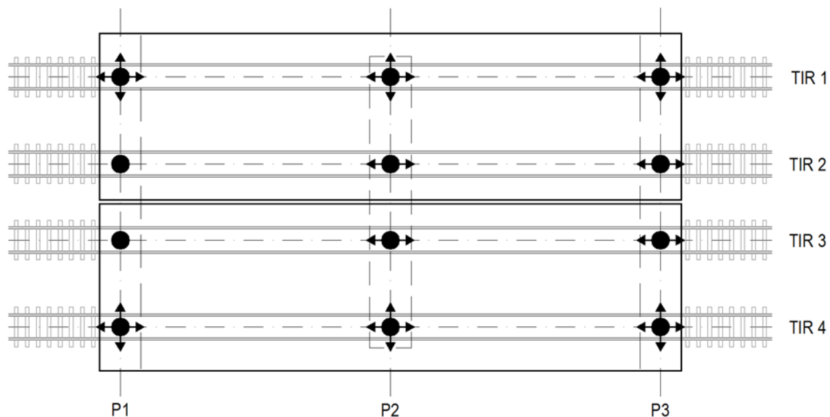
Slika 0.24: Shema podpiranja železniškega premostitvenega objekta z vzdolžno dilatacijo
