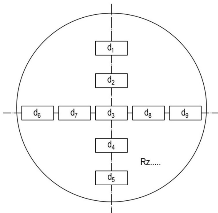
Slika 4.5: Prikaz meritev nanosa trde kromirane plasti na kaloti na notranjem kontrolnem listu
