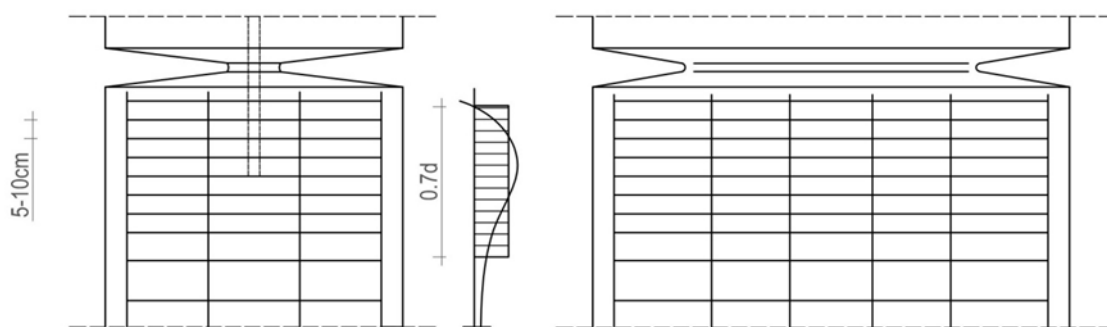
Slika 1.14: Skica armiranja priključnih elementov v prerezu betonskega členka.
