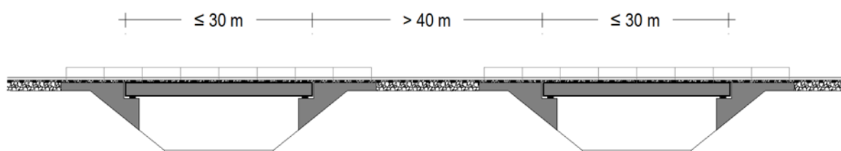
Slika 0.22: Shema elastičnega podpiranja v vzdolžnem prerezu železniškega premostitvenega objekta dolžine do 30 m.
