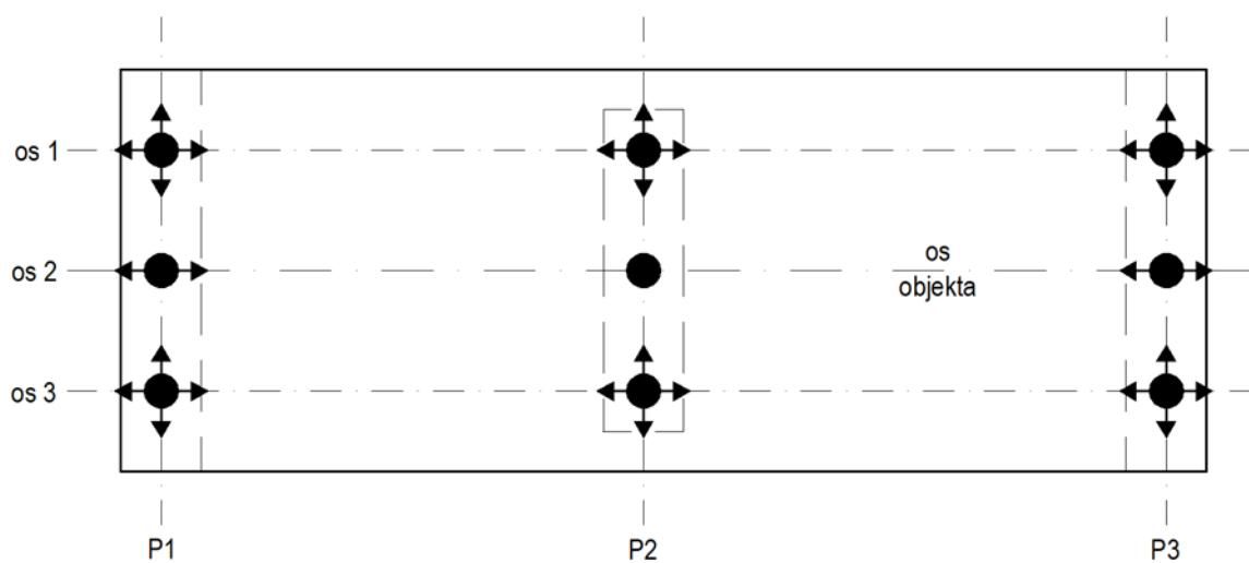
Slika 0.29: Shema podpiranja železniškega premostitvenega objekta s tirom na togi podlagi za omejitev prečnih pomikov vzdolž zunanjih robov.
