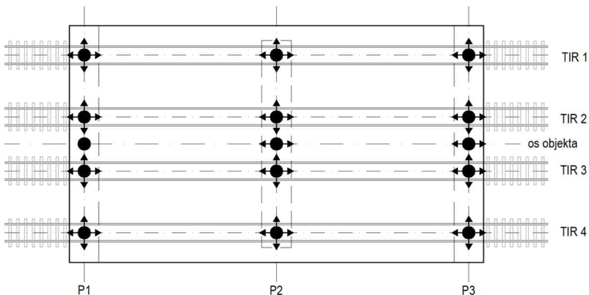
Slika 0.23: Shema podpiranja železniškega premostitvenega objekta z več kot dvema tiroma
