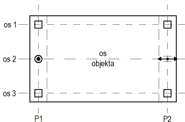
Slika 0.5: Shema elastičnega podpiranja mostu preko enega polja z uporabo vodenega in pridrževalnega ležišča s fiksno točko v vzdolžni osi 2 na krajnem oporniku P1 na lokaciji pridrževalnega ležišča.
