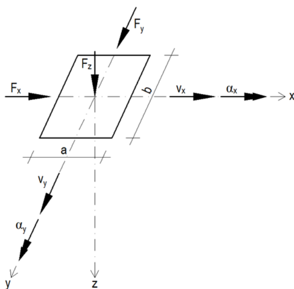
Slika 1.1: Koordinatni sistem za podajanje sil, pomikov in zasukov na primeru elastomernega ležišča.
