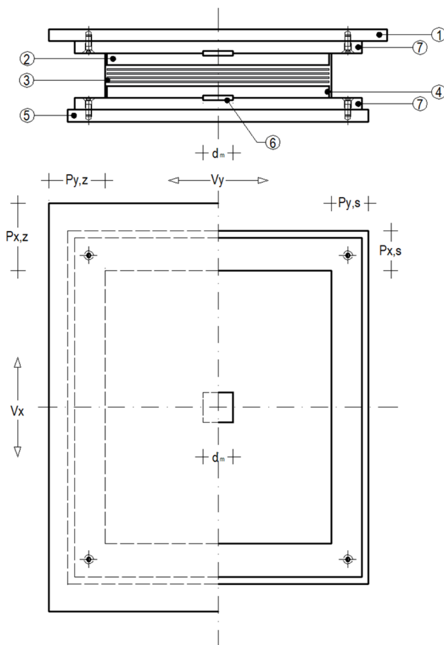
Slika 2.22: Skica vgradnje elastomernega ležišča s spodnjo in zgornjo sidrno ploščo, vmesno ploščo privijačeno na sidrno ploščo in zavarovanja proti zdrsu (1 – zgornja sidrna plošča; 2 – zgornja ležiščna plošča; 3 – ležišče; 4 – spodnja ležiščna plošča; 5 – spodnja sidrna plošča; 6 – mozni; 7 – vmesna plošča; a – debelina zvara).
