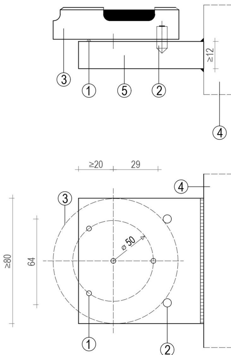
Slika 3.5: Referenčna horizontalna ravnina (1 – navojni zatič; 2- pozicijski zatič; 3 – dvoosna libela, merilno območje 3‰ razdeljeno s petimi črticami; 4 – spodnji del ležišča (ležišča oziroma sidrna plošča; 5 konzolna ravnina za tritočkovno libelo; dimenzije na sliki so podane v mm).
