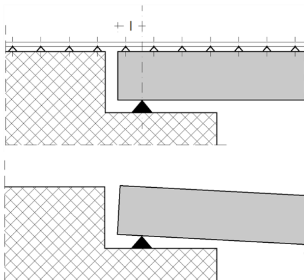
Slika 0.30: Shema položaja osi podpiranja ob dilataciji premostitvenega objekta z neprekinjenimi tirnicami. Razdalja med osjo podpiranja in robom prekladne konstrukcije l je majhna, zato so pri zasuku vertikalni zamiki vzdolž dilatacije lahko majhni in posledično nastopajo majhne obremenitve v tirnicah.
