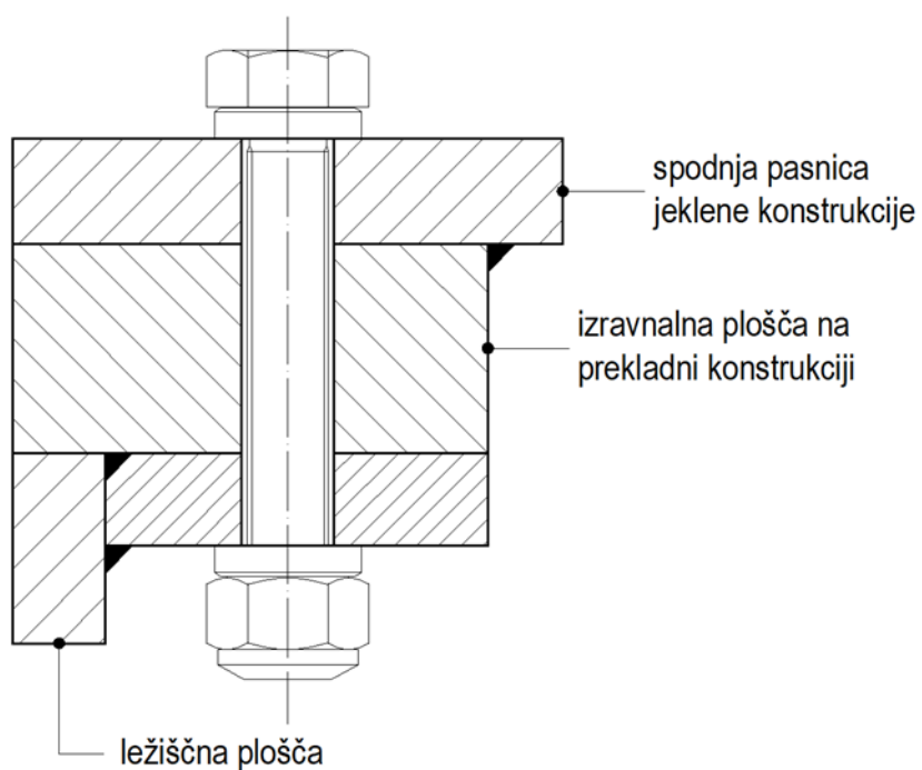
Slika 2.16: Skica vijačnega spoja ležišča z jekleno konstrukcijo
