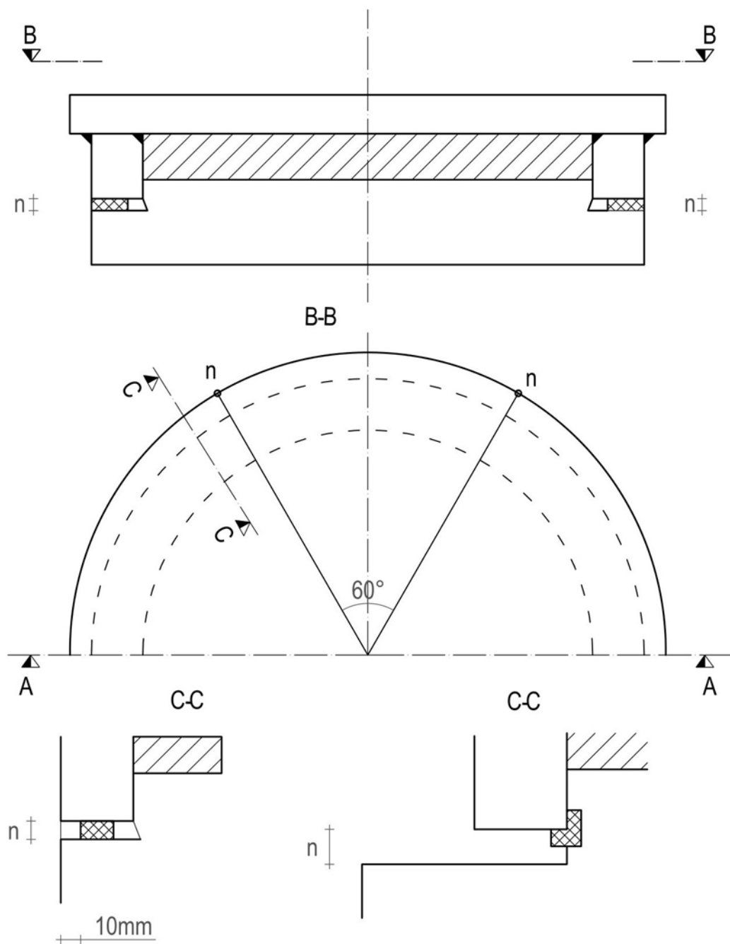
Slika 3.8: Merilne točke nagibne špranje n pri lončnem fiksnem ležišču v vzdolžni osi ležišča.
