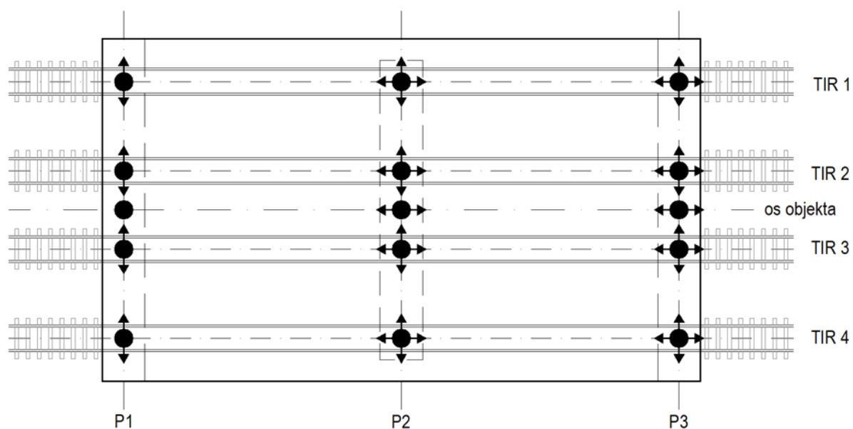
Slika 0.25: Shema podpiranja železniškega premostitvenega objekta z več kot dvema tiroma s prevzemom horizontalnih sil na krajnem oporniku s fiksnim in prečno vodenimi ležišči
