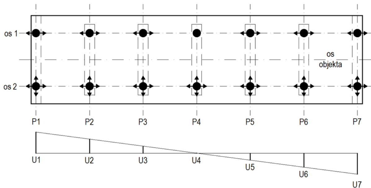
Slika 0.13: Shema podpiranja kontinuirane prekladne konstrukcije s fiksnim ležiščem v osi 1 na vmesnem oporniku v osi P4, ki je tako tudi lokacija fiksne točke konstrukcije, iz katere se meri dolžina raztezanja
