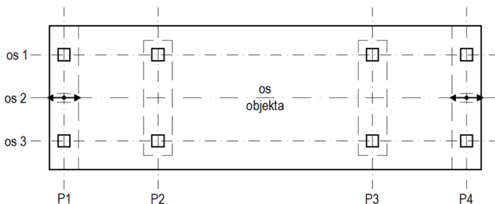
Slika 0.8: Shema elastičnega podpiranja kratkega mostu preko treh polj z vodenima ležiščema v osi objekta na obeh krajnih opornikih
