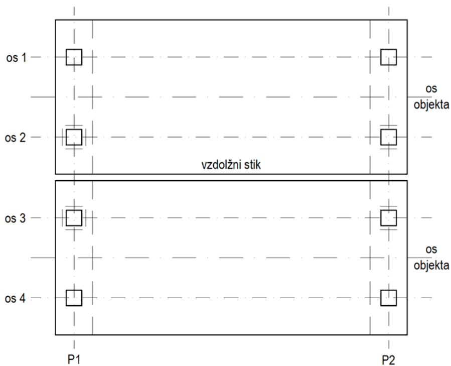
Slika 0.28: Shema elastičnega podpiranja železniškega premostitvenega objekta z vzdolžno dilatacijo.
