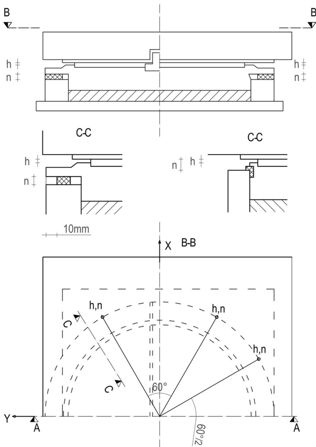
Slika 3.7: Merilne točke drsne špranje h in nagibne špranje n pri lončnem drsnem ležišču v osi glavnih pomikov za vodeno drsno ležišče in vsestransko pomično ležišče
