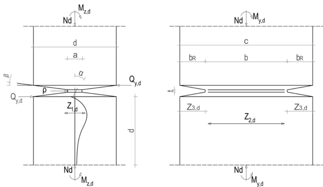
Slika 1.13: Skica obremenitev, področja armiranja ter geometrijski podatki betonskega členka.
