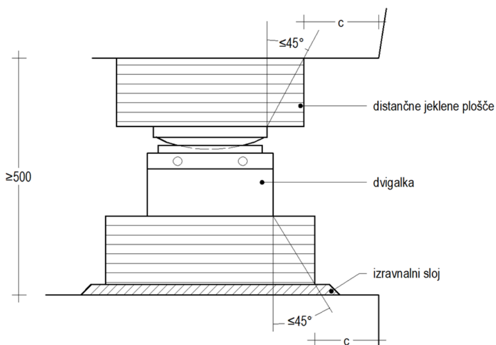
Slika 2.9: Shema dvigalka s podložnimi ploščami in minimalnim odmikom od prostih robov betonske prekladne in podporne konstrukcije.
