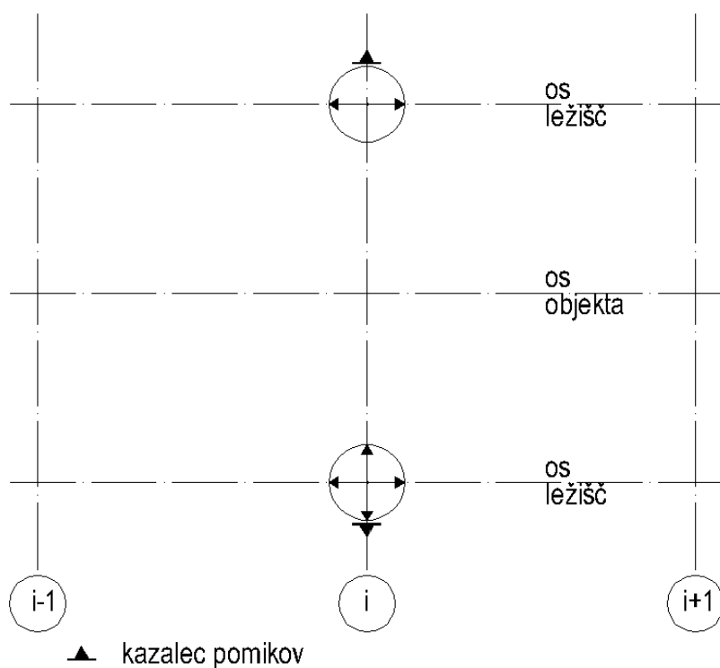
Slika 1.6: Možna situacija kazalca pomikov in mersko skalo, če je dostop za pregled ležišč omogočen z lestvijo ali dvizžno ploščadjo.
