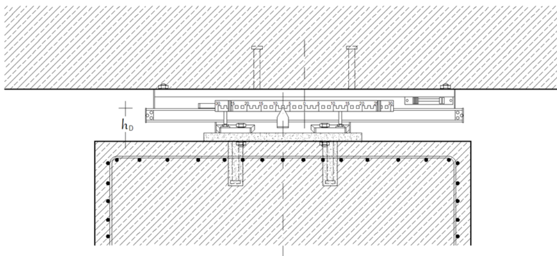
Slika 2.7: Shema delovnega prostora na vrhu stebra z ležiščema na betonskih podstavkih in lokacijami dvigalk. Betonski podstavki omogočajo normalno dostopnost do ležišč ob višini 50 cm in več med spodnjo površino prekladne konstrukcije in ležiščno polico ob pregledu ali zamenjavi ležišč.
