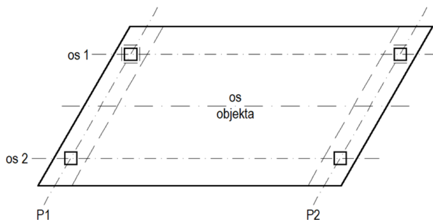
Slika 0.9: Shema elastičnega podpiranja mostu preko enega polja s poševnimi podporami s fiksno točko v osi 1 na krajnem oporniku P1 na lokaciji fiksnega ležišča. Fiksno ležišče je postavljeno na lokaciji z največjo tlačno silo
