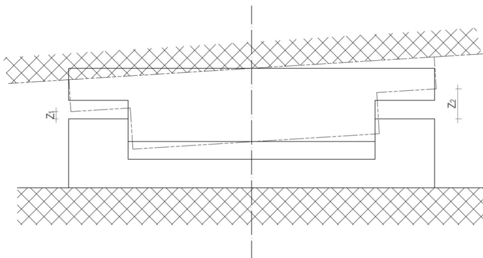
Slika 8.3: Meritve nagibnih špranj lončnega ležišča.
