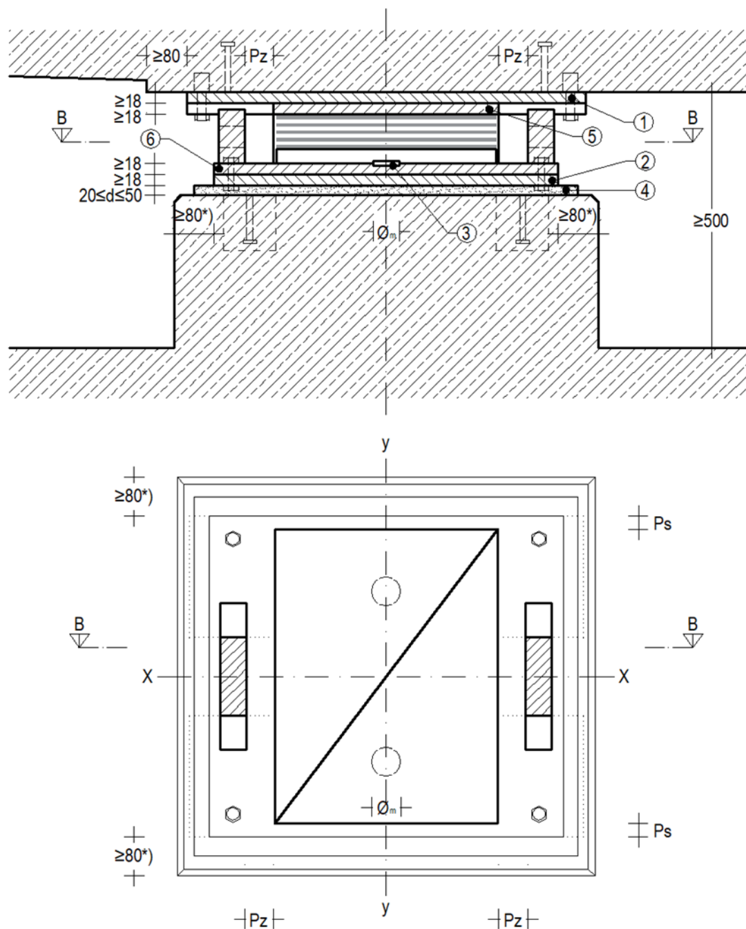
Slika 5.3: Prikaz vgradnje deformabilnega ležišča s pridrževalno konstrukcijo v prečni smeri ( p_s \geq 25 mm; p_z \geq 0,7 \times T_q + 10 mm); 1 – zgornja sidrna plošča; 2 – spodnja sidrna plošča; 3 – moznik; 4 – podlivna malta; 5 – zgornja ležiščna plošča; 6 – spodnja ležiščna plošča)
