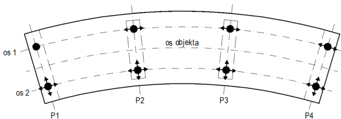
Slika 0.17: Shema tangencialnega podpiranja kontinuirane prekladne konstrukcije v krivini.
