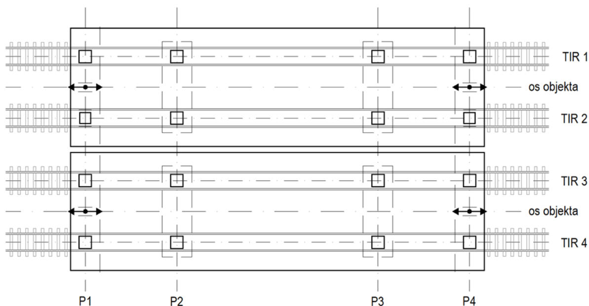
Slika 0.27: Shema elastičnega podpiranja v kombinaciji z vodenima ležiščema železniškega premostitvenega objekta z vzdolžno dilatacijo pri objektih dolžine do 30 m.
