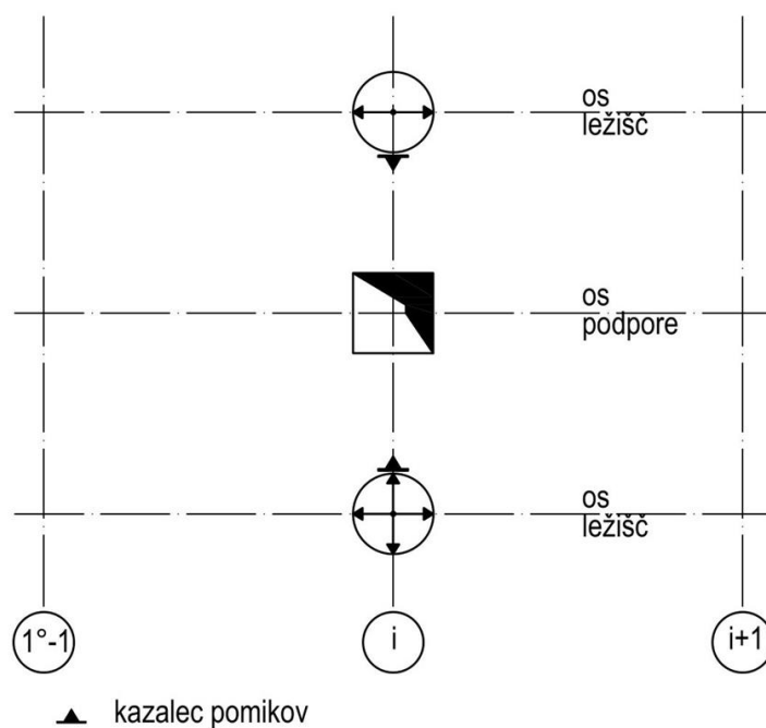
Slika 1.2: Situacija kazalca pomikov in mersko skalo, če je dostop za pregled ležišč omogočen preko škatle prekladne konstrukcije ali pa preko dostopa na vrhu stebra.
