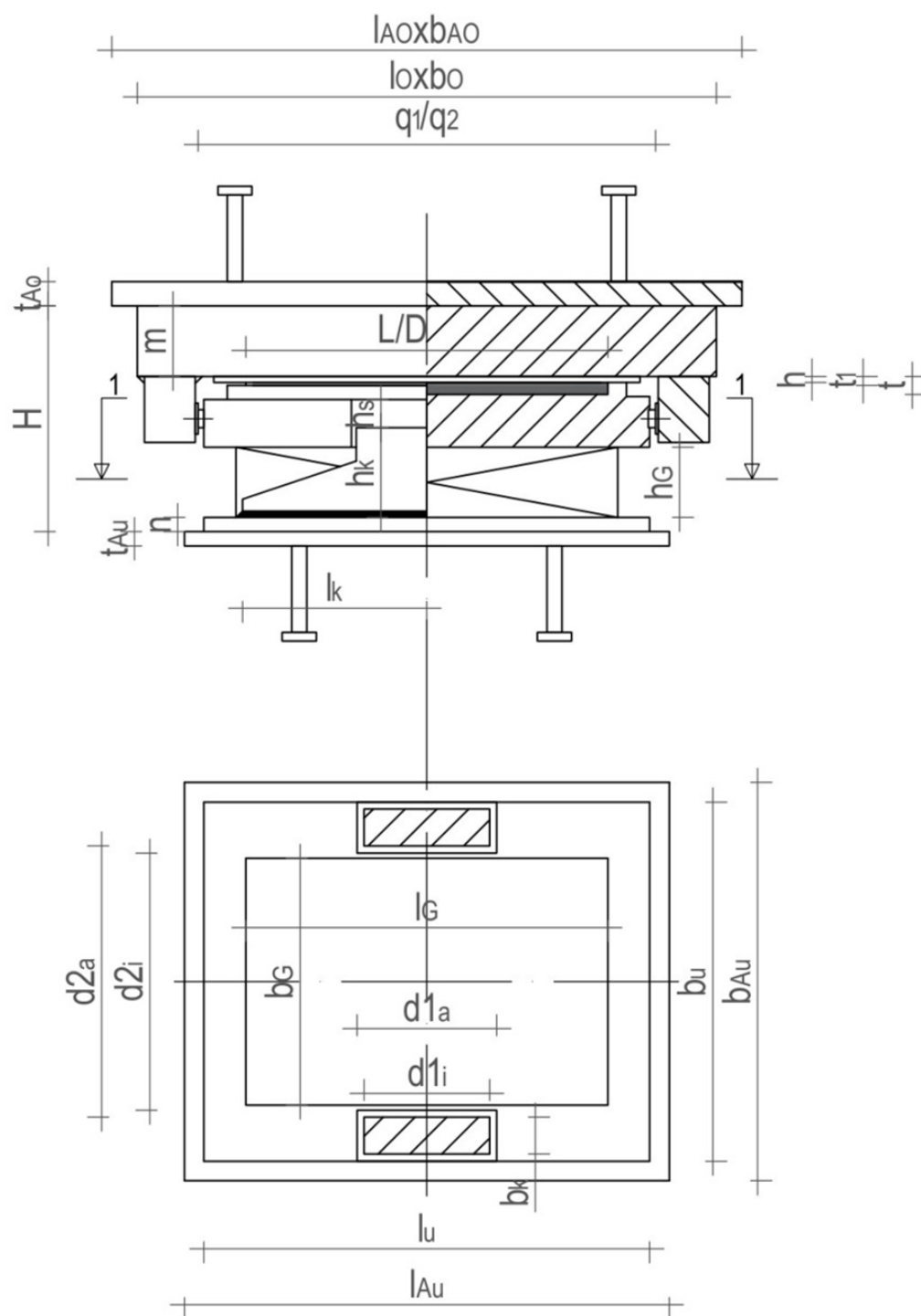
Slika 4.11: Prikaz dimenzij deformabilnega ležišča s preprečenimi pomiki v obeh smereh s pomočjo pridrževalne konstrukcije in vzdolžno drsnim delom na notranjem kontrolnem listu
