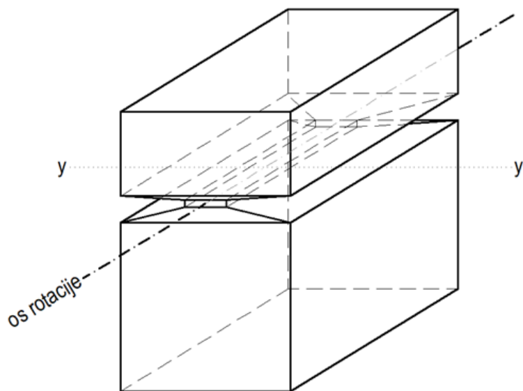
Slika 1.11: 3D skica betonskega členka.
