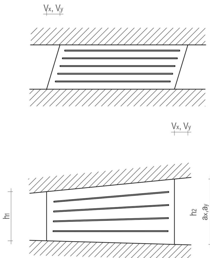
Slika 8.2: Meritve višin in deformacij deformabilnih – elastomernih - ležišč.
