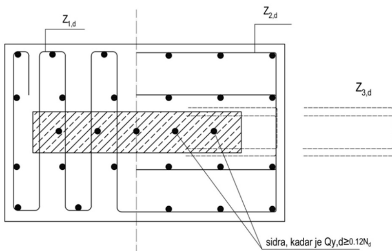
Slika 1.15: Skica armiranja priključnih elementov v tlorisu betonskega členka.
