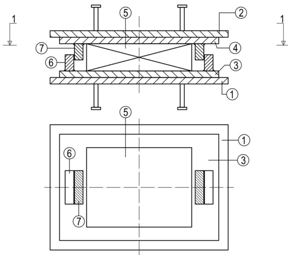
Slika 1.9: Shematski prikaz deformabilnega ležišča s preprečenimi pomiki v prečni smeri (1 – spodnja sidrna plošča; 2 – zgornja sidrna plošča; 3 – spodnja ležiščna plošča; 4 zgornja ležiščna plošča; 5 – deformabilno ležišče; 6 – spodnji strižni mozni; 7 – zgornji strižni mozni).
