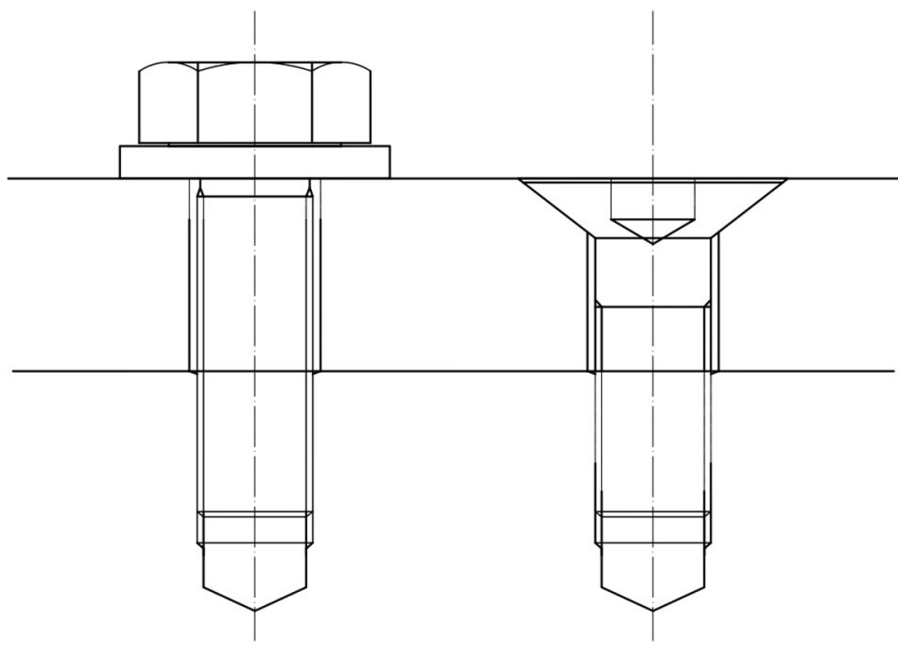
Slika 2.17: Skica vijčnega spoja ležišča v jekleno konstrukcijo
