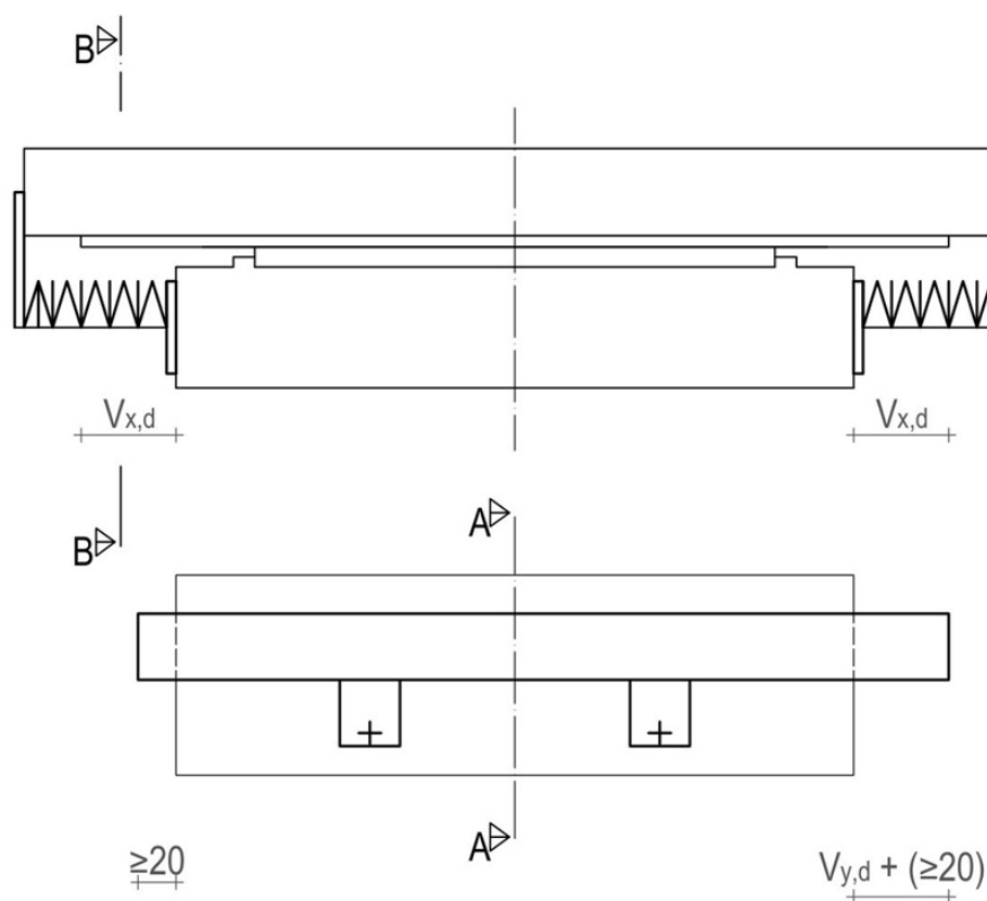
Slika 3.11: Shematski prikaz zaščite drsnih površin z mehom v obliki harmonike
