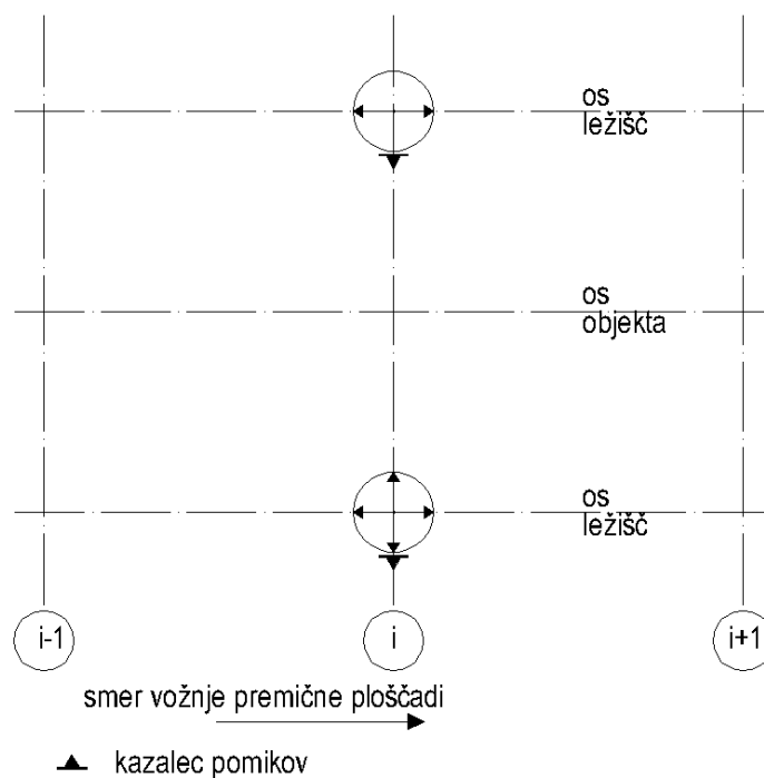
Slika 1.3: Situacija kazalca pomikov in mersko skalo, če je dostop za pregled ležišč omogočen s pomočjo premične ploščadi za pregled objektov.
