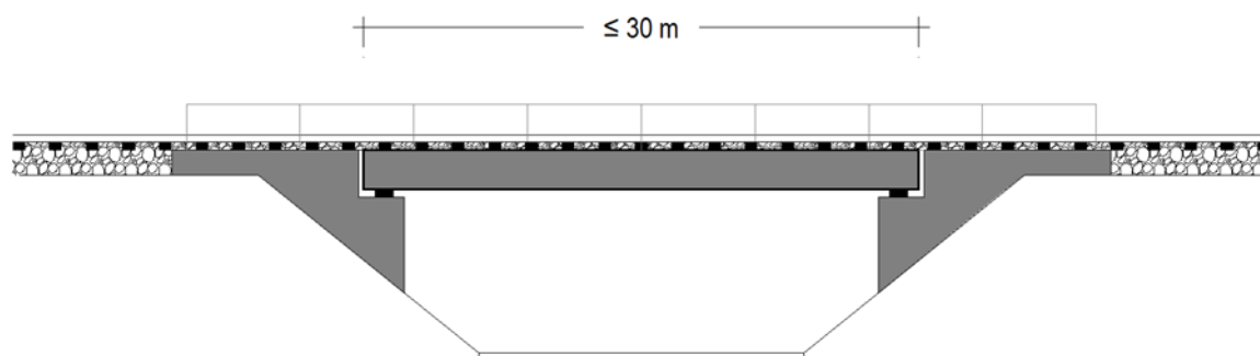
Slika 0.19: Shema elastičnega podpiranja v vzdolžnem prerezu železniškega premostitvenega objekta dolžine do 30 m preko enega polja.
