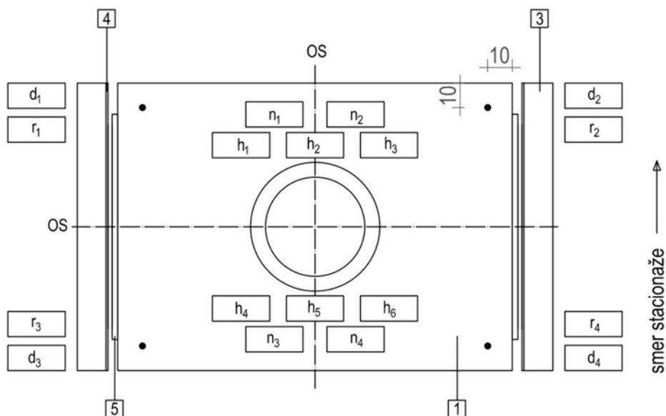
Slika 4.6: Prikaz meritev nagibnih špranj n_1 do n_4 ob robovih nosilne plošče [1] ( \approx 10/10 mm), drsnih špranj h_1 do h_6 , bočnih drsnih špranj d_1 do d_4 med drsno pločevino vodila ([4],[3]) in bočnim drsnim trakom [5] ter razmike r_1 do r_4 med drsno pločevino vodila ([4],[3]) in nosilno ploščo [1], ki so podane na notranjem kontrolnem listu
