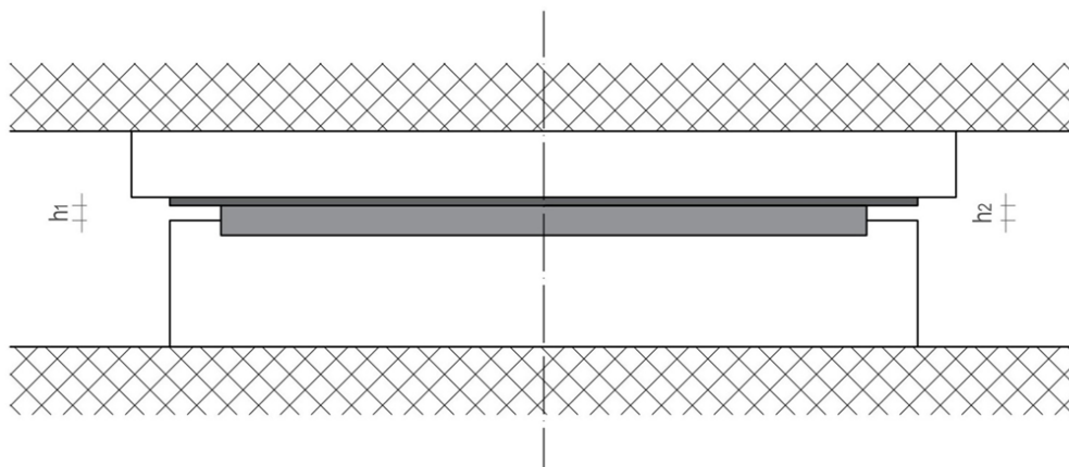
Slika 8.1: Meritve drsnih špranj.
