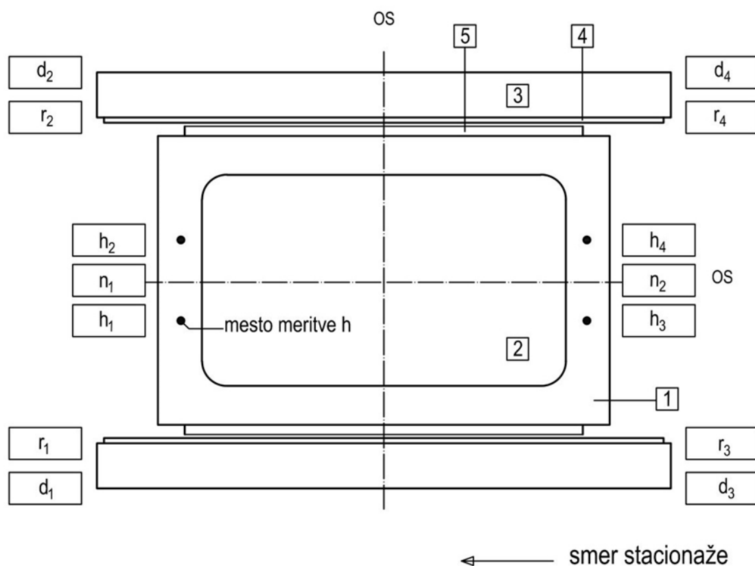
Slika 4.12: Prikaz meritev nagiba n_1 in n_2 v osi ležišča, drsnih špranj h_1 do h_4 , bočnih drsnih špranj d_1 do d_4 med drsno pločevino vodila ([4],[3]) in bočnim drsnim trakom [5] ter razmike r_1 do r_4 med drsno pločevino vodila ([4],[3]) in nosilno ploščo [1], ki so podane na notranjem kontrolnem listu
