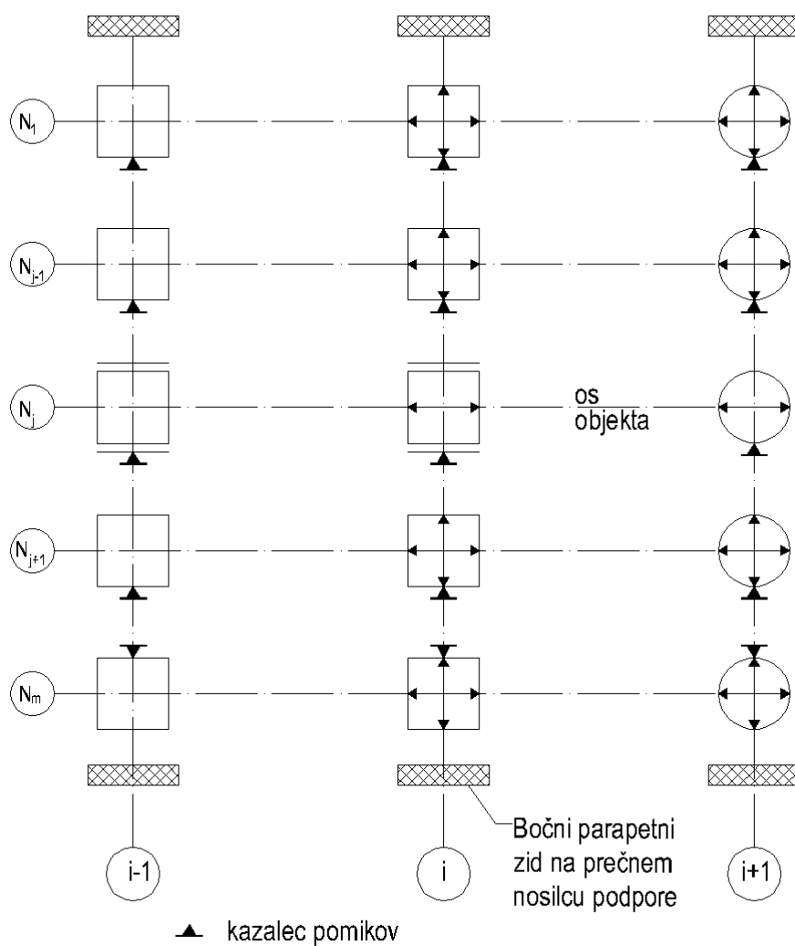
Slika 1.4: Situacija kazalca pomikov in mersko skalo pri objektih z bočnim parapetnim zidom na prečnem nosilcu podpore, ne glede na vrsto dostopa.
