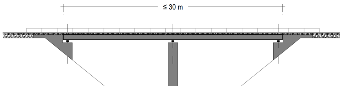
Slika 0.20: Shema elastičnega podpiranja v vzdolžnem prerezu železniškega premostitvenega objekta dolžine do 30 m preko dveh polj.
