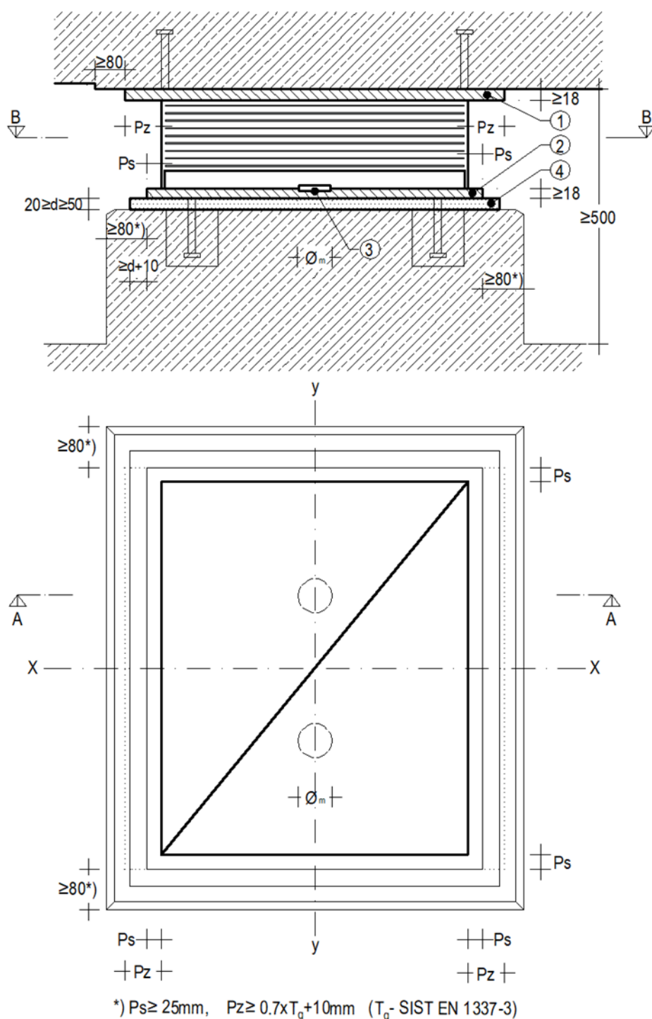
Slika 5.1: Prikaz vgradnje vsestransko pomičnega deformabilnega ležišča z glavnimi pomiki v vzdolžni smeri (1 – zgornja sidna plošča; 2 – spodnja sidna plošča; 3 – mozniček; 4 – podliva malta)
