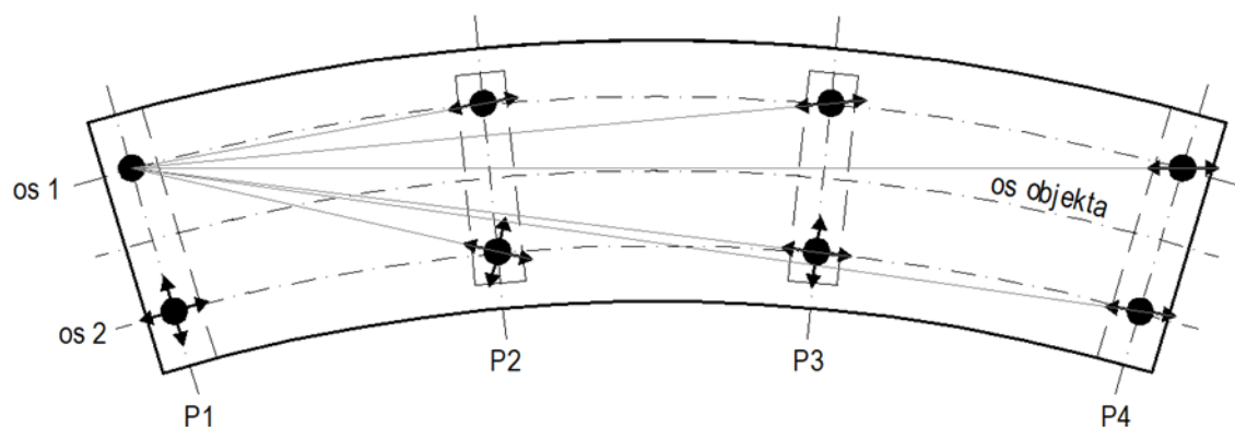
Slika 0.15: Shema polarnega podpiranja kontinuirane prekladne konstrukcije v krivini.
