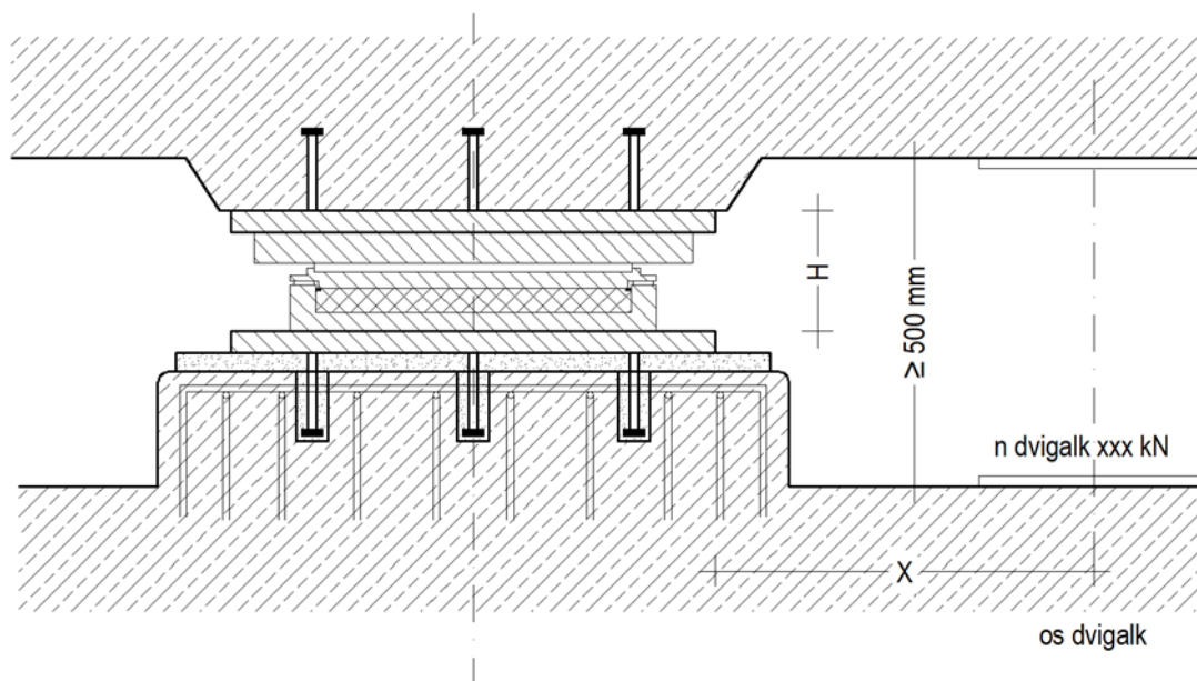
Slika 2.2: Shema sidranja ležišča s sidrno ploščo v betonski podstavek s podlivno malto in v betonsko prekladno konstrukcijo ter lokacijo jeklenih podložnih plošč za dvigalke. H je referenčna višina (do zgoranjega roba sidrne plošče).
