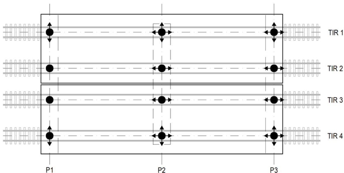
Slika 0.26: Shema podpiranja železniškega premostitvenega objekta z več kot dvema tiroma z vzdolžno dilatacijo s prevzemom horizontalnih sil na krajnem oporniku s fiksnim in prečno vodenimi ležišči
