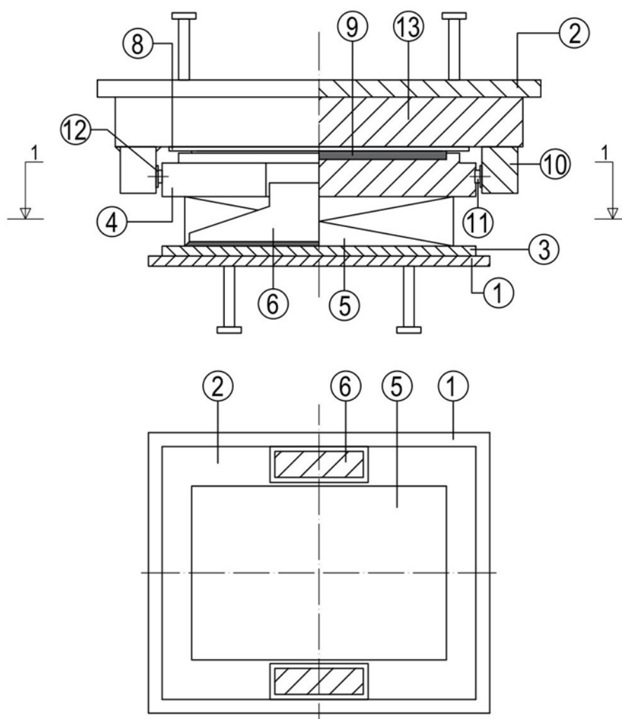
Slika 1.10: Shematski prikaz deformabilnega ležišča z vsestransko preprečenimi pomiki s pomočjo pridrževalne konstrukcije in nadgradnjo z drsnim delom z bočnima vodiloma v vzdolžni smeri (1 – spodnja sidrna plošča; 2 – zgornja sidrna plošča; 3 – spodnja ležiščna plošča; 4 zgornja ležiščna plošča; 5 – deformabilno ležišče; 6 – spodnji strižni moznik; 8 – drsna površina iz nerjavne pločevine; 9 – drsni disk; 10 – bočno vodilo; 11 – bočni drsni trak; 12 – bočna drsna površina iz nerjavne pločevine; 13 – drsna plošča).
