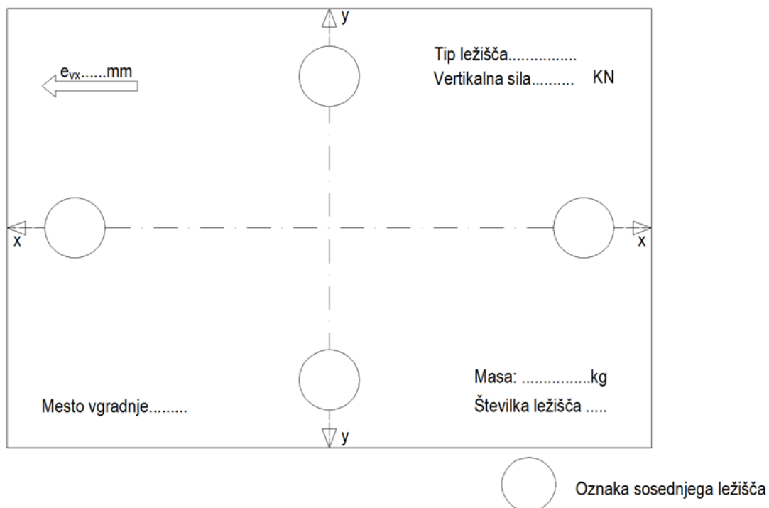
Slika 3.4: Oznake in podatki, ki morajo biti prikazani na zgornji površini pomičnega ležišča
