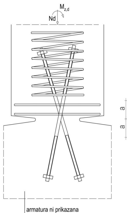
Slika 1.17: Skica armiranja sider v členku v prečnem prerezu betonskega členka.
