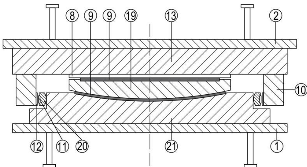
Slika 1.8: Shematski prikaz enostransko drsnega sfernega ležišča z bočnima vodiloma (1 – spodnja sidrna plošča; 2 – zgornja sidrna plošča; 8 – drsna površina iz nerjavne pločevine; 9 – drsni disk; 10 – bočno vodilo; 11 – bočni drsni trak; 12 – bočna drsna površina iz nerjavne pločevine; 13 – drsna plošča; 19 – sferna plošča; 20 – nagibna nosilna letev bočnega drsnega traku; 21 – nosilna ležiščna plošča).
