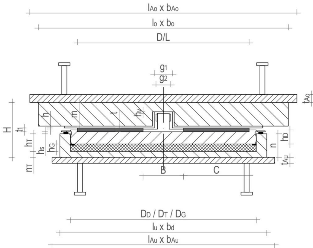
Slika 4.1: Prikaz dimenzij za drsno lončno ležišče s centralnim vodilom na notranjem kontrolnem listu
