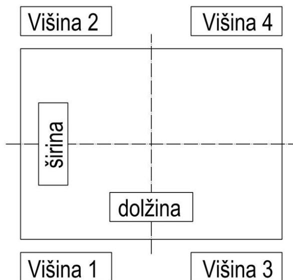
Slika 4.8: Prikaz meritev deformabilnega ležišča na notranjem kontrolnem listu
