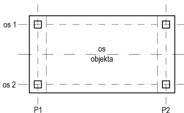
Slika 0.2: Shema elastičnega podpiranja mostu preko enega polja s fiksno točko v sredini razpetine mostu.
