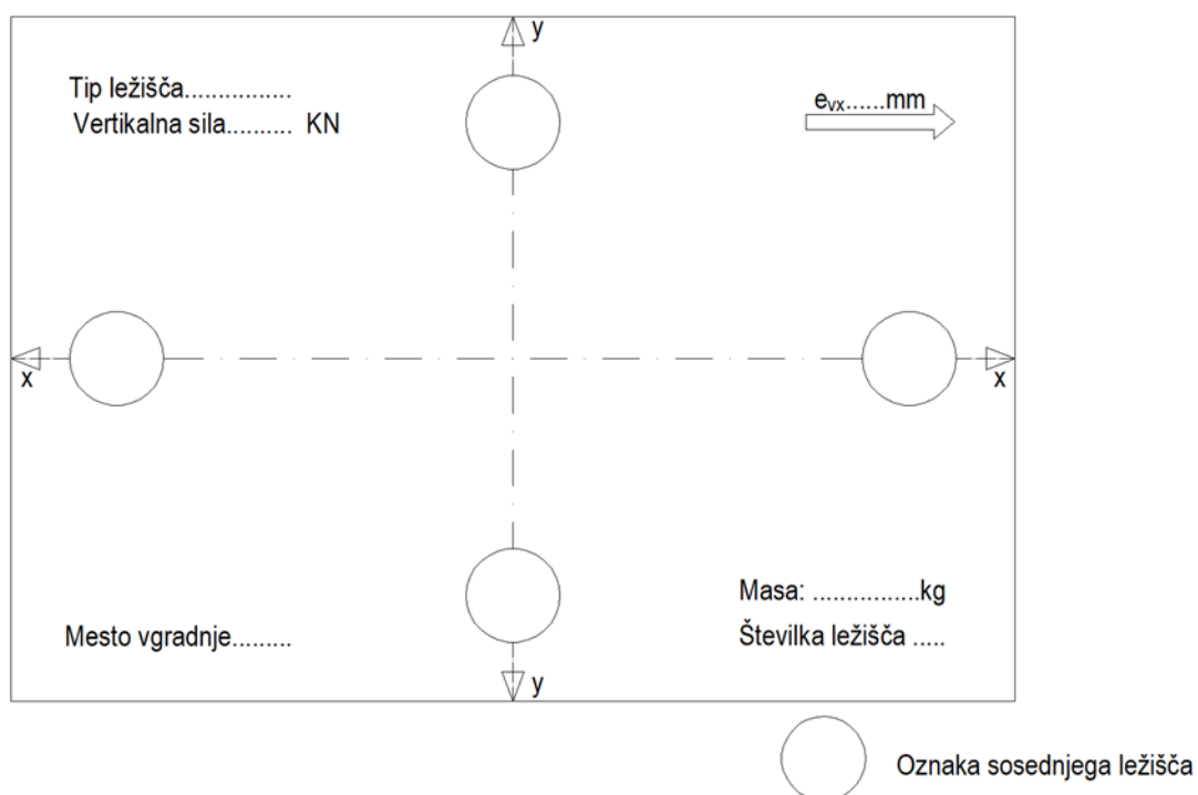
Slika 3.3: Oznake in podatki, ki morajo biti prikazani na zgornji površini pomičnega ležišča
