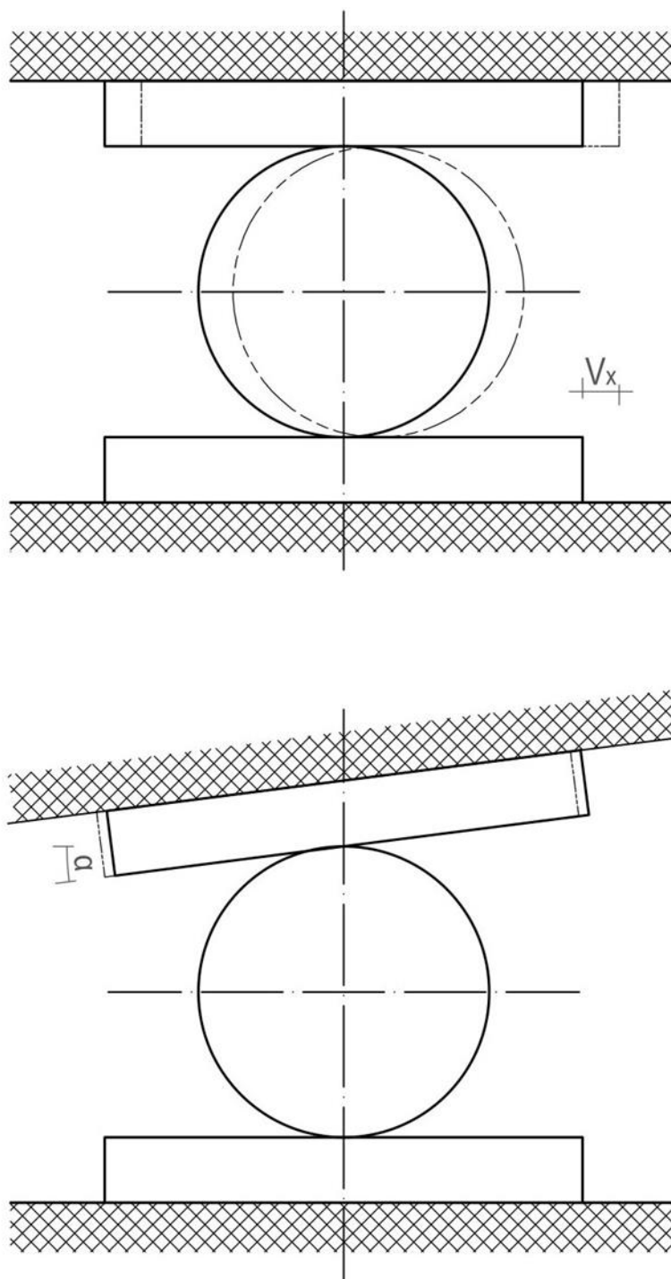
Slika 8.7: Meritve pomika in zasuka valjčnega ležišča.
