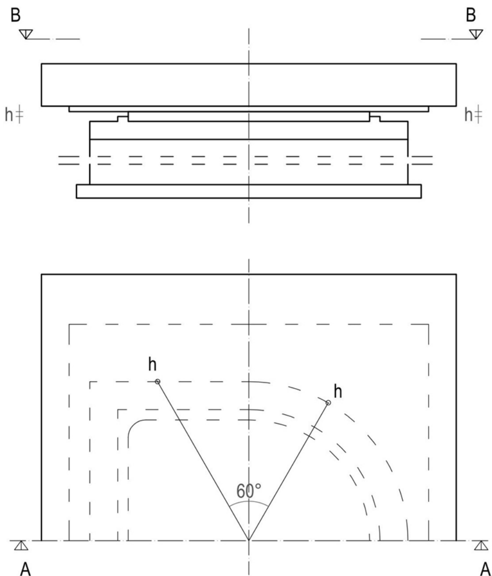
Slika 3.6: Merilne točke drsne špranje h pri deformabilnem vsestransko drsnim ležiščem v osi glavnih pomikov za pravokotno in okroglo ležišče
