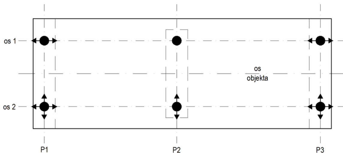
Slika 0.18: Shema podpiranja za prevzem horizontalnih sil v vzdolžni smeri s fiksnim in prečno pomičnim ležiščem. Takšna shema podpiranja se ne priporoča razen v primeru, kadar so zagotovljeni posebni pogoji za maksimalno vsoto širin vseh špranj drsnega ležišča.
