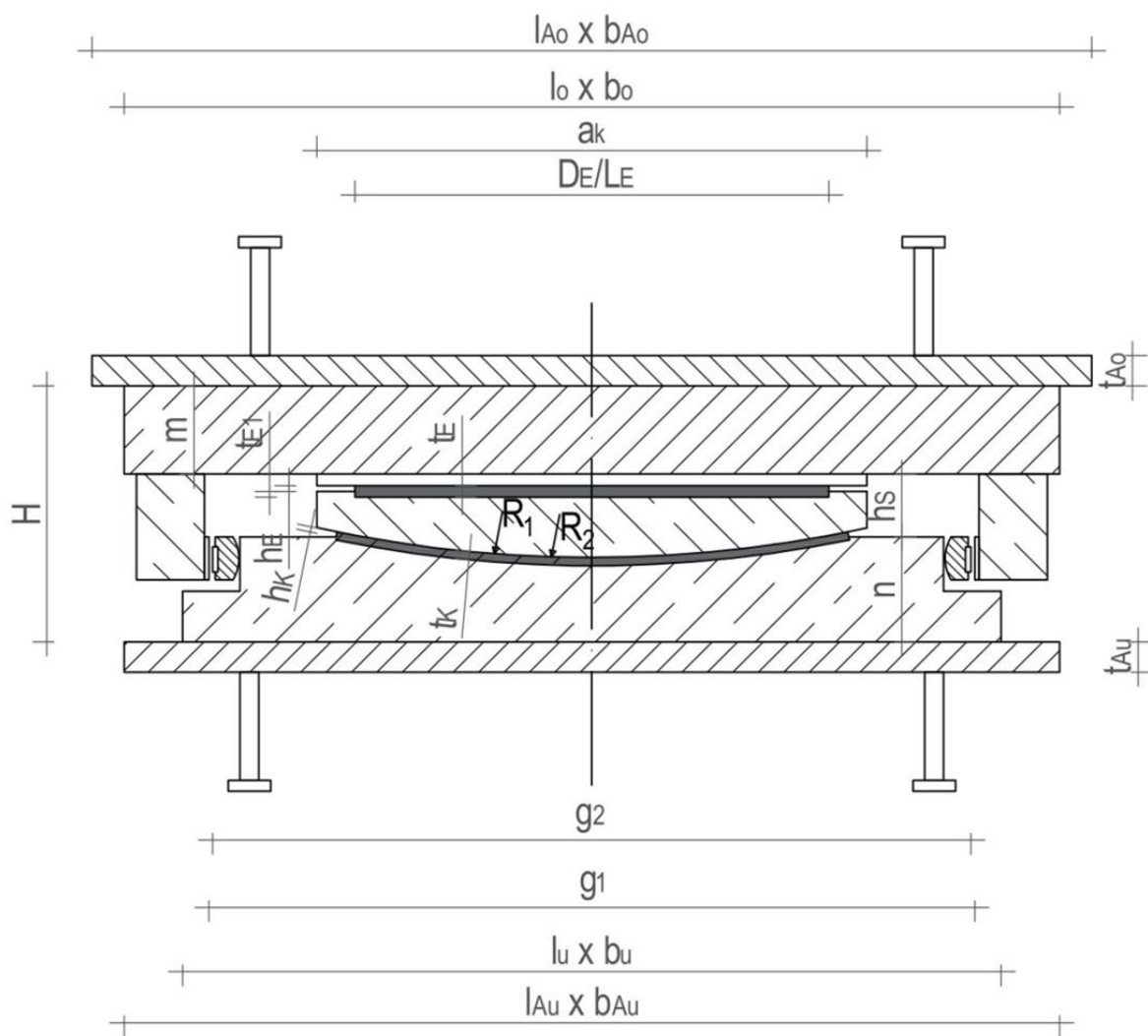
Slika 4.4: Prikaz dimenzij za drsno sferno ležišče z bočnima vodiloma na notranjem kontrolnem listu
