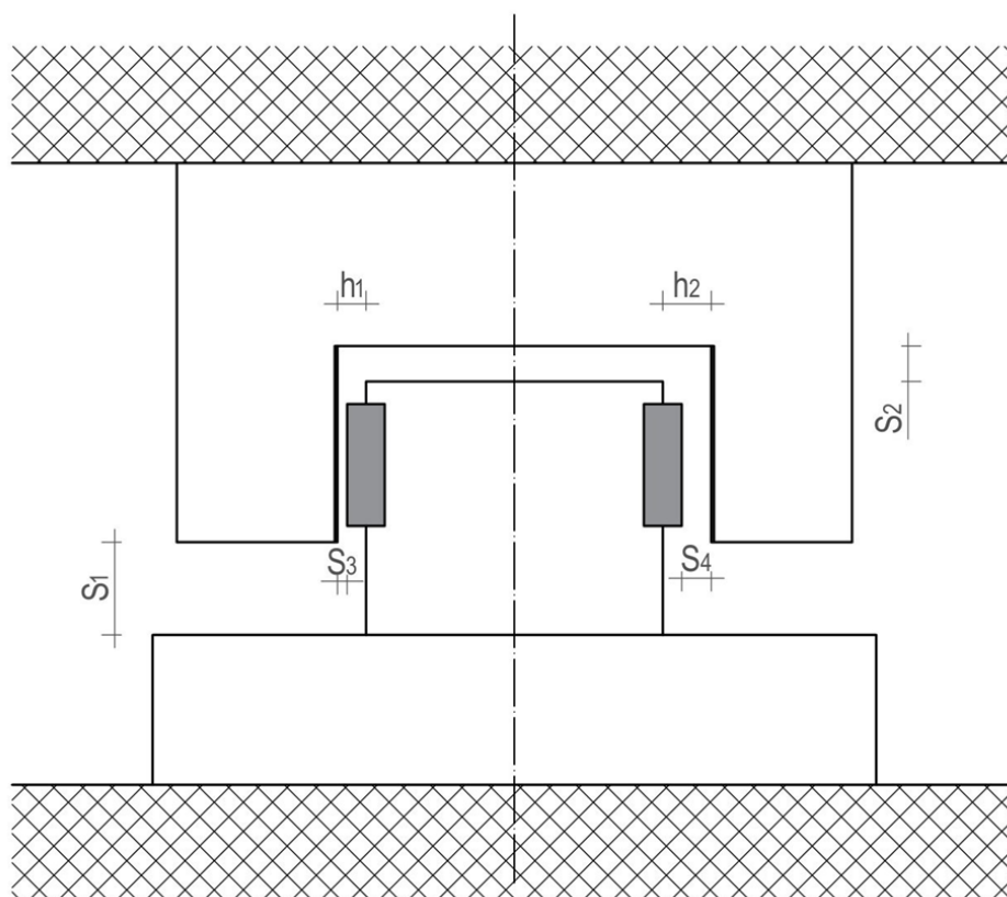
Slika 8.6: Meritve drsniš špranj s_3 in s_4 , razmikov med trnom (vodilom) in zgornjim nosilnim delom ležišča h_1 in h_2 , vertikalnega razmika s_1 med spodnjo in zgornjo nosilno ploščo ter s_2 med zgornjo površino vodila in spodnjo površino zgornje nosilne plošče nad vodilom vodenega ležišča.
