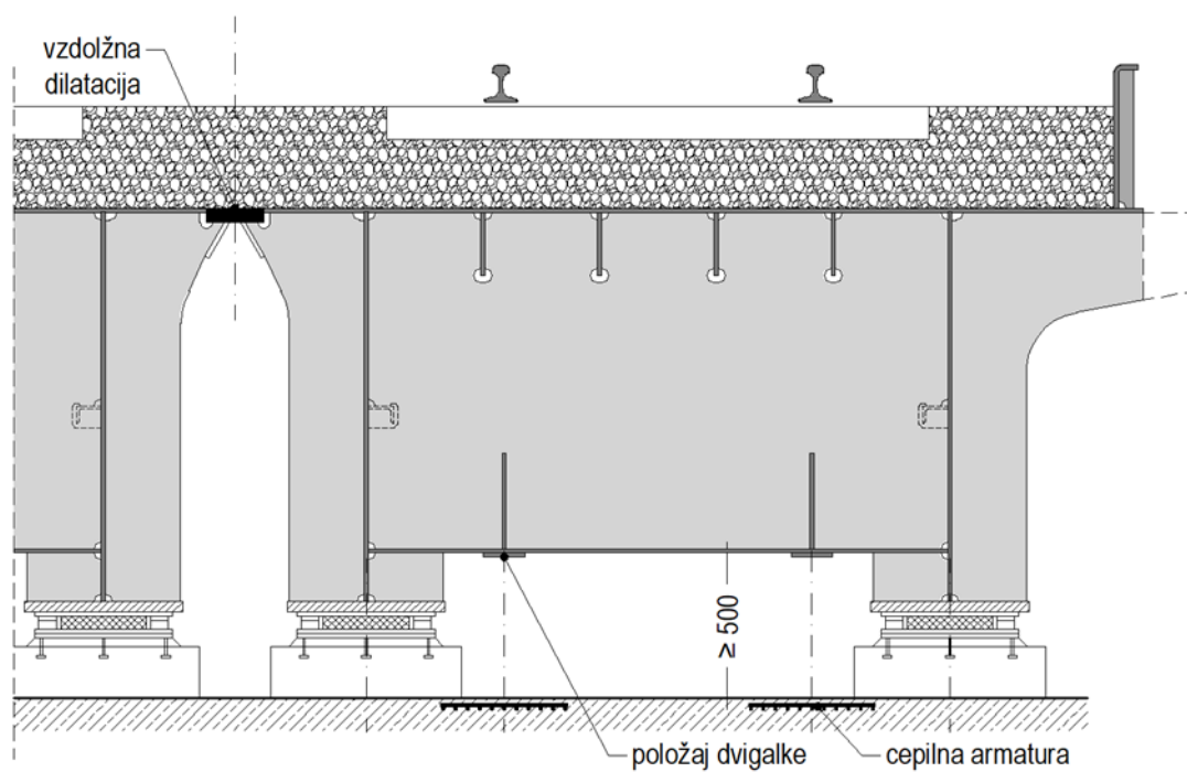
Slika 2.8: Ojačitve prečnika prekladne konstrukcije iz polnostenskih nosilcev nad drsnim ležiščem in v področju predvidenih dvigalk.
