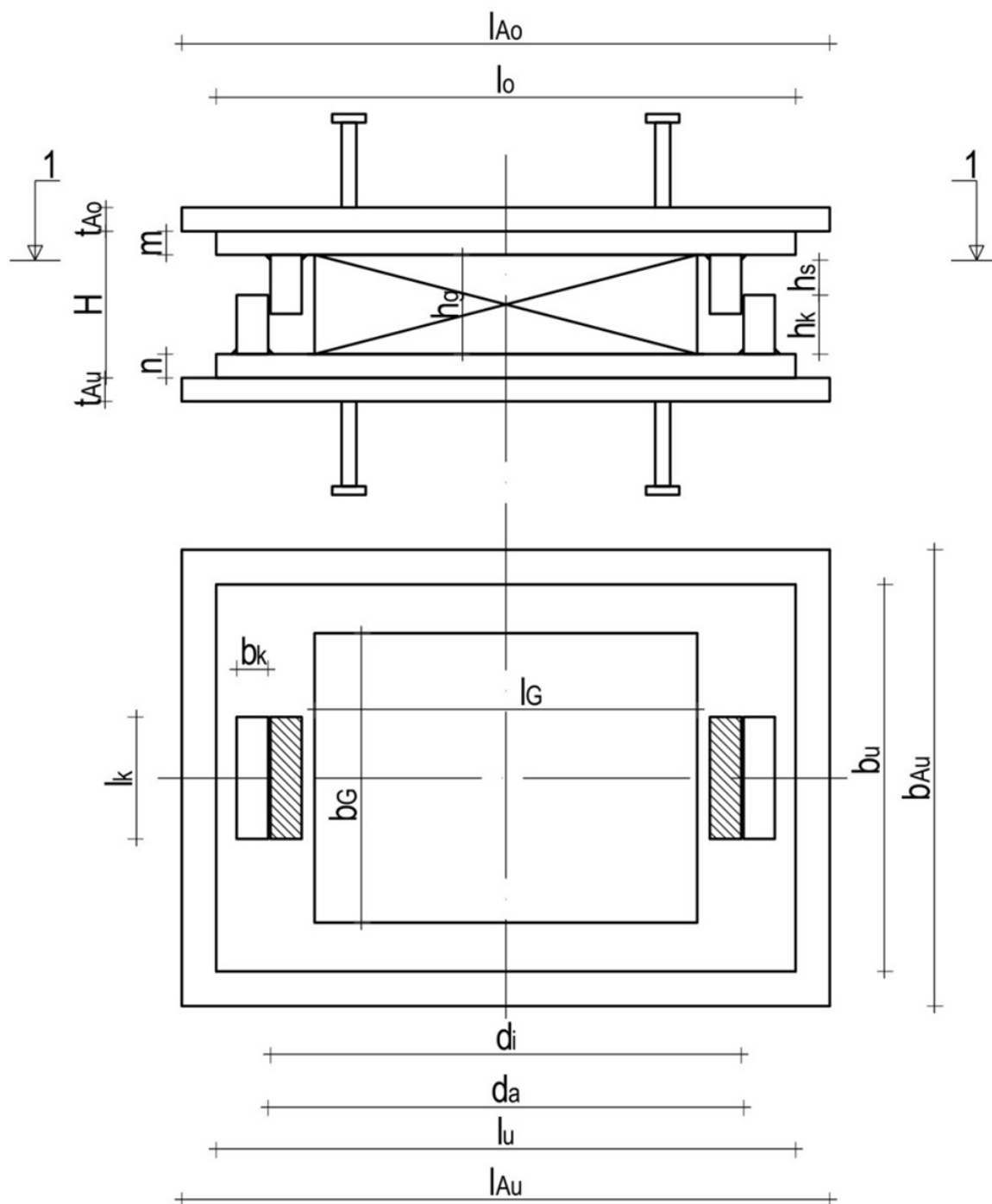
Slika 4.9: Prikaz dimenzij deformabilnega ležišča z ležiščnima in sidrnima ploščama in preprečenimi pomiki v prečni smeri na notranjem kontrolnem listu
