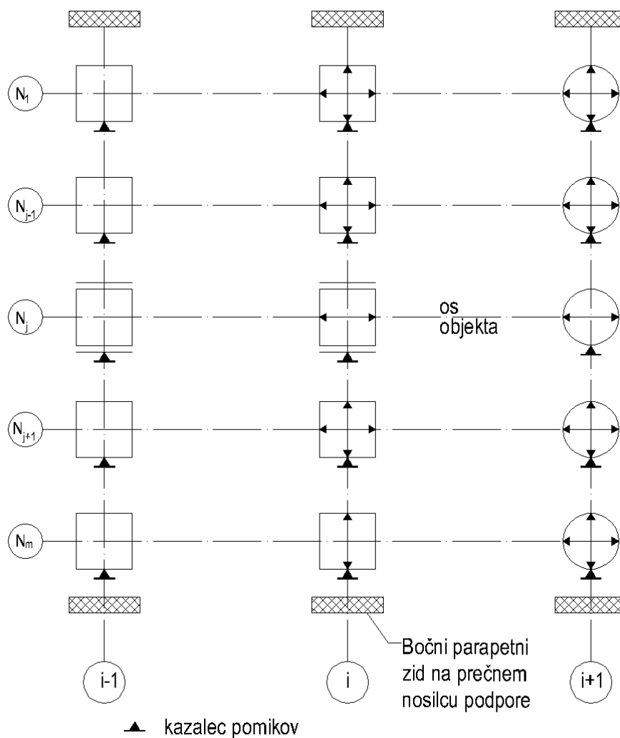
Slika 1.5: Nepravilna situacija kazalca pomikov v osi N_m in mersko skalo pri objektih z bočnim parapetnim zidom na prečnem nosilcu podpore, ne glede na vrsto dostopa.
