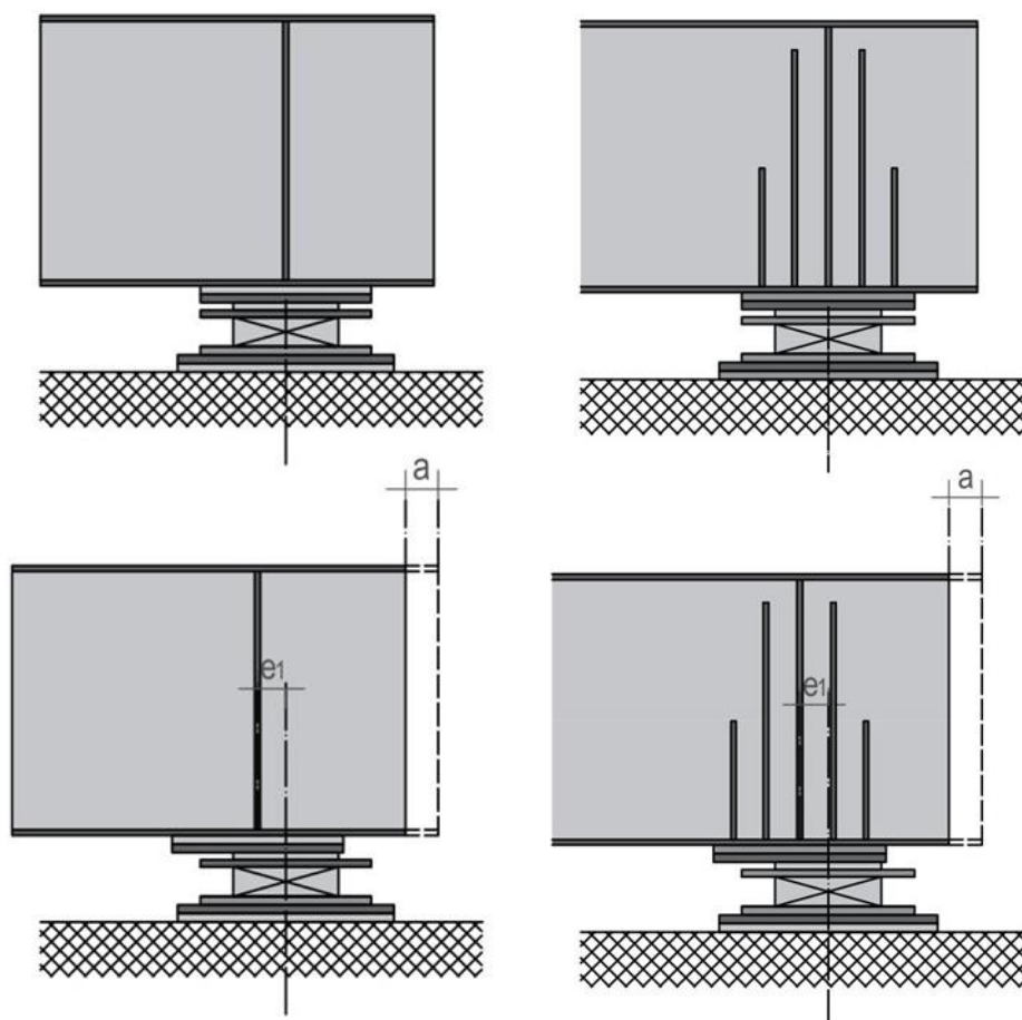
Slika 2.11: Jekleni nosilec nad drsnim ležiščem brez ojačitve in z ojačitvami v vzdolžni smeri za prenos tlačnih sil v področju pomikov ležišča.
