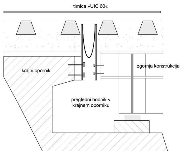
Slika 3.16: Blazinasta dvojna zaprta dilatacija na srednje dolgih železniških objektih
