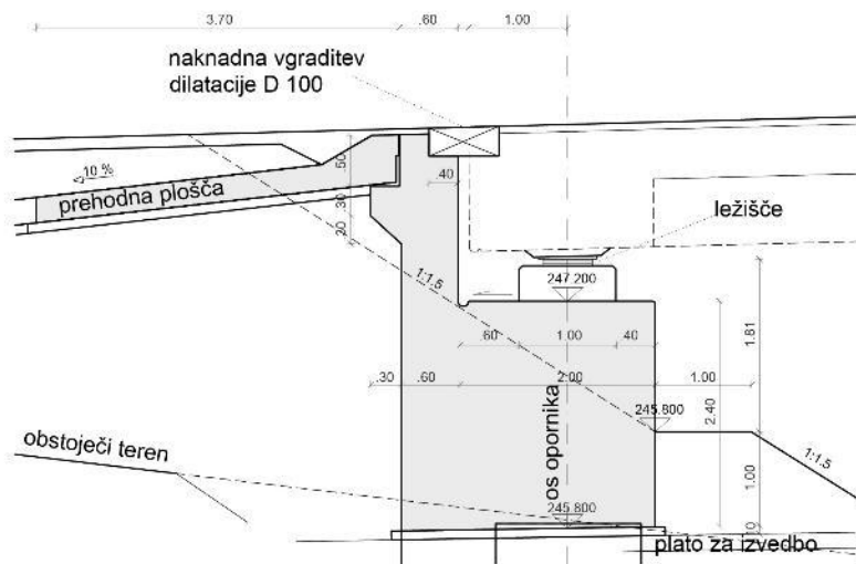
Slika 3.1: Shema dilatiranja (krajni podpori) v vzdolžnem prerezu cestnega premostitvenega objekta dolžine do 50 m
