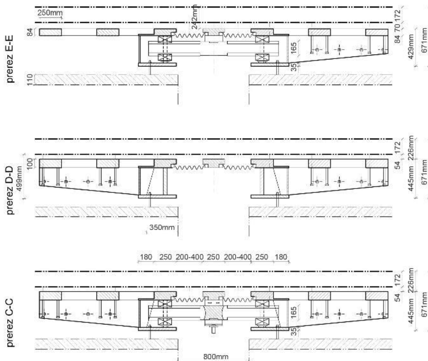
Slika 4.25: Shematski prikaz železniške drsne pragovne dilatacije v povezavi s tirom na togi podlagi za velike in zelo velike pomike ter način podpiranja z ležišči in vzmetmi (sistem Maurer)
