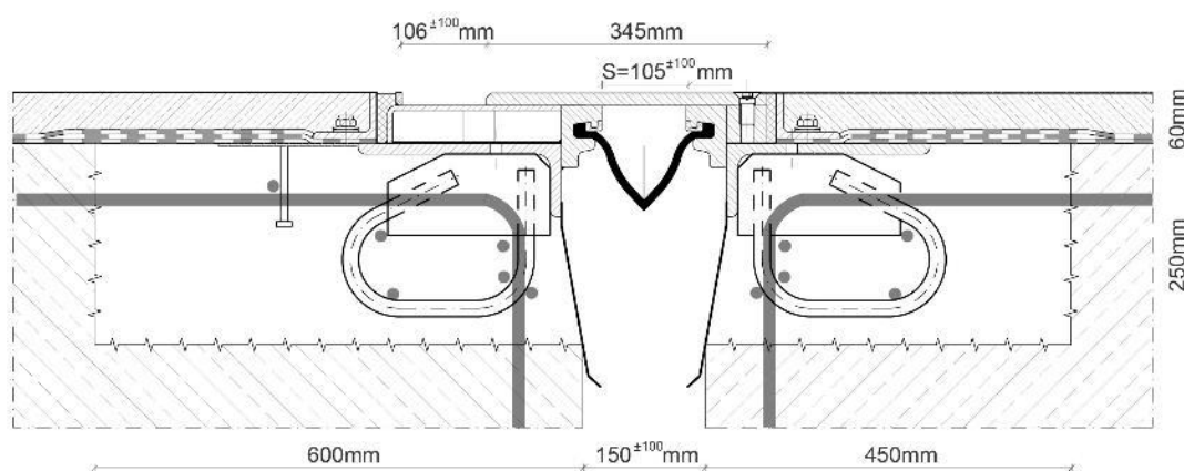
Slika 4.21: Shematski prikaz železniške podprte dilatacije z drsko ploščo
