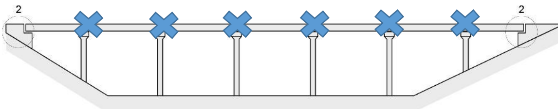
Slika 3.3: Shema dilatiranja (krajni podpori) v vzdolžnem prerezu cestnega premostitvenega objekta, viadukta dolžine do 400 m preko ene zavrne enote
