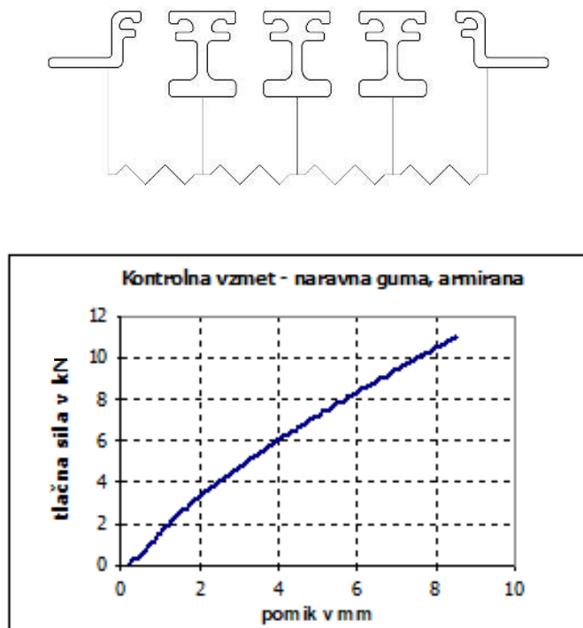
Slika 5.2: Shema krmilnih vzmeti pri lamelni dilataciji ter lastnost Hookove vzmeti za ta namen (sistem Mageba)
