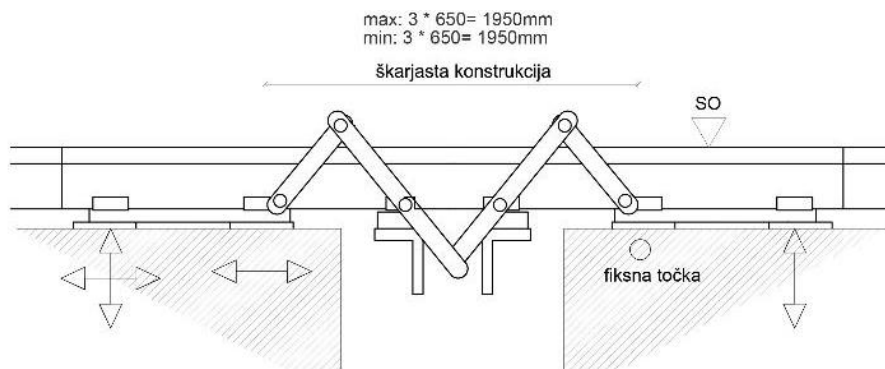
Slika 4.26: Shema podprte drsne dilatacijske plošče za tir na togi podlagi (sistem STOG)
