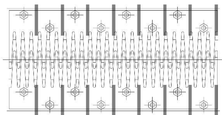
Slika 4.20: Shematski prikaz cestne konzolne dilatacije s ploščami z glavniki, z dvorednimi sidri (prerez in tloris)
