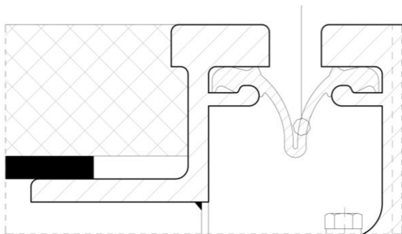
Slika 13. 28: Primer neustreznega vpetja elastomernega traku v čeljusti robnega in vmesnega profila (točkovno tesnjenje namesto linijskega tesnjenja po obodu utora), tehnična vodotesnost ni zagotovljena
