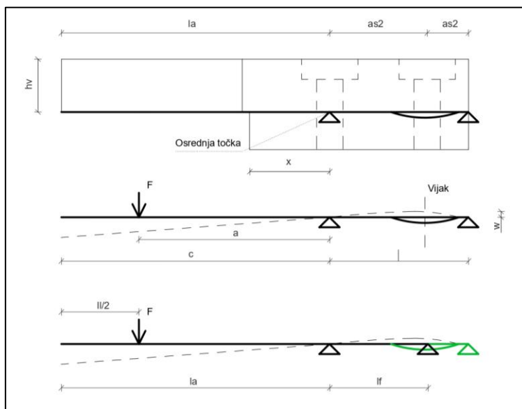
Slika 13.23: Statični sistem pri konzolni glavnikasti dilataciji (dvorednost vpetja) in deformacija dilatacije pod prometno obtežbo - neravnina ob vpetju (vijaku) je lahko vzrok za odpoved sidrnega sistema
