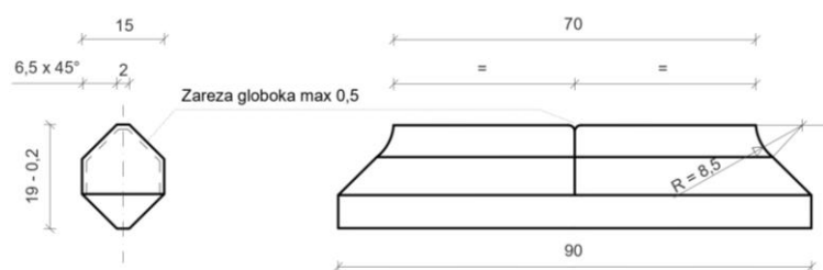
Slika 13.17: Na utrujanje nezadostno zasnovani zvari vitalnih jeklenih delov npr. zvarov med lamelami in prečkami. Znan primer so lamelne gredne jeklene dilatacije proizvajalca Maurer tipa DT proizvodnje od 1981 do 2003
