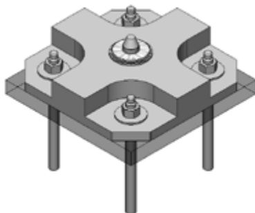
Slika 6.13: Montažna noga železniške drsne pragovne dilatacije tipa Maurer
