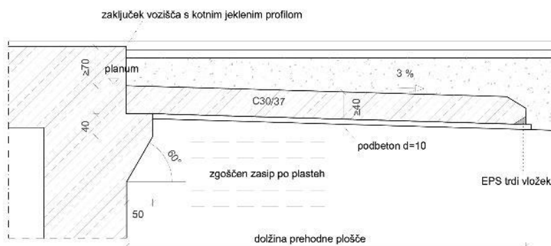
Slika 3.5: Primer zaključka s pokrito dilatacijo (jeklen kotni profil z bitumensko rego) in prehodno ploščo integralnega podvoza do 30 m
