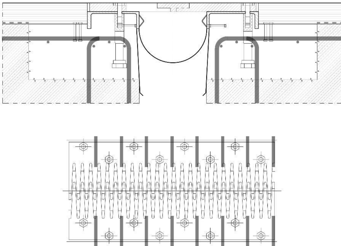
Slika 4.19: Shematski prikaz cestne konzolne dilatacije s ploščami z glavniki, z dvorednimi sidri (prerez in tloris)
