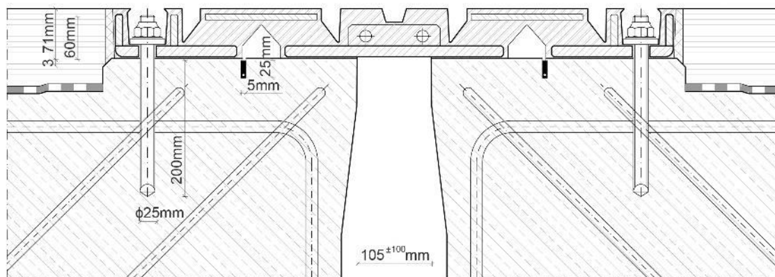
Slika 4.17: Shematski prikaz cestne ali železniške blazinaste dilatacije za masivni premostitveni objekt (prerez)
