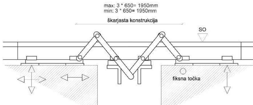
Slika 4.25: Shema podprte- drsne dilatacijske plošče za tir na togi podlagi (sistem STOG)
