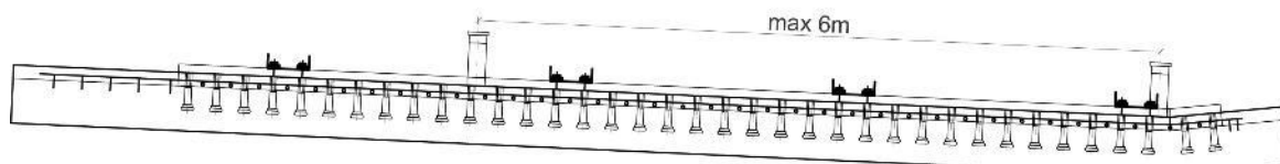
Slika 6.12: Položaj vmesnih cevi za polnjenje s SCC betonom max. 6 m
