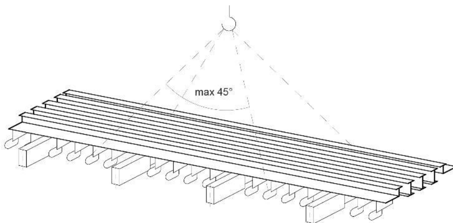
Slika 6.7: Shema dviznih vrvi pri dvigu in spustu lamelne dilatacije – vpenjalna mesta označena z barvo
