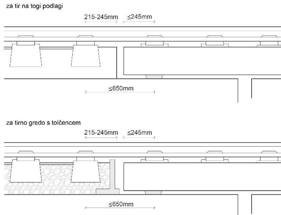
Slika 3.21: Shema odmikov robov in pragov za kompenzacijske dilatacije v vzdolžnem prerezu železniškega premostitvenega objekta
