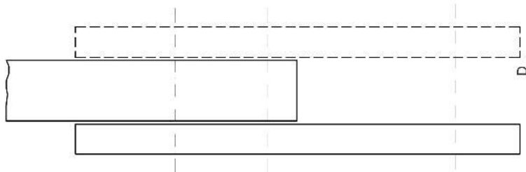
Slika 5.4: Skica odstopanja od ravnosti med podlago in jekleno ploščo – D, po SIST EN 1090
