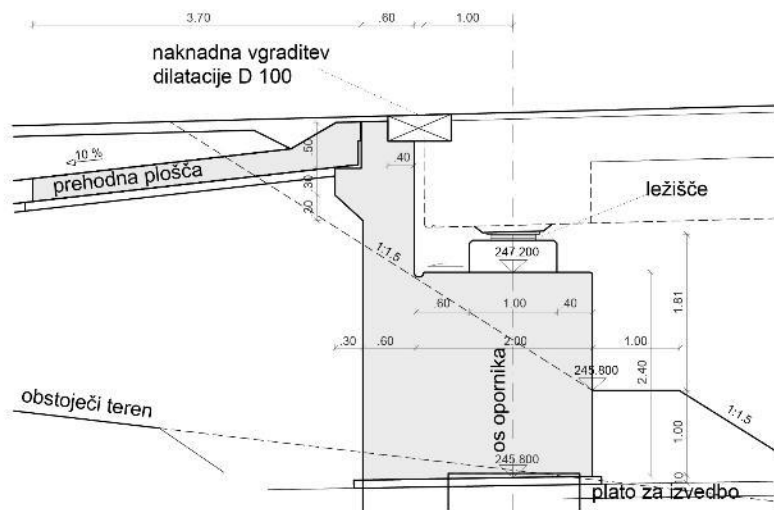
Slika 3.1: Shema dilatiranja (krajni podpori) v vzdolžnem prerezu cestnega premostitvenega objekta, podvoza dolžine do 50 m preko treh polj
