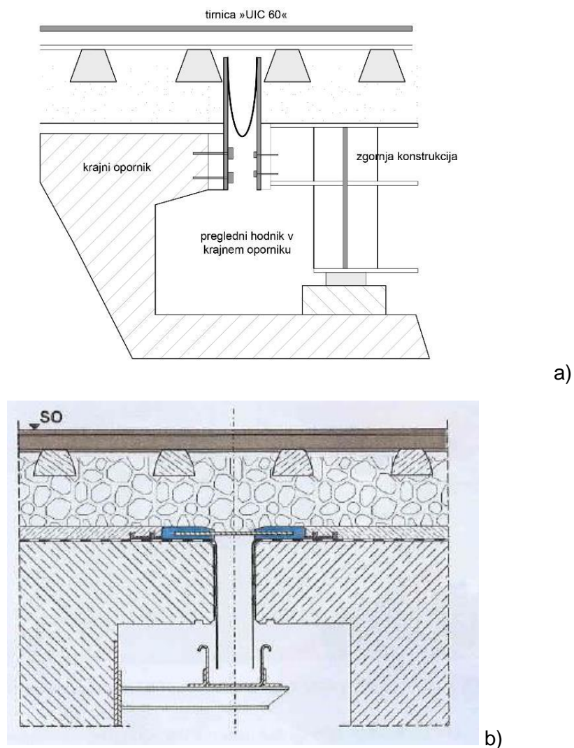
Slika 3.17: Primeri odprte dilatacije železniškega premostitvenega objekta z neprekinjeno tirno gredo (primera a in b)
