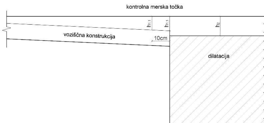
Slika 6.3: Merilne točke robnega stika dilatacije s priključnim voziščem
