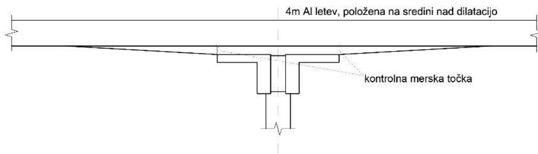
Slika 6.2: Meritev ravnosti vgrajene cestne dilatacije z voziščem, s 4 m Al letvijo in kontrolni višinski točki
