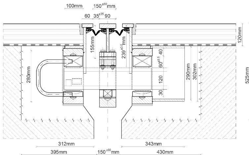
Slika 4.21: Shematski prikaz cestne lamelne dilatacije (prerez)
