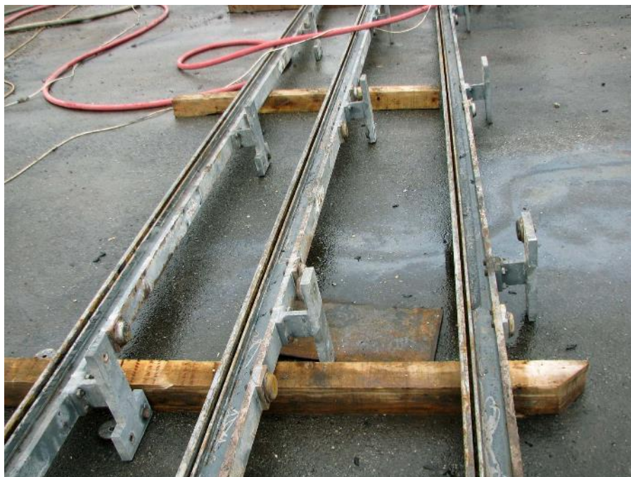
Slika 8.2: Razstavljena dilatacija na platuju v delavnici -vmesne lamele s krmilnimi deli
