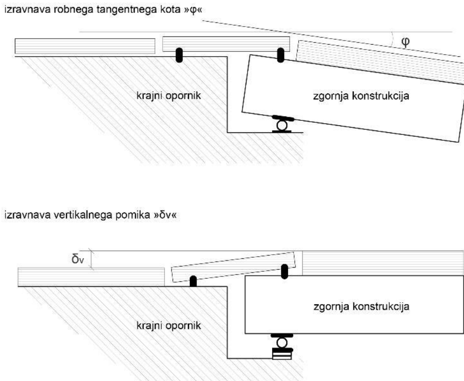
Slika 3.20: Shema premoščanja gradbene odprtine železniškega premostitvenega objekta s tirom na togi podlagi s kompenzacijskimi ploščami kot sistem dilatacij
