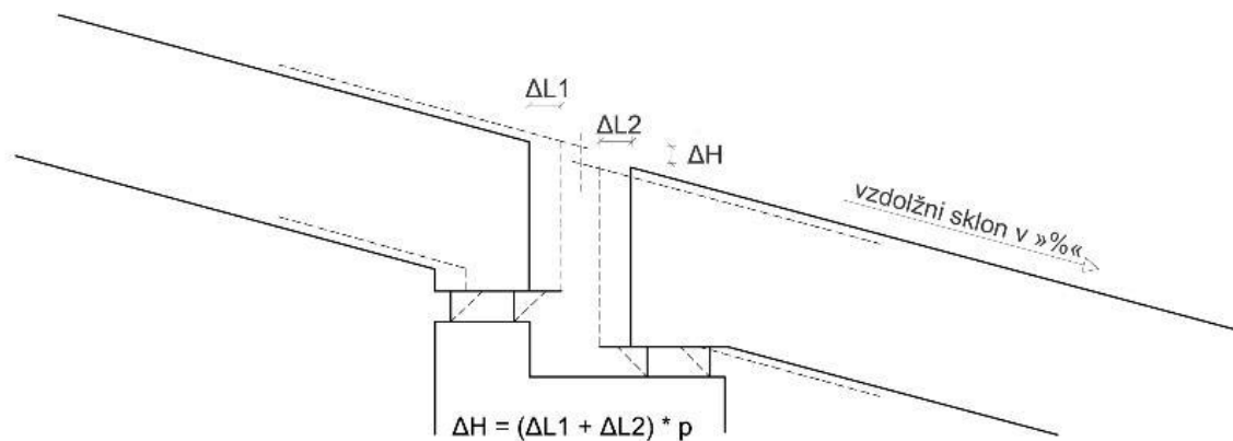
Slika 4.7: Shema vpliva vzdolžnega sklona prekladne konstrukcije z dilatacijo
