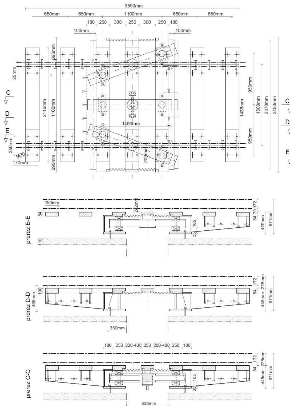
Slika 4.24: Shematski prikaz železniške drsne pragovne dilatacije v povezavi s tirom na togi podlagi za velike in zelo velike pomike ter način podpiranja z ležišči in vzmetmi (sistem Maurer)
