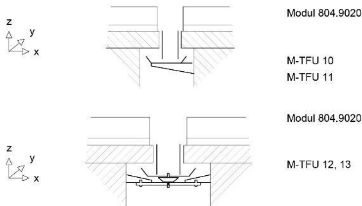
Slika 4.23: Shematski prikaz železniške odprte dilatacije v povezavi s tirom na togi podlagi za velike in zelo velike pomike ter način odvodnjavanja z lovilnim kanalom spodaj
