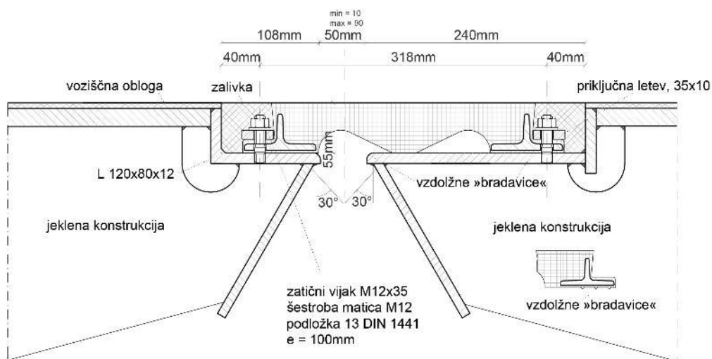
Slika 4.18: Shematski prikaz železniške blazinaste dilatacije za jekleni premostitveni objekt (prerez)
