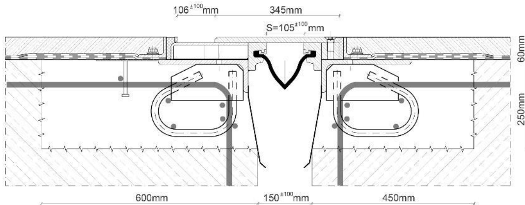
Slika 4.20: Shematski prikaz železniške podprte dilatacije z drsno ploščo
