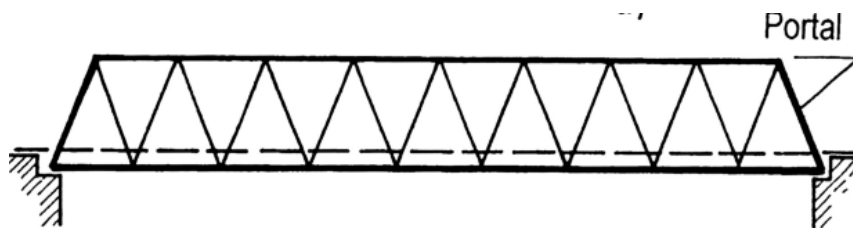
Slika 3.7: Shema dilatiranja in prehoda na krajnih opornikih v vzdolžnem prerezu železniškega premostitvenega objekta z jeklenim paličjem, dolžine do 50 m, preko enega polja
