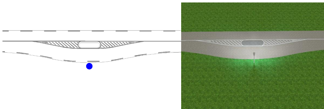
Slika 47: Primer postavitve svetilk za osvetlitev deniveliranega otoka za zamik osi smernega vozišča iz ene strani ceste
