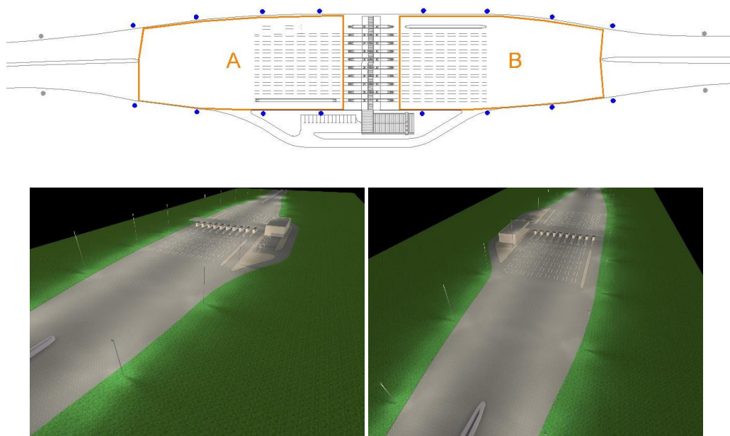
Slika 37: Primer postavitve svetilk za osvetlitev kontrolne postaje
