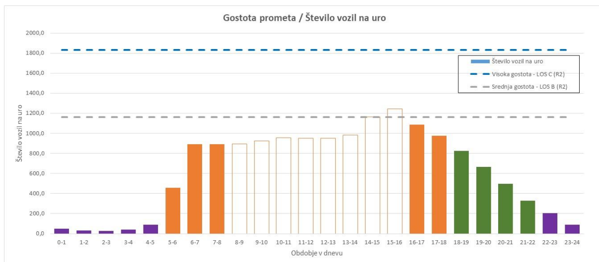
Slika 1: Pregled gostote prometa za obravnavani odsek ceste
