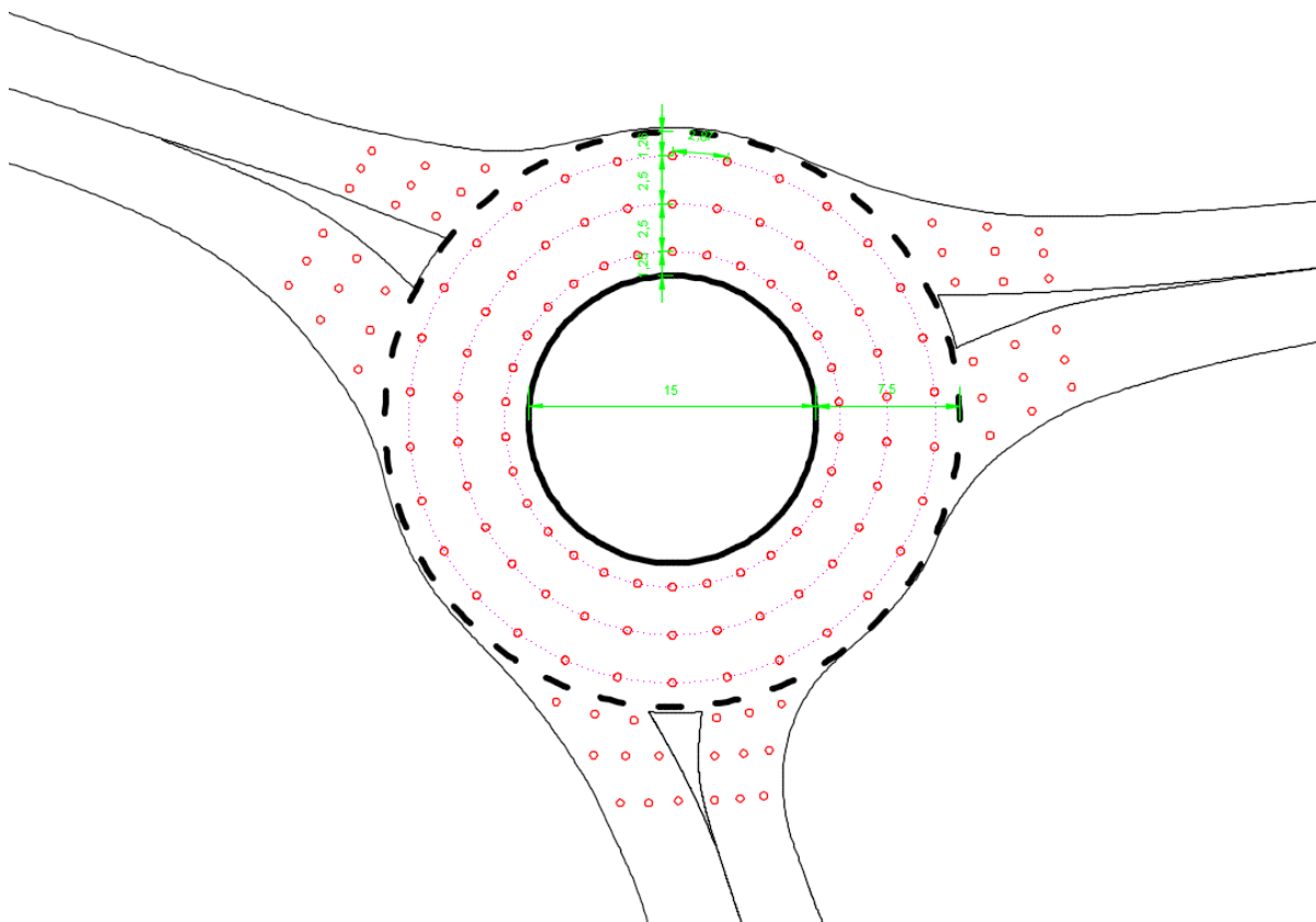
Slika 53: Primer merilne mreže pri meritvi osvetljenosti v krožnem križišču
