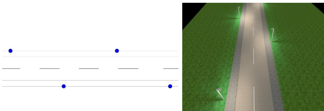
Slika 18: Primer postavitve zamaknjenih svetilk na obeh straneh ceste za osvetlitev površin za pešce na neobremenjenem delu ceste v naselju
