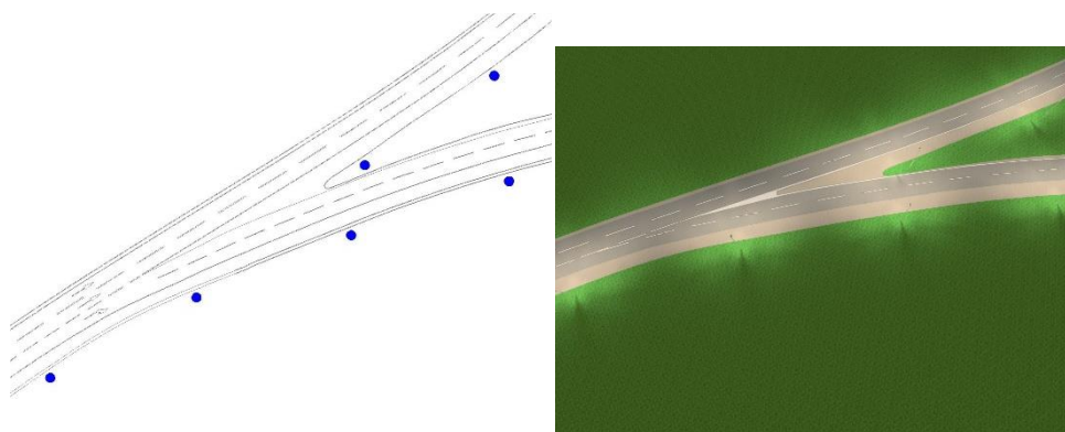
Slika 22: Primer postavitve svetilk za osvetlitev razcepa na avtocesti
