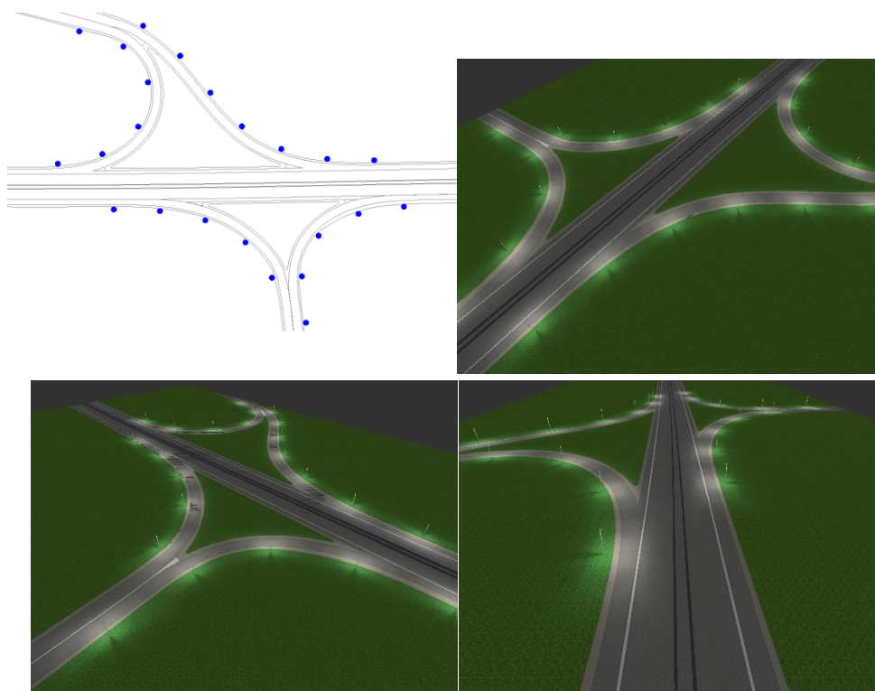
Slika 26: Primer postavitve svetilk za osvetlitev uvoza in izvoza na avtocesti oziroma hitri cesti
