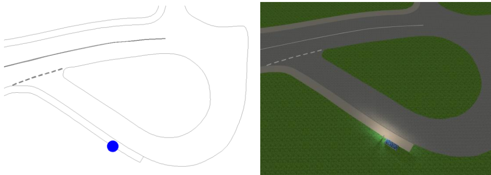
Slika 36: Primer postavitve svetilk za osvetlitev obračališča
