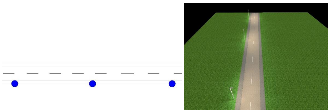
Slika 17: Primer postavitve svetilk na eni strani ceste za osvetlitev površin za pešce na neobremenjenem delu ceste v naselju
