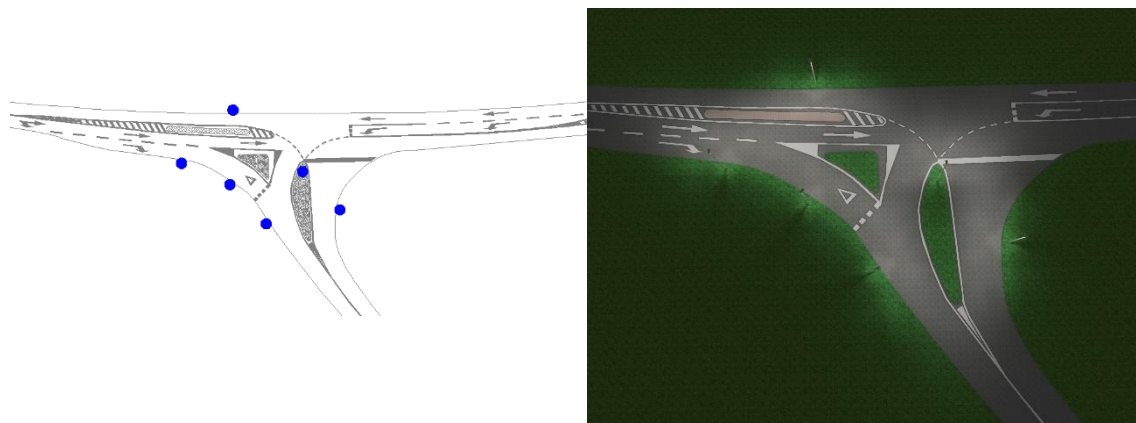
Slika 46: Primer postavitve svetilk za osvetlitev deniveliranih otokov v križišču
