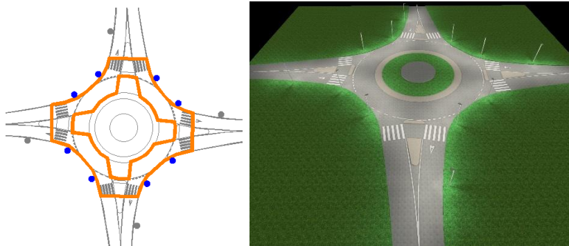
Slika 41: Primer postavitve svetilk za osvetlitev krožnega križišča z vključenimi prehodi za pešce
