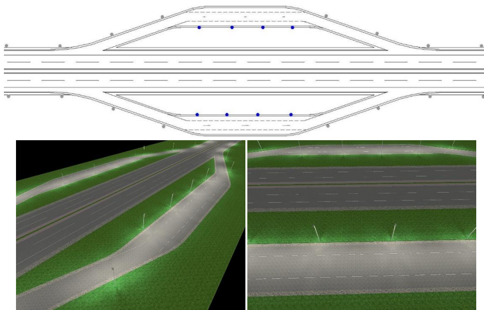
Slika 33: Primer postavitve svetilk za osvetlitev počivališča
