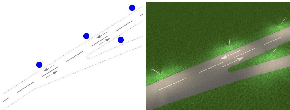
Slika 24: Primer postavitve svetilk za osvetlitev razcepa na daljinski cesti
