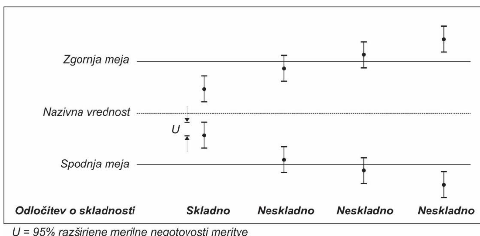
Slika 56: Pravilo odločanja z upoštevanjem merilne negotovosti meritve
