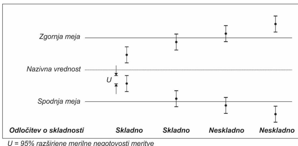
Slika 55: Pravilo odločanja brez upoštevanja merilne negotovosti meritve
