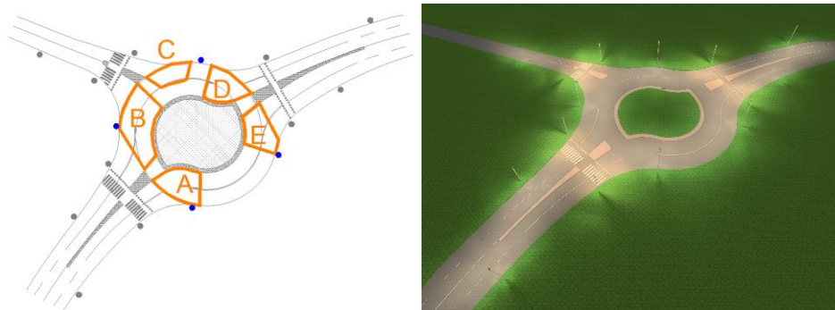
Slika 42: Primer postavitev svetilk za osvetlitev turbo krožnega križišča
