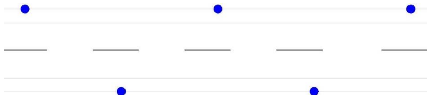
Slika 13: Dvostranska zamaknjena razporeditev svetilk
