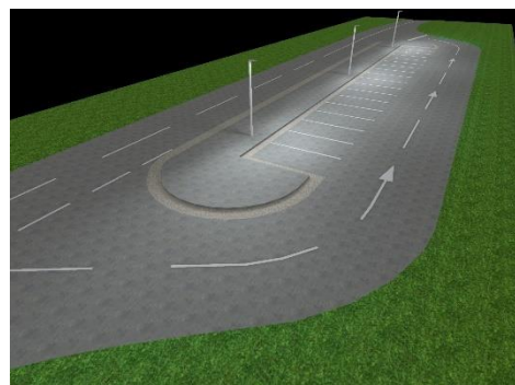
Slika 32: Primer postavitve svetilk za osvetlitev parkirišča
