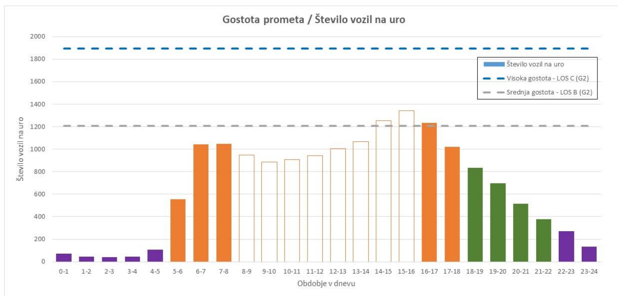
Slika 7: Pregled gostote prometa za obravnavani odsek ceste
