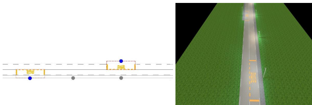
Slika 30: Primer postavitve svetilk za osvetlitev avtobusnih postajališč na neobremenjenem delu ceste z eno svetilko
