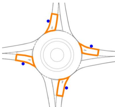
Slika 39: Primer postavitve svetilk za osvetlitev krožnega križišča brez prehodov za pešce
