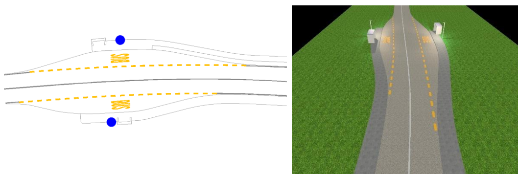
Slika 31: Primer postavitve svetilk za osvetlitev nasproti ležečih avtobusnih postajališč izven vozišča ob cesti izven naselja
