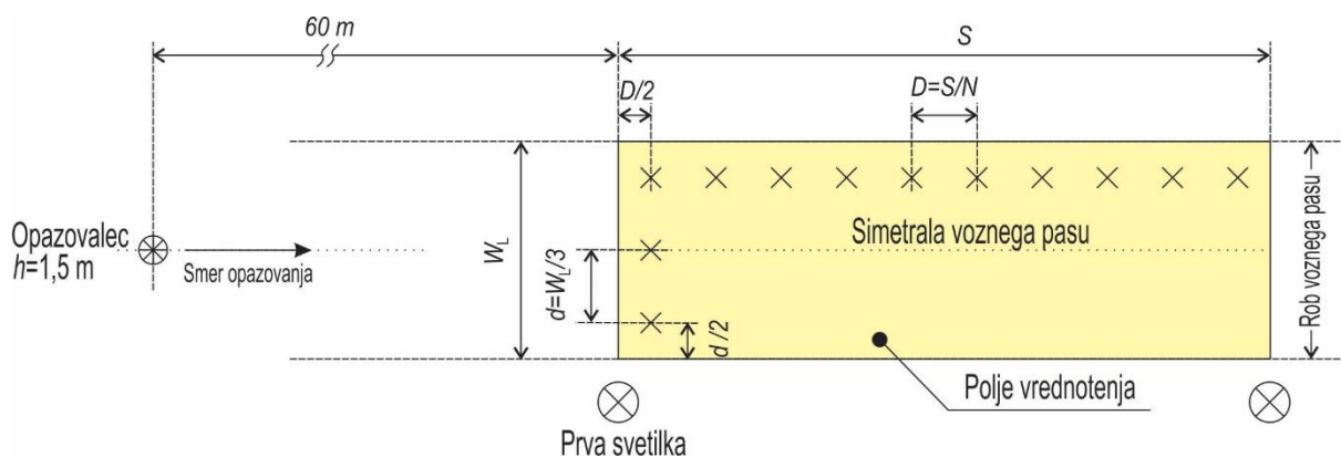
Slika 51: Postavitev merilnih točk na posameznem voznem pasu za meritev svetlosti
