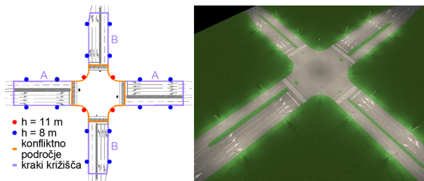
Slika 38: Primer postavitve svetilk za osvetlitev križišča z več kot tremi razvrstilnimi pasovi
