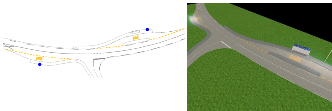
Slika 27: Primer postavitve svetilk za osvetlitev avtobusnih postajališč izven naselja z deniveliranim otokom
