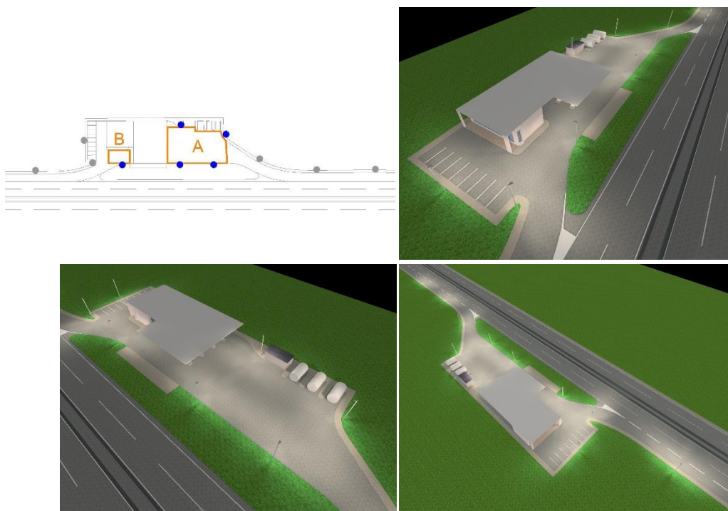
Slika 34: Primer postavitve svetilk za osvetlitev oskrbne postaje
