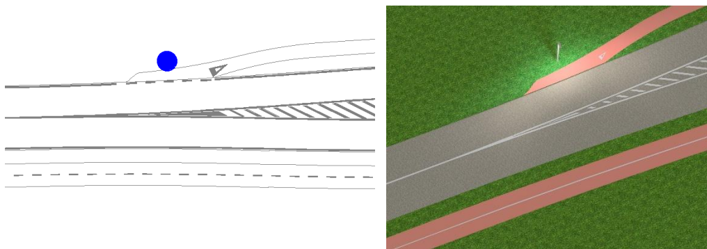
Slika 48: Primer postavitve svetilk za osvetlitev območja, kjer se prepletata motorni in kolesarski promet
