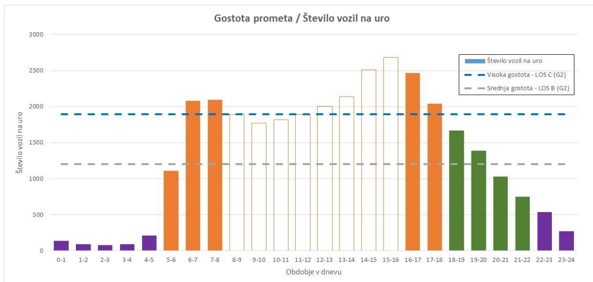
Slika 11: Primer porazdelitve števila vozil v dnevu
