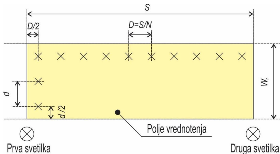
Slika 52: Merilna mreža pri meritvi osvetljenosti
