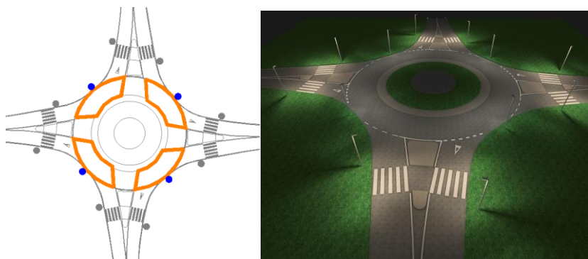
Slika 40: Primer postavitve svetilk za osvetlitev krožnega križišča s samostojnimi prehodi za pešce
