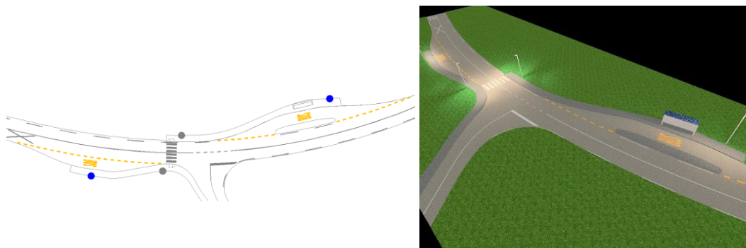
Slika 28: Primer postavitve svetilk za osvetlitev avtobusnih postajališč izven naselja z deniveliranim otokom in prehodom za pešce med njima
