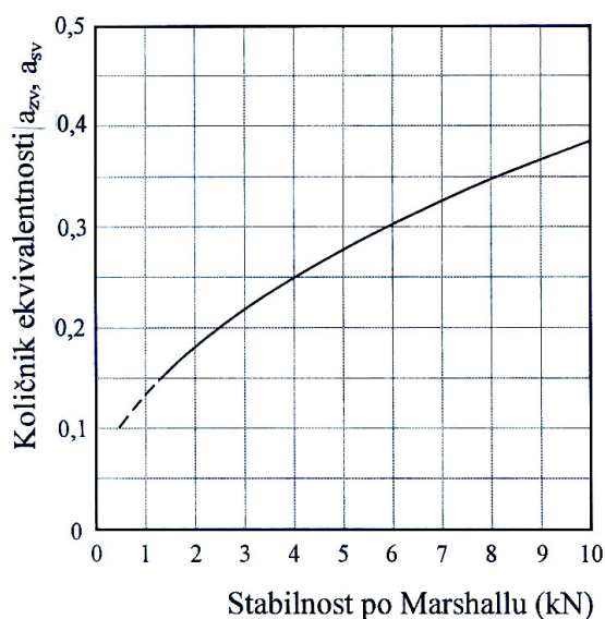
Slika 3: Količniki ekvivalentnosti za bituminizirani prodec in zmes kamnitih zrn, stabilizirano z bitumnom
