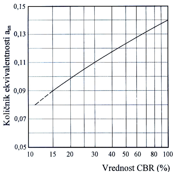
Slika 5: Količniki ekvivalentnosti za nevezano zmes kamnitih zrn (drobljenec, prodec)
