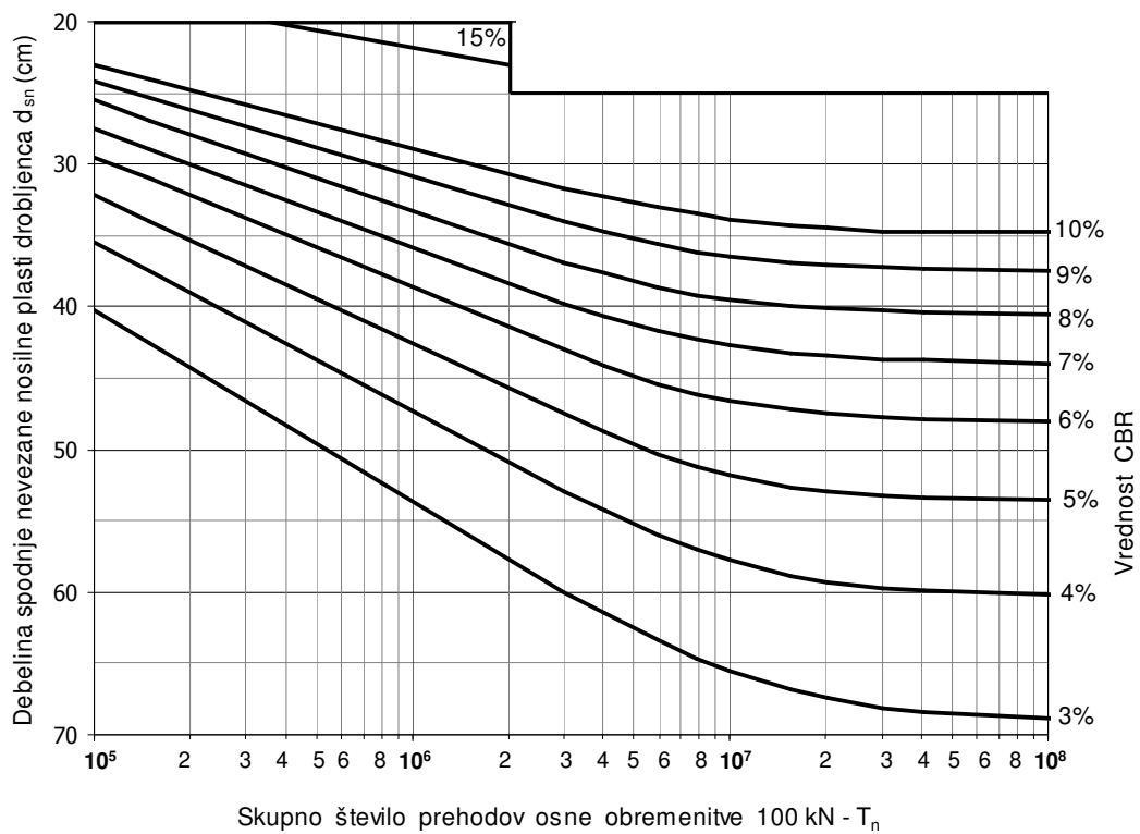
Slika 9: Diagram za določitev dimenzij osnovnih plasti novih asfaltnih voziščnih konstrukcij
