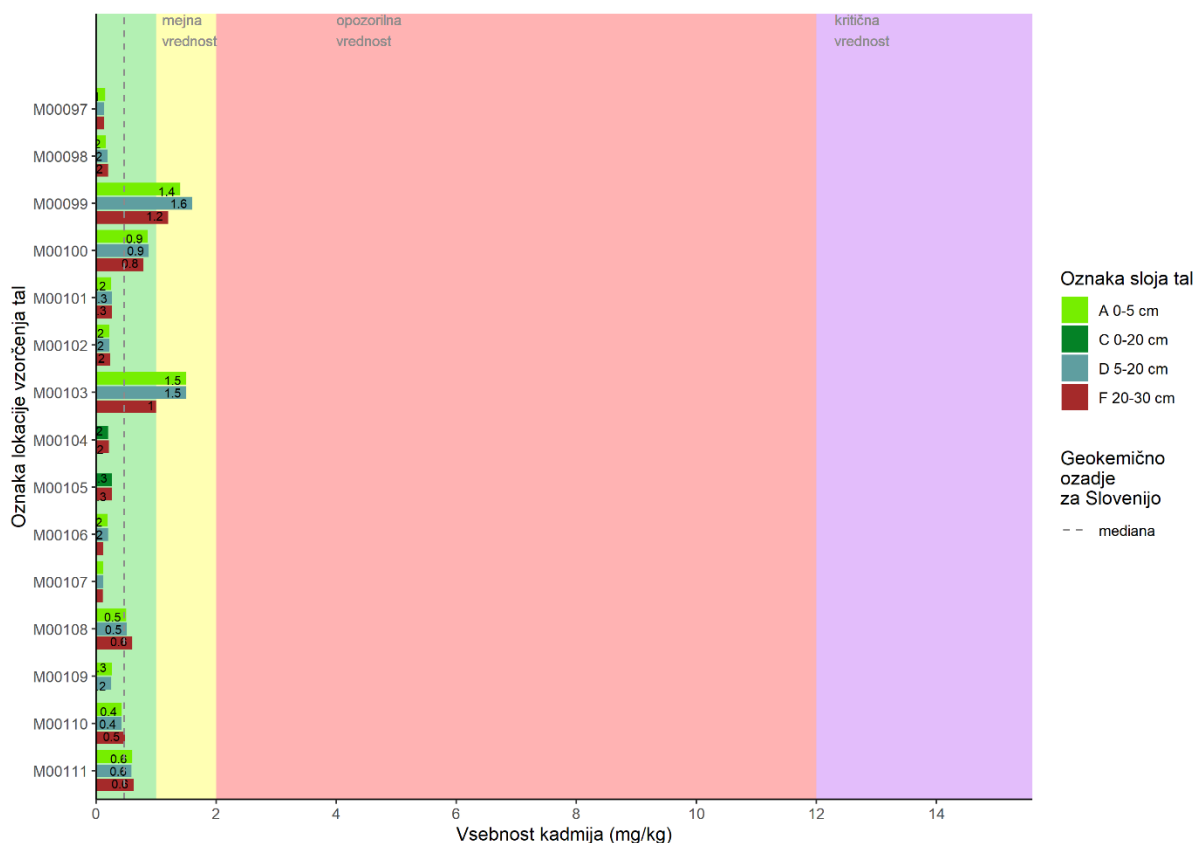
Slika 9: Izmerjene vsebnosti kadmija (mg/kg) v talnih vzorcih različnih slojev vzorčnih mest v MKT24.
