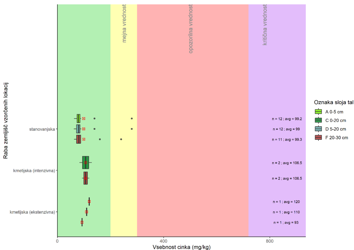
Slika 18: Vsebnost cinka (mg/kg) v talnih vzorcih različnih slojev na preiskovanih rabah tal v MKT24.
