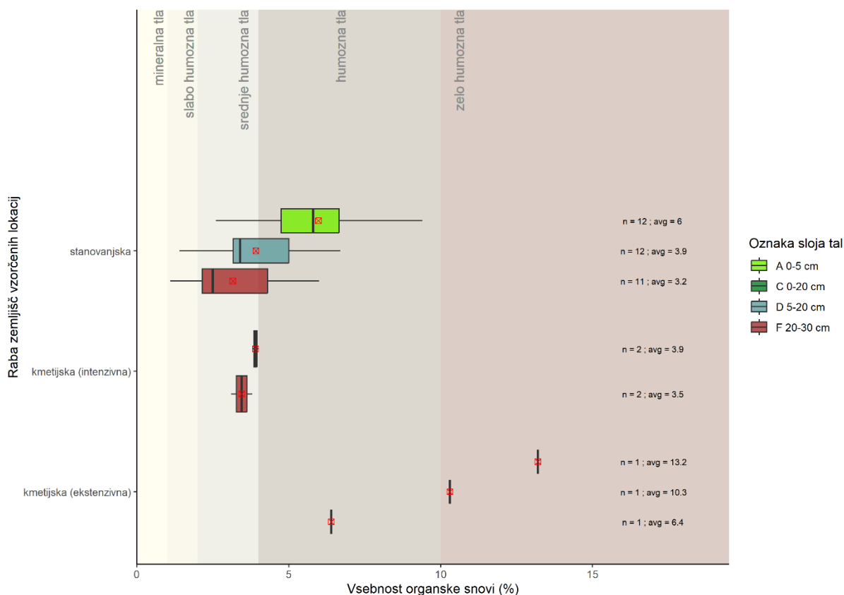
Slika 6: Vsebnost organske snovi (v %) v talnih vzorcih različnih slojev na preiskovanih rabah tal v MKT24.
