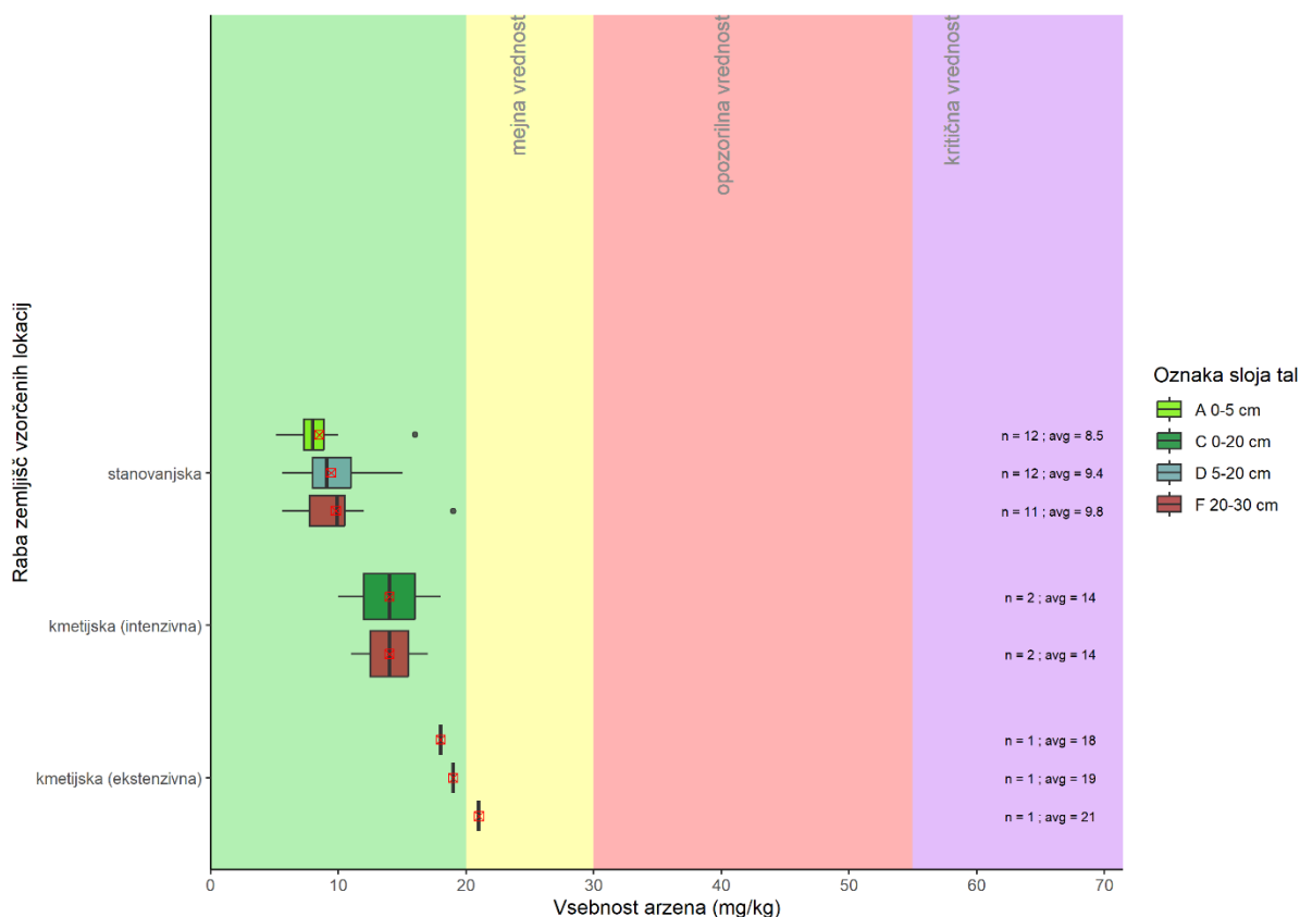
Slika 20: Vsebnost arzena (mg/kg) v talnih vzorcih različnih slojev na preiskovanih rabah tal v MKT24.
