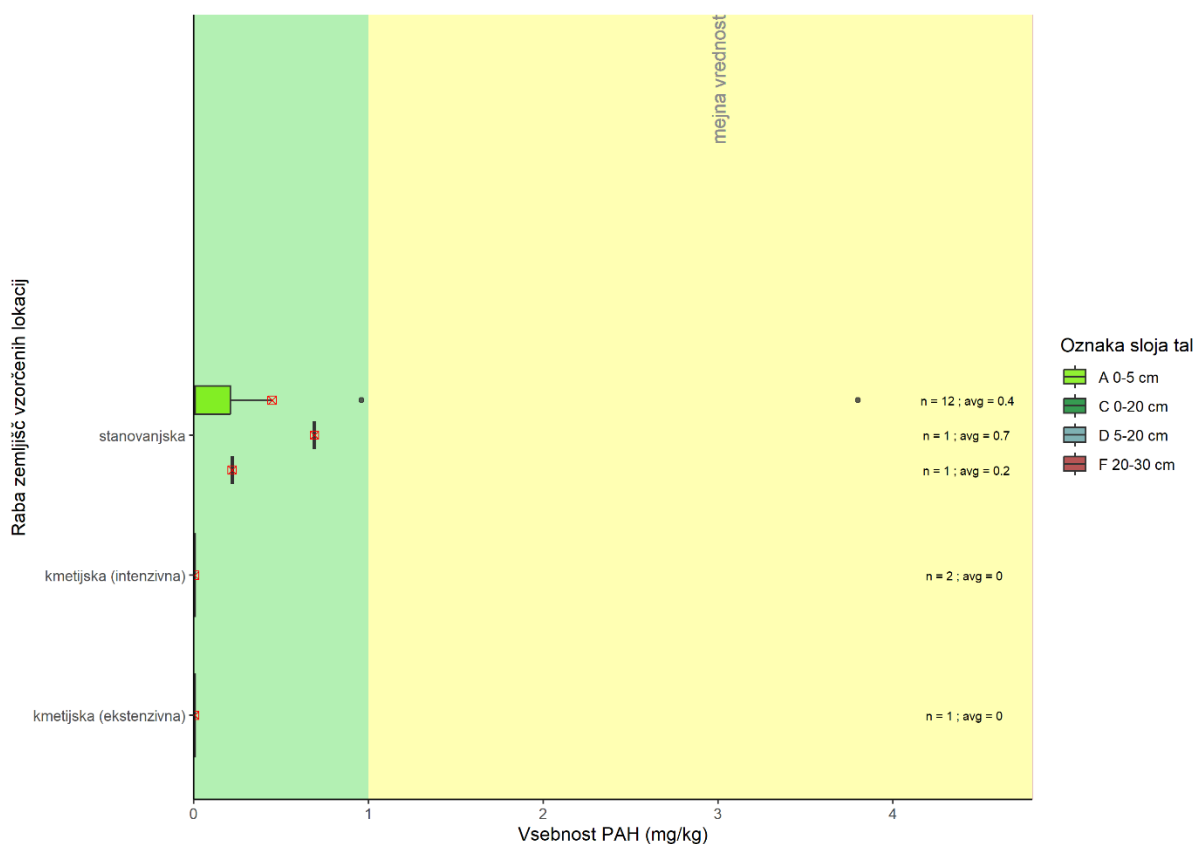
Slika 22: Vsebnost PAH (mg/kg) v talnih vzorcih različnih slojev na preiskovanih rabah tal v MKT24.
