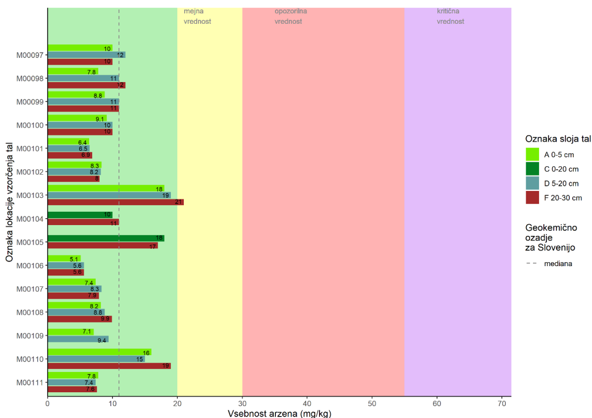
Slika 19: Izmerjene vsebnosti arzena (mg/kg) v talnih vzorcih različnih slojev vzorčnih mest v MKT24.
