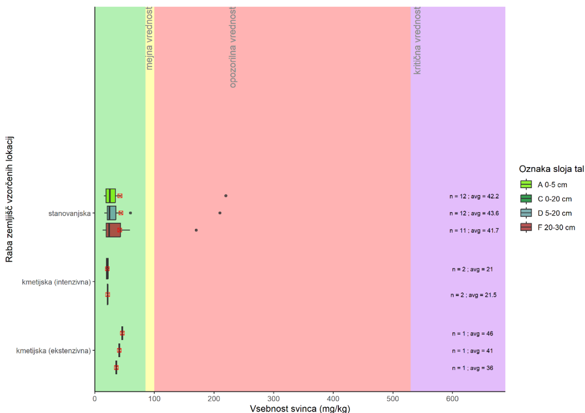
Slika 16: Vsebnost svine (mg/kg) v talnih vzorcih različnih slojev na preiskovanih rabah tal v MKT24.
