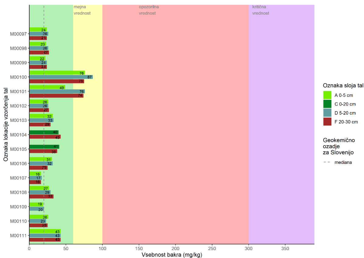
Slika 11: Izmerjene vsebnosti bakra (mg/kg) v talnih vzorcih različnih slojev vzorčnih mest v MKT24.
