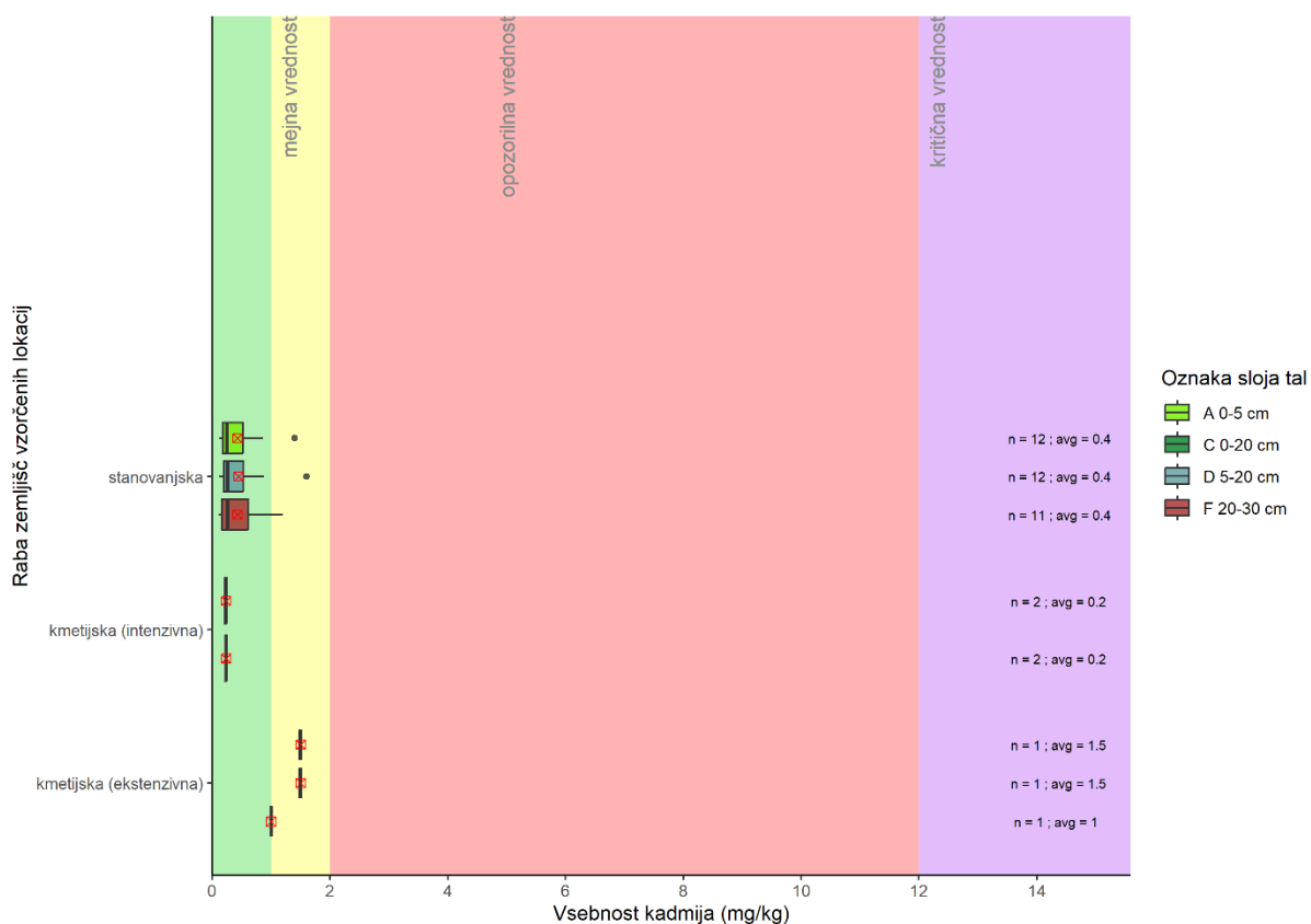
Slika 10: Vsebnost kadmija (mg/kg) v talnih vzorcih različnih slojev na preiskovanih rabah tal v MKT24.
