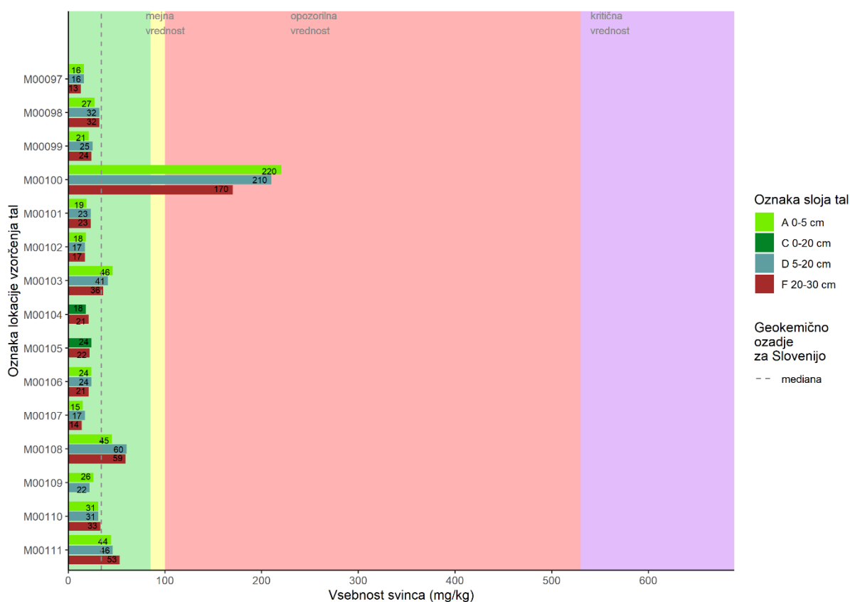
Slika 15: Izmerjene vsebnosti svinca (mg/kg) v talnih vzorcih različnih slojev vzorčnih mest v MKT24.
