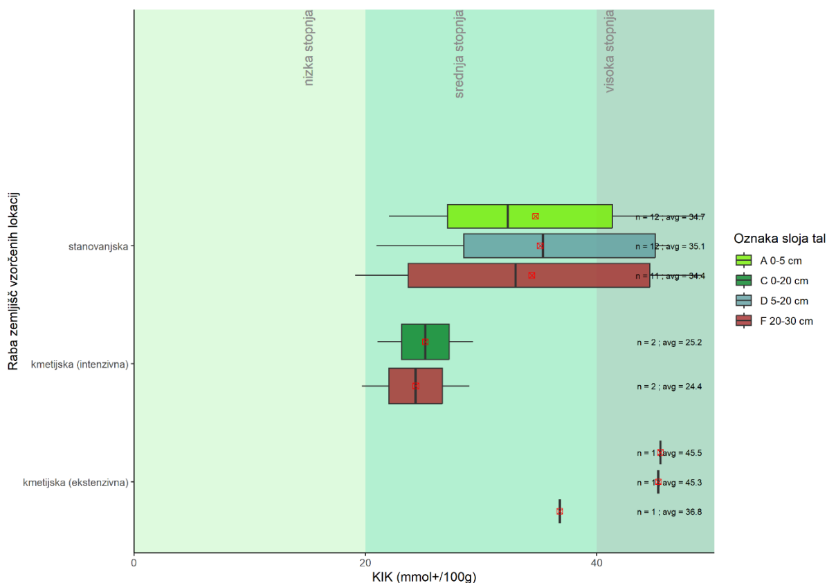
Slika 8: Kationska izmenjalna kapaciteta tal (mmol+/100g) v talnih vzorcih različnih slojev na preiskovanih rabah tal v MKT24.
