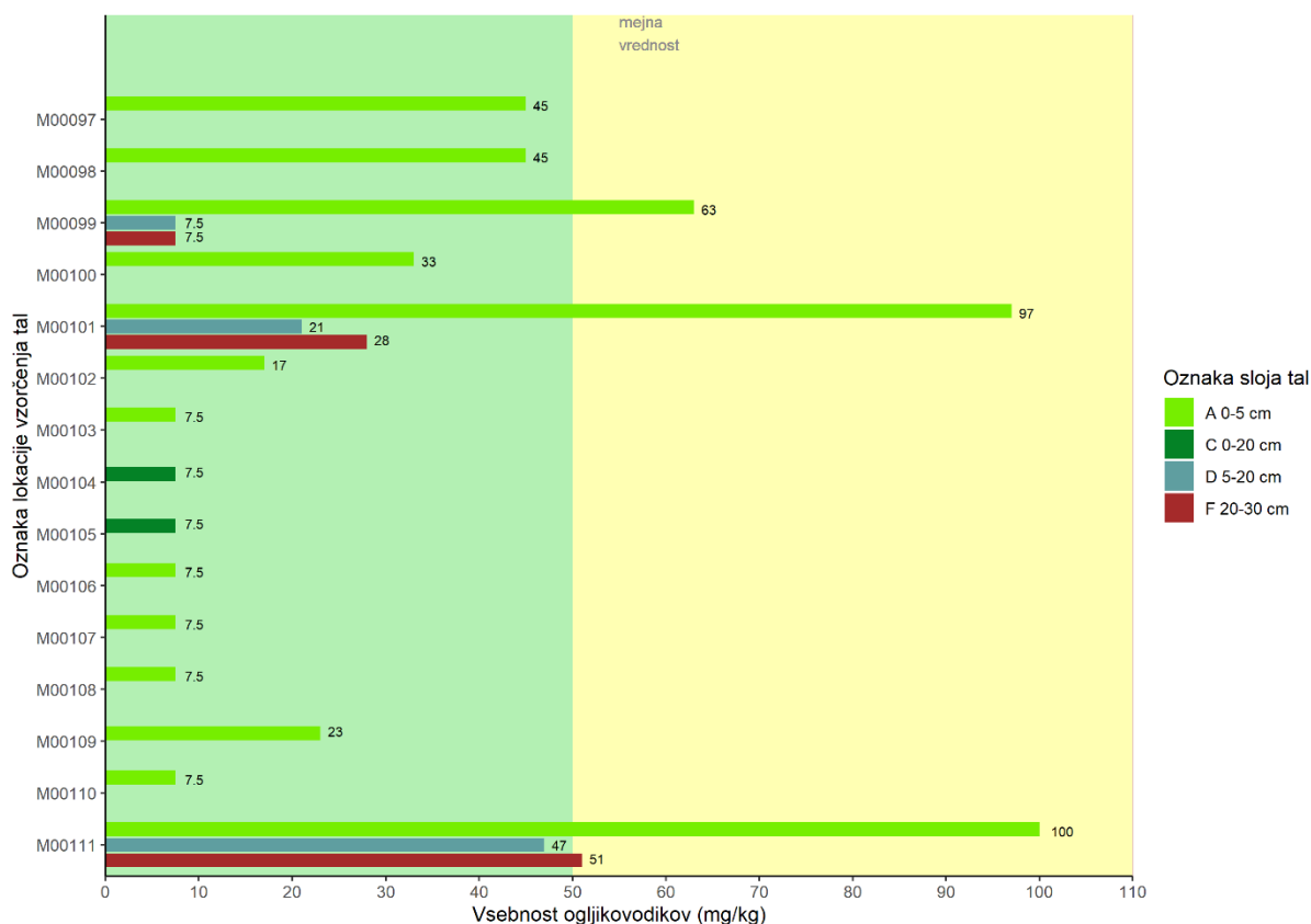
Slika 23: Izmerjene vsebnosti ogljikovodikov C 10 -C 40 (mg/kg) v talnih vzorcih različnih slojev vzorčnih mest v MKT24.
