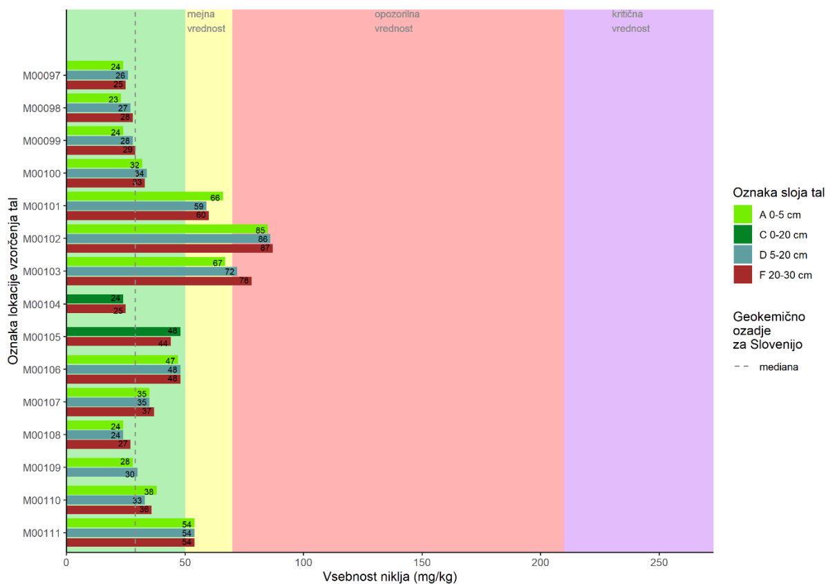
Slika 13: Izmerjene vsebnosti niklja (mg/kg) v talnih vzorcih različnih slojev vzorčnih mest v MKT24.
