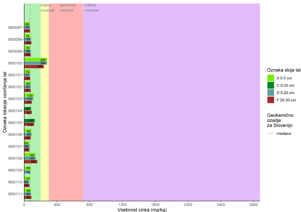
Slika 17: Izmerjene vsebnosti cinka (mg/kg) v talnih vzorcih različnih slojev vzorčnih mest v MKT24.
