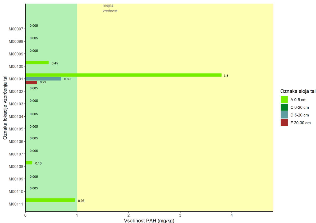
Slika 21: Izmerjene vsebnosti PAH (mg/kg) v talnih vzorcih različnih slojev vzorčnih mest v MKT24.
