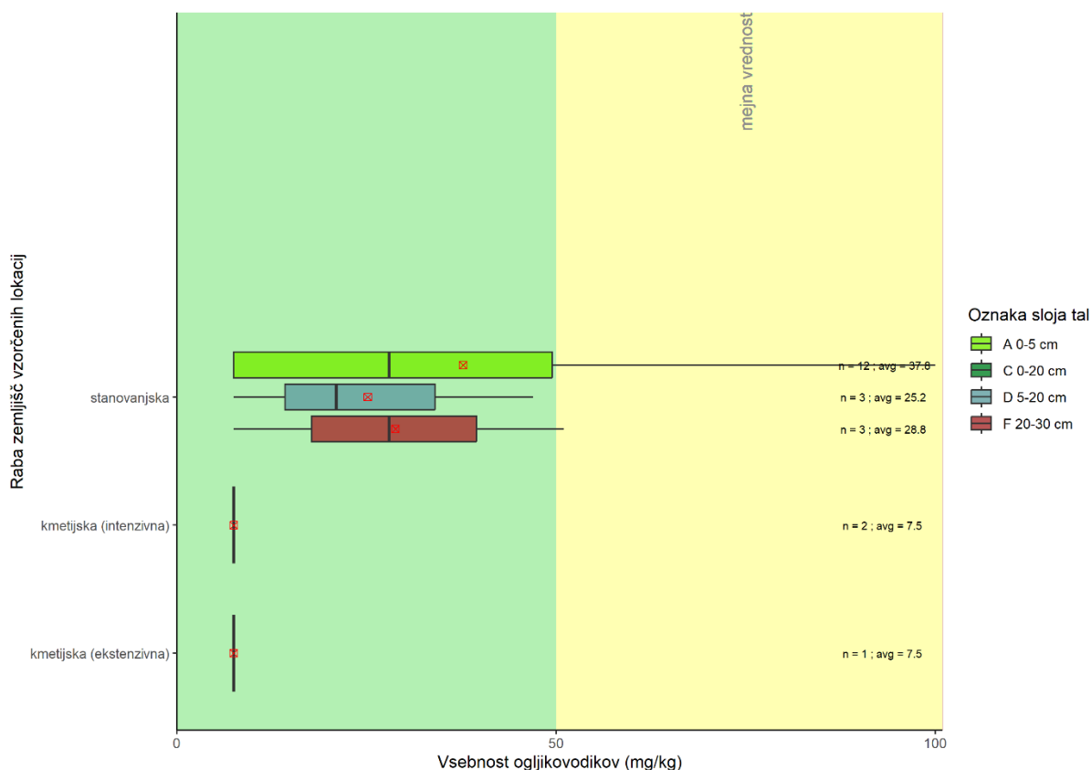
Slika 24: Vsebnost ogljikovodikov C_{10}-C_{40} (mg/kg) v talnih vzorcih različnih slojev na preiskovanih rabah tal v MKT24.
