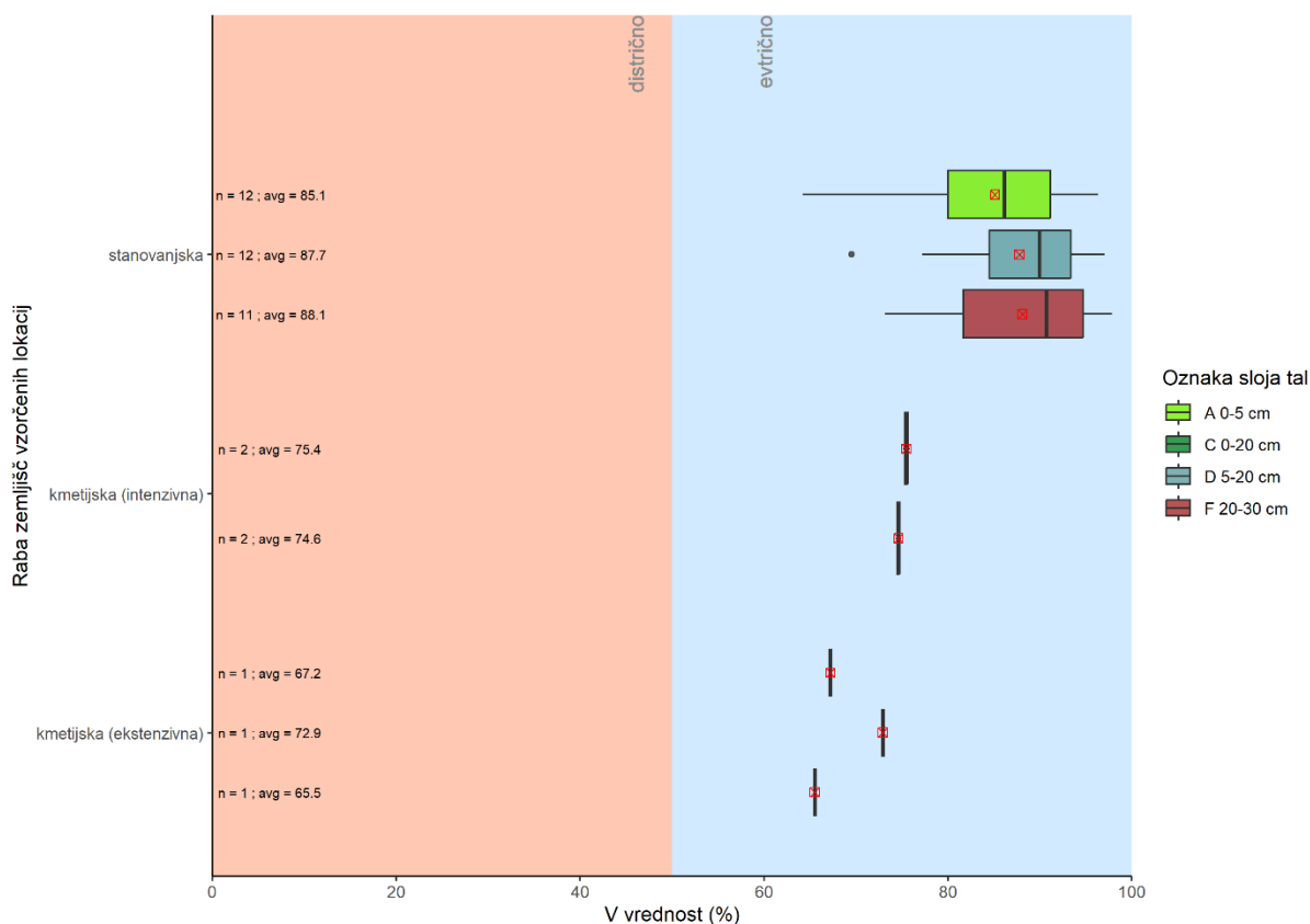
Slika 7: Delež bazičnih kationov (v %) v talnih vzorcih različnih slojev na preiskovanih rabah tal v MKT24.
