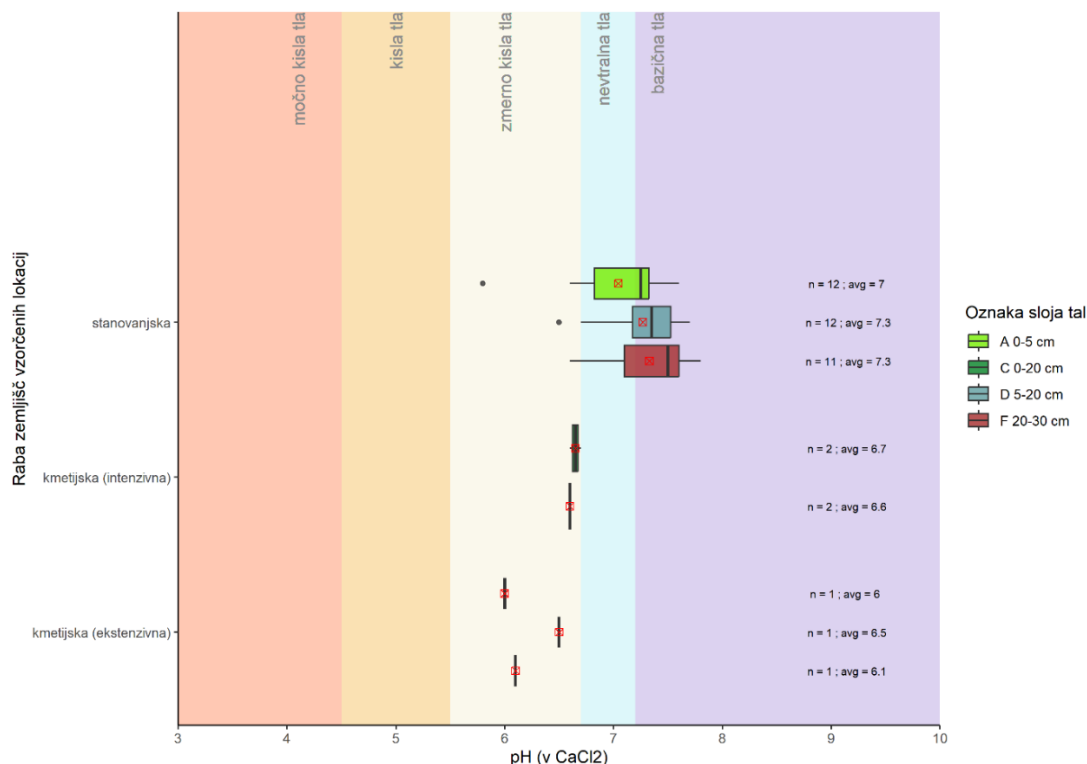
Slika 4: Potencialna kislost (pH) v talnih vzorcih različnih slojev na preiskovanih rabah tal v MKT24.
