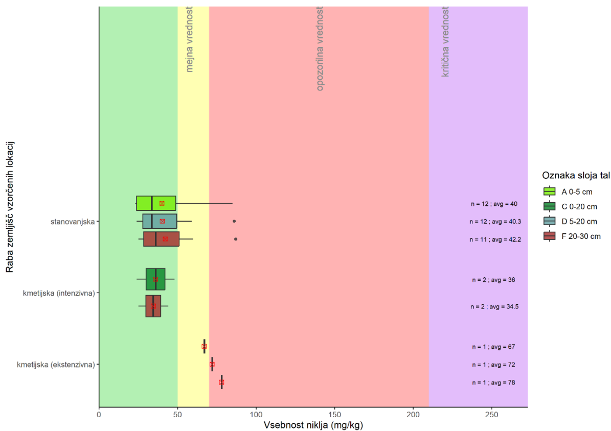
Slika 14: Vsebnost niklja (mg/kg) v talnih vzorcih različnih slojev na preiskovanih rabah tal v MKT24.
