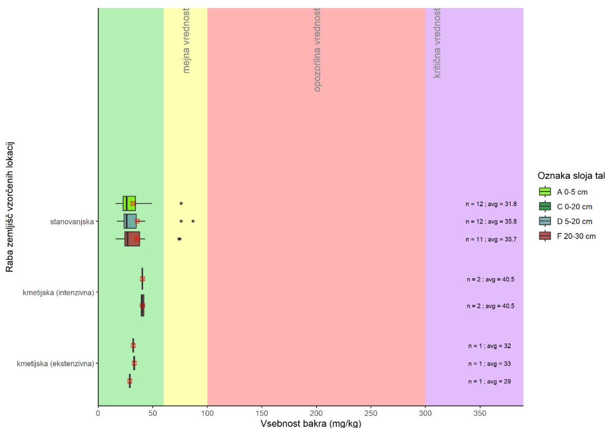
Slika 12: Vsebnost bakra (mg/kg) v talnih vzorcih različnih slojev na preiskovanih rabah tal v MKT24.
