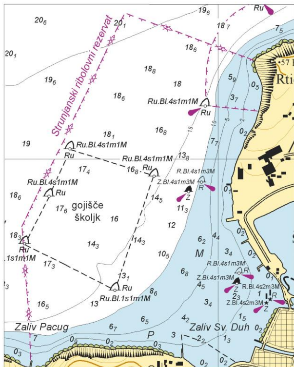
Blok za karto Piranski zaliv 02 Block for Chart Piranski zaliv 02
