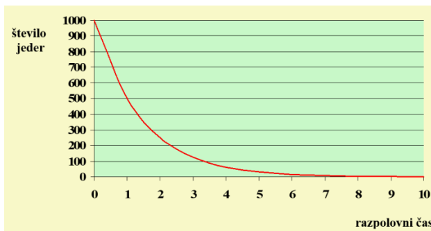
Slika II-3.7: Zmanjševanje števila jeder radioaktivnega izotopa s časom
