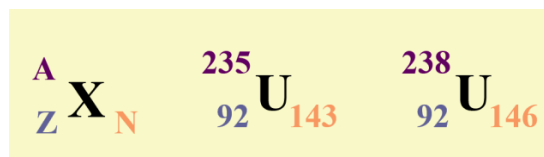
Slika II-3.2: Splošni zapis izotopa
