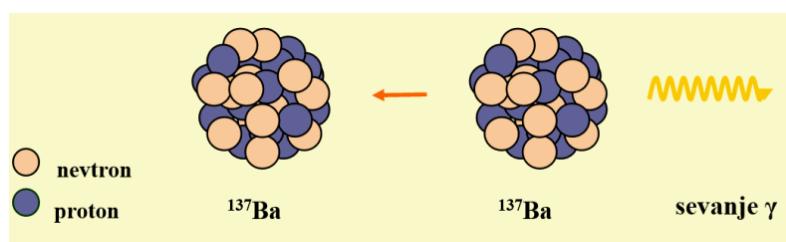
Slika II-3.6: Jedro barija (Ba)
