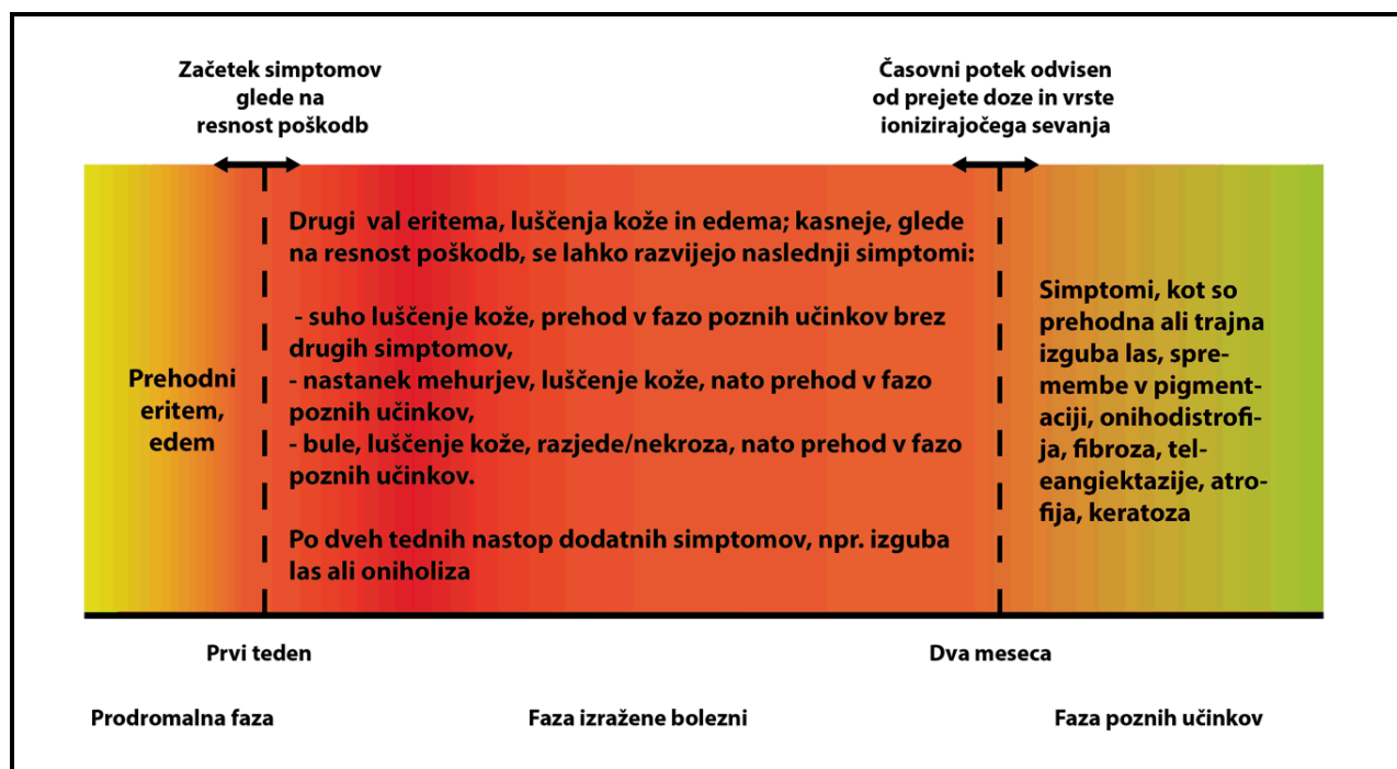
Slika II-3.18: Spremembe pri lokalizirani radiacijski poškodbi glede na čas po poškodbi
