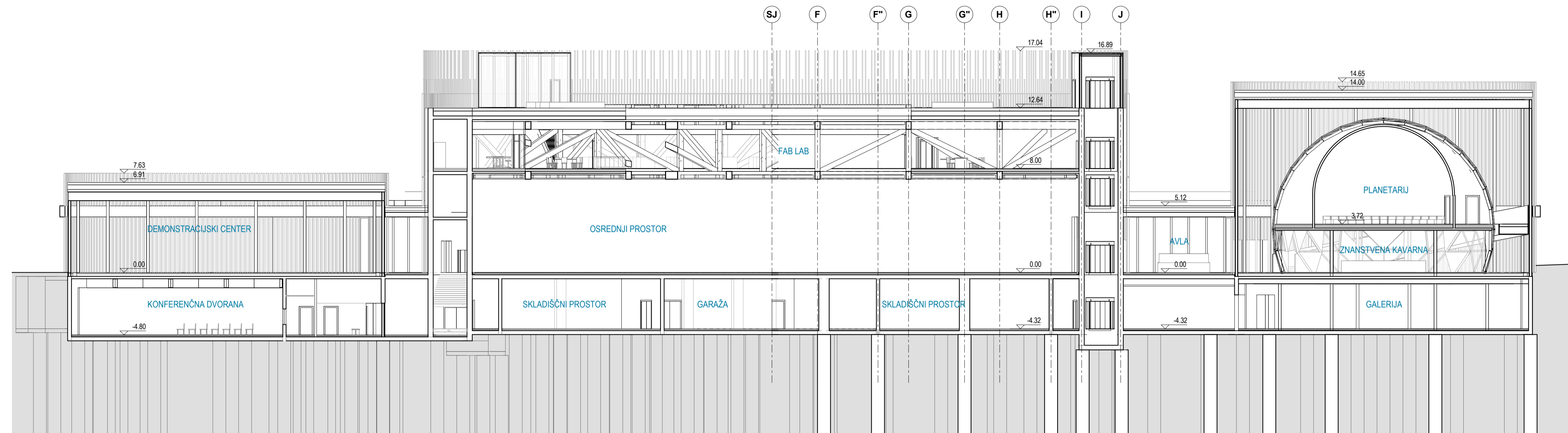
PREREZ AA
