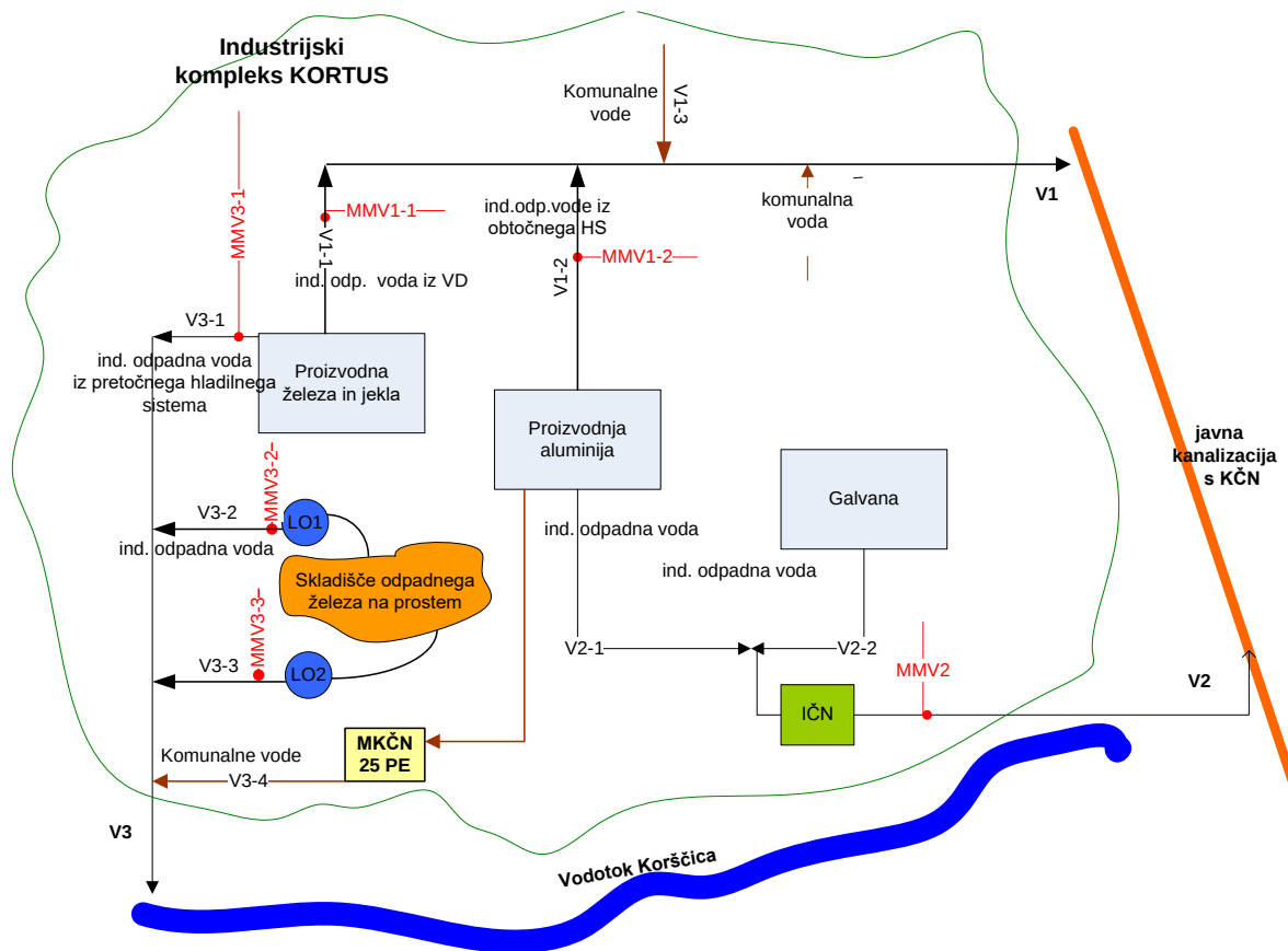
Slika 7: Shematski prikaz (poenostavljen) iztokov/odtokov za podjetje Kortus
