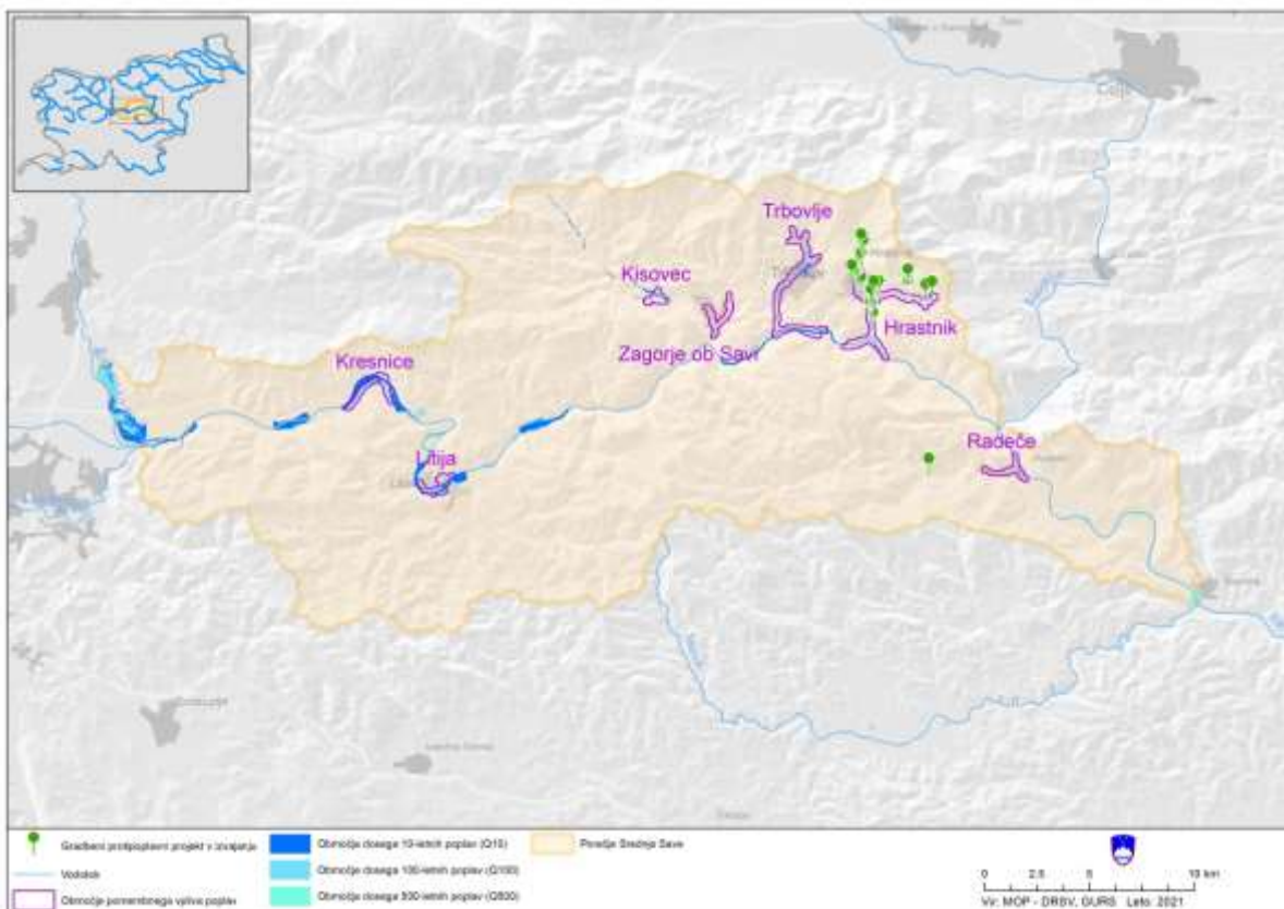
Slika 56. Prikaz porečja Srednje Save z lokacijami gradbenih protipoplavnih ukrepov (informativni prikaz).
