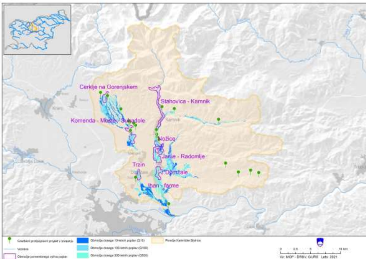
Slika 48. Prikaz porečja Kamniške Bistrice z lokacijami gradbenih protipoplavnih ukrepov (informativni prikaz).
