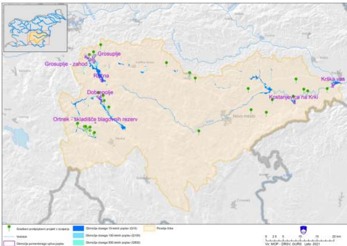
Slika 72. Prikaz porečja Krke z lokacijami gradbenih protipoplavnih ukrepov (informativni prikaz)..
