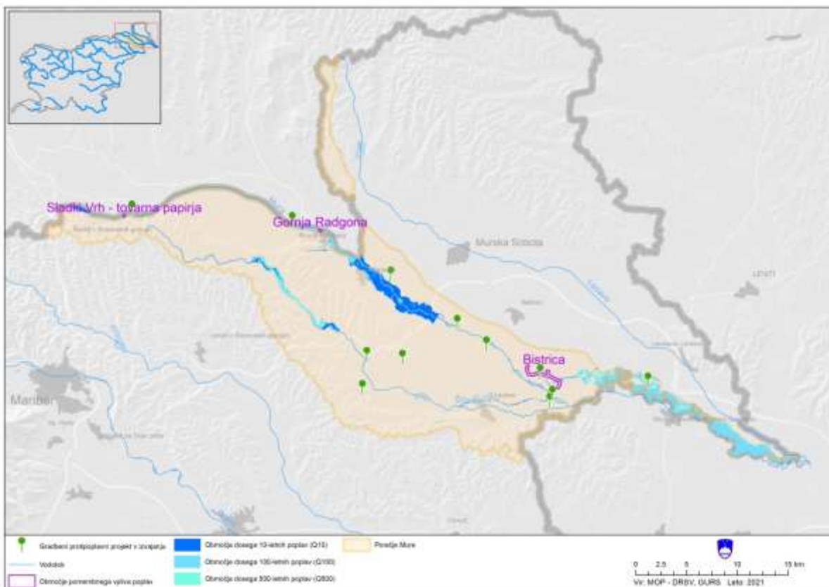
Slika 121. Prikaz porečja Slovenske Mure z lokacijami gradbenih protipoplavnih ukrepov (informativni prikaz).
