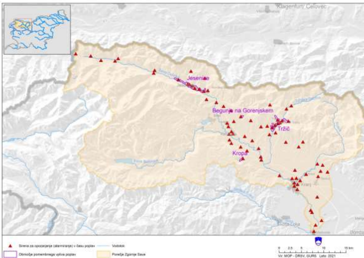
Slika 18. Prikaz porečja Zgornje Save z lokacijami siren za alarmiranje.
