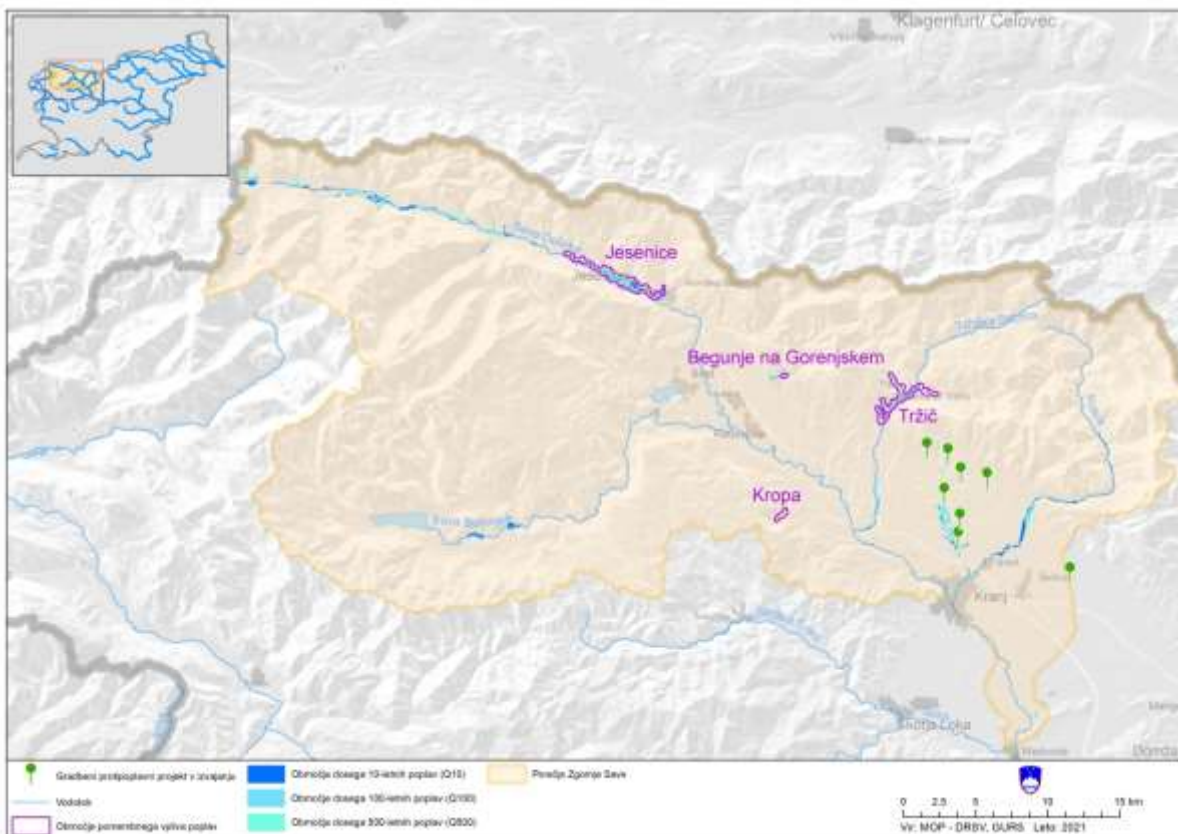
Slika 17. Prikaz porečja Zgornje Save z lokacijami gradbenih protipoplavnih ukrepov (informativni prikaz).
