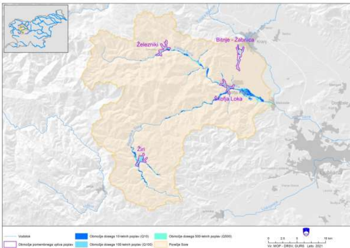
Slika 21. Prikaz poplavne nevarnosti (dosegi 10-, 100- in 500-letnih poplav) na porečju Sore (integralna karta poplavne nevarnosti – iKPN Si). 33
