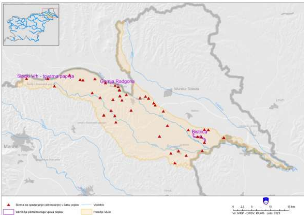
Slika 122. Prikaz porečja Slovenske Mure z lokacijami siren za alarmiranje.
