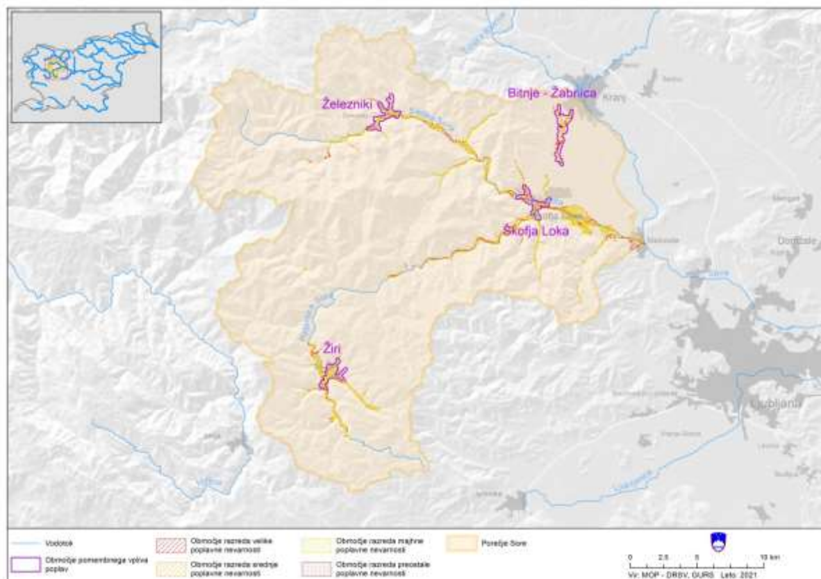
Slika 22. Prikaz razredov poplavne nevarnosti (velika, srednja, majhna in preostala) na porečju Sore.
