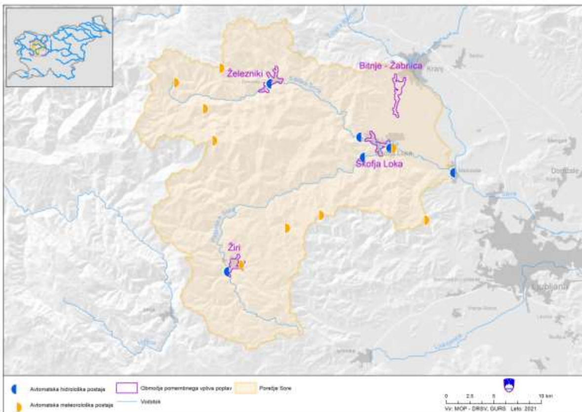
Slika 24. Prikaz lokacij hidrološkega in meteorološkega monitoringa na porečju Sore.
