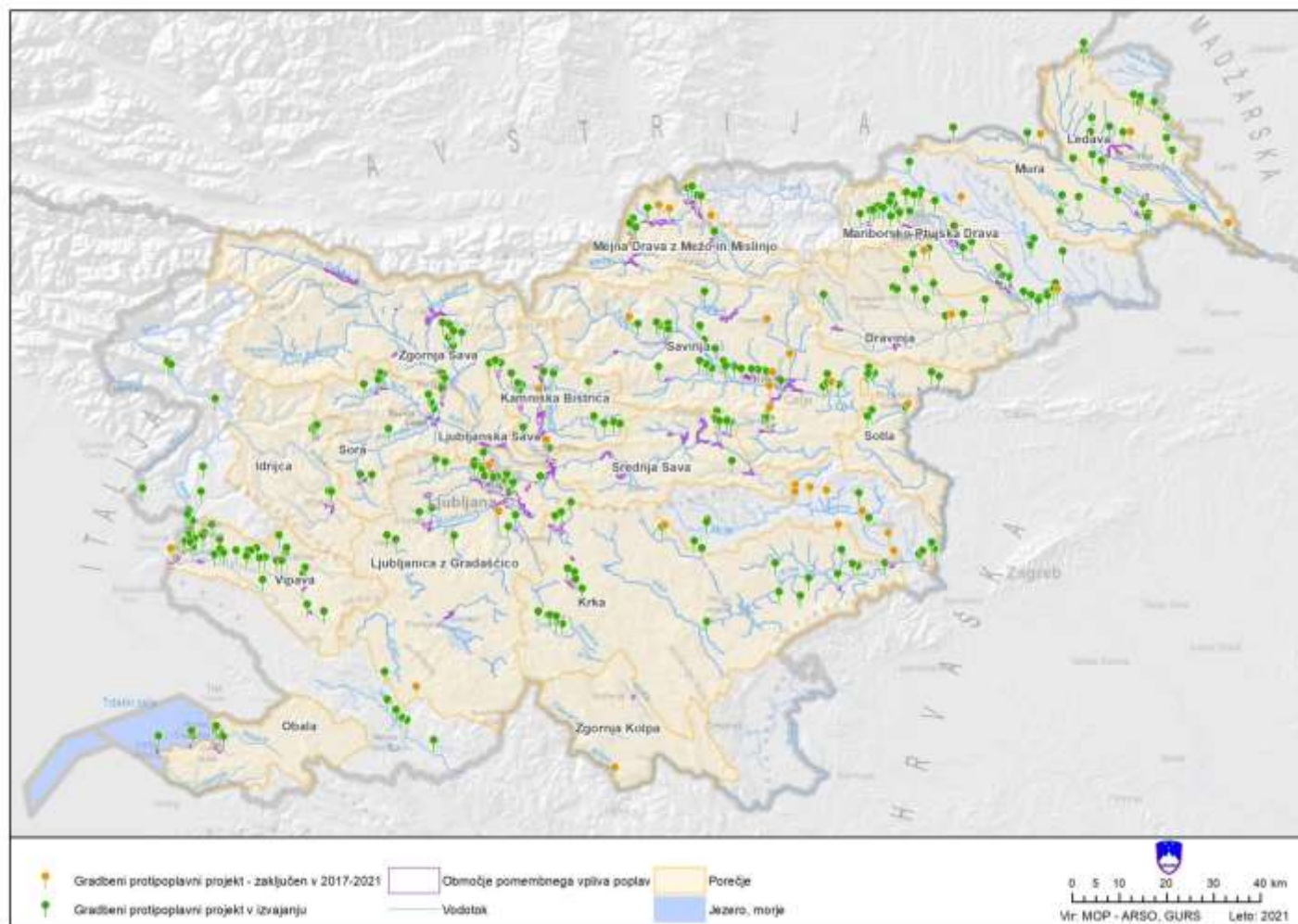
Slika 162. Informativni pregled gradbenih protipoplavnih ukrepov v izvajanju.
