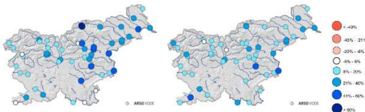
Slika 168. Sprememba letnih konic pretokov v obdobjih 2011–2040 (levo) in 2041–2070 (desno) v primerjavi z obdobjem 1981–2010, po scenariju izpustov toplogrednih plinov RCP4.5
