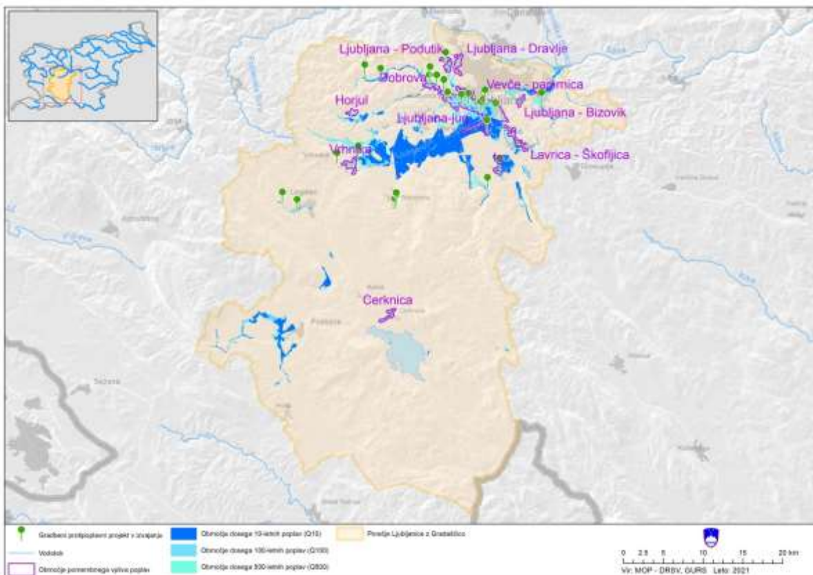
Slika 40. Prikaz porečja Ljubljanice z Gradaščico z lokacijami gradbenih protipoplavnih ukrepov (informativni prikaz).
