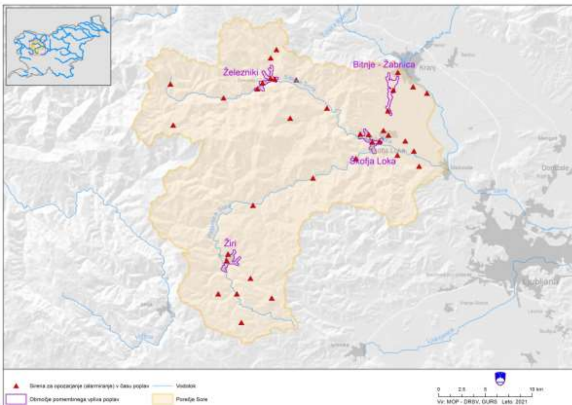
Slika 26. Prikaz porečja Sore z lokacijami siren za alarmiranje.
