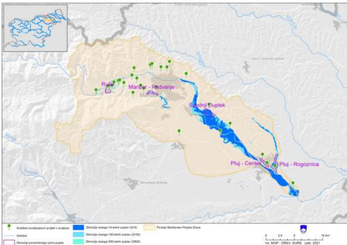
Slika 104. Prikaz porečja Mariborsko-Ptujske Drave z lokacijami gradbenih protipoplavnih ukrepov (informativni prikaz).
