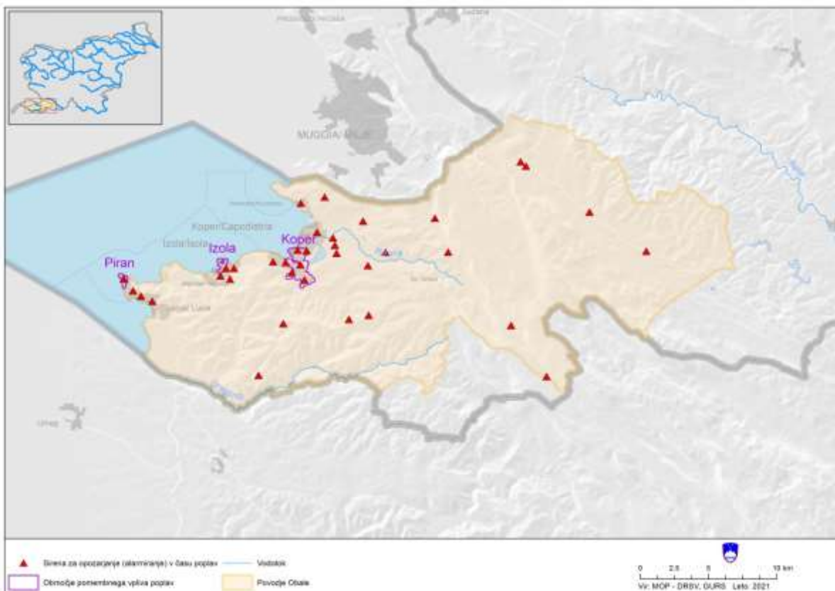
Slika 157. Prikaz porečja Obale z lokacijami siren za alarmiranje.
