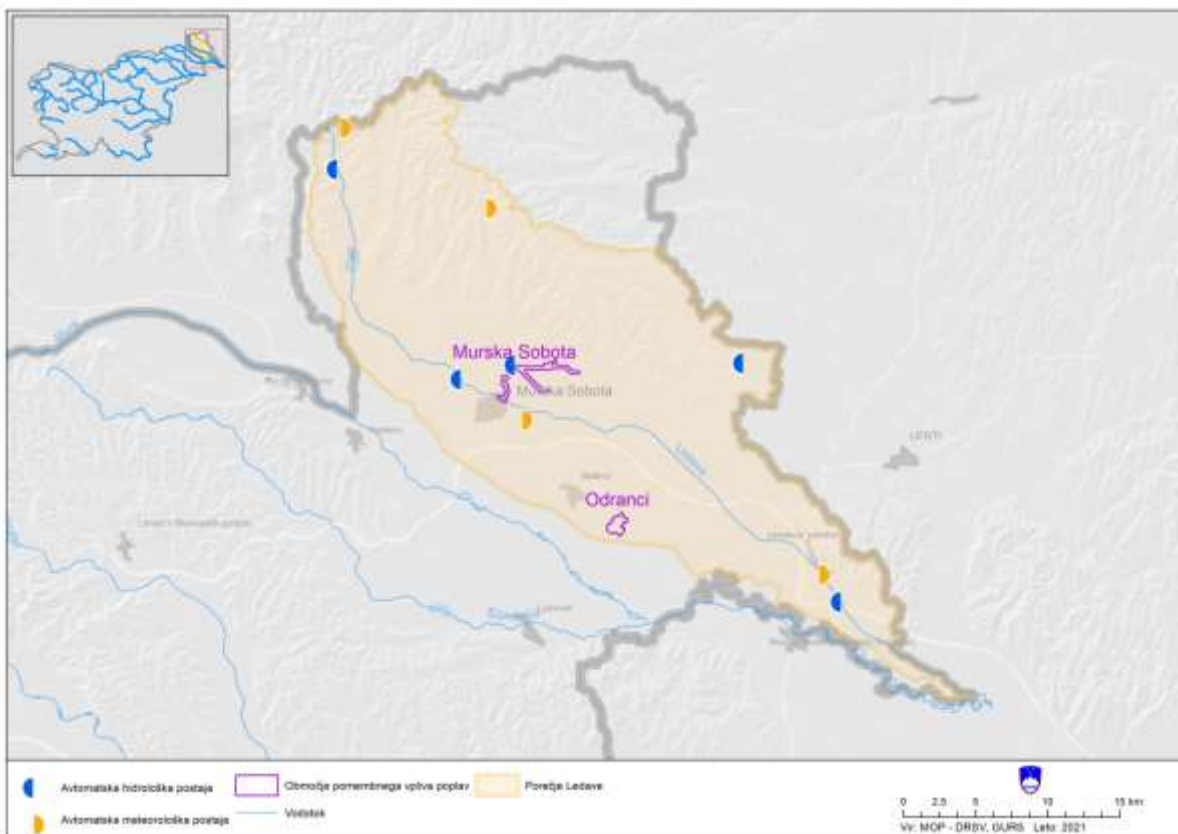
Slika 128. Prikaz lokacij hidrološke in meteorološkega monitoringa na porečju Ledave.
