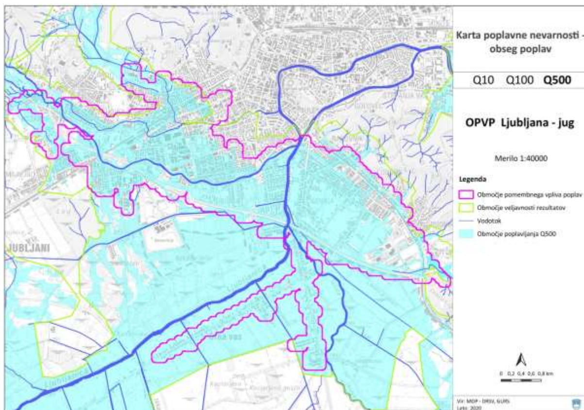
Slika 3. Primer karte poplavne nevarnosti (karta 500-letne poplavne nevarnosti za območje pomembnega vpliva poplav Ljubljana-jug).
