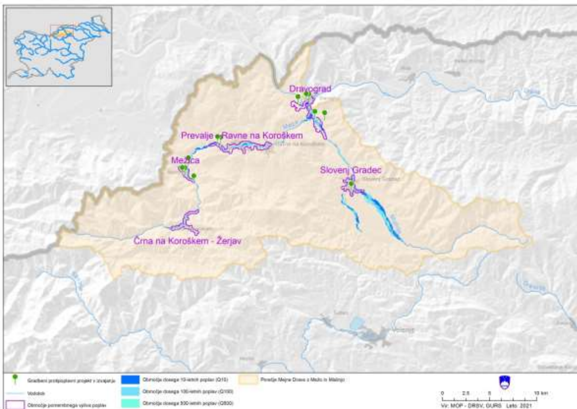
Slika 96. Prikaz porečja Mejne Drave z Mežo in Mislinjo z lokacijami gradbenih protipoplavnih ukrepov (informativni prikaz).
