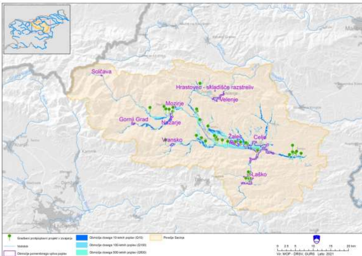
Slika 64. Prikaz porečja Savinje z lokacijami gradbenih protipoplavnih ukrepov (informativni prikaz).
