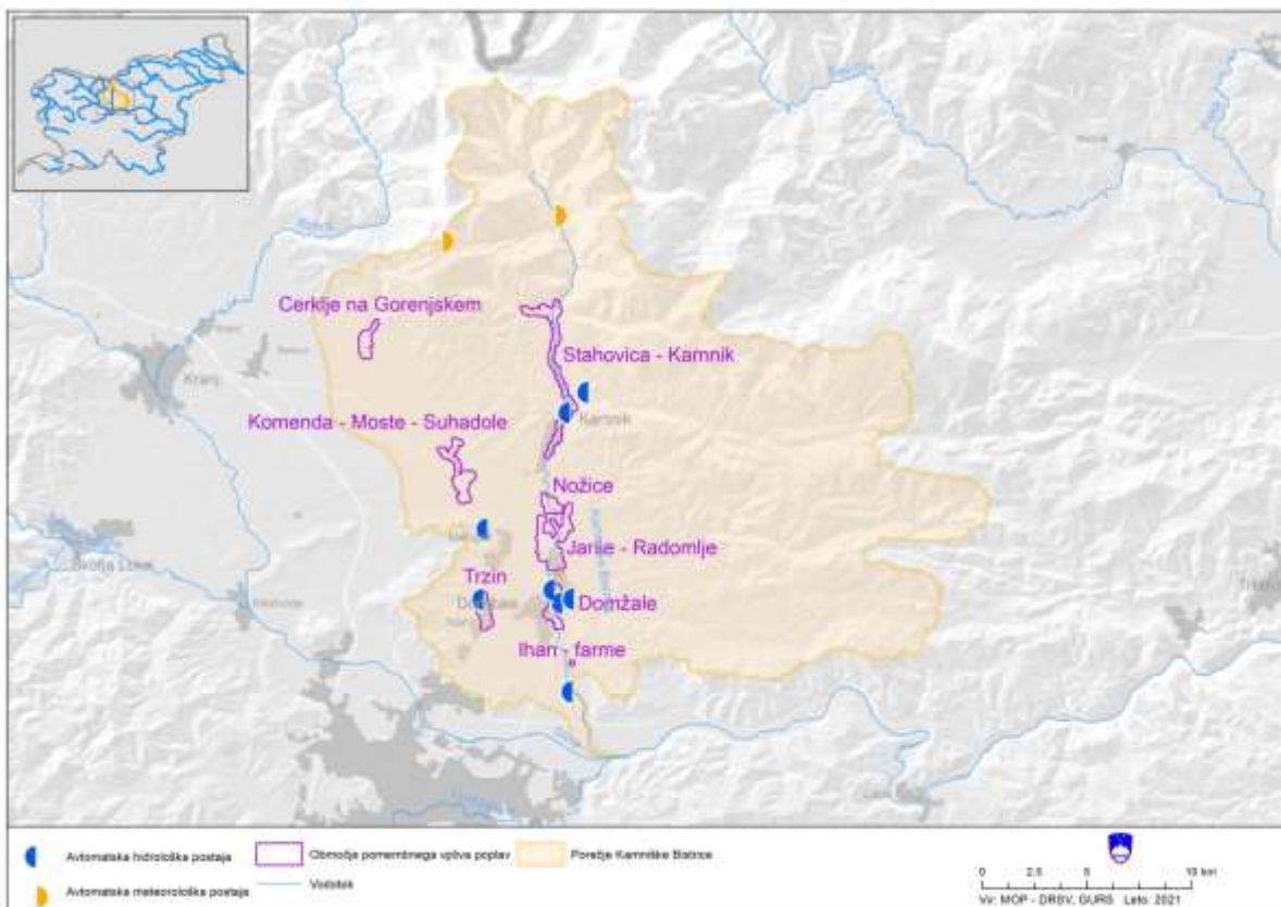
Slika 47. Prikaz lokacij hidrološkega in meteorološkega monitoringa na porečju Kamniške Bistrice.
