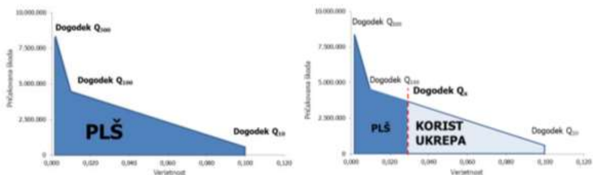
Slika 161. Pričakovana letna škoda pred in po izvedbi ukrepov in koristi ukrepov.
