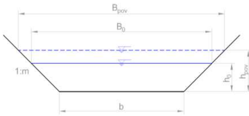
Slika 171. Karakteristični prikaz testnega pretočnega korita
