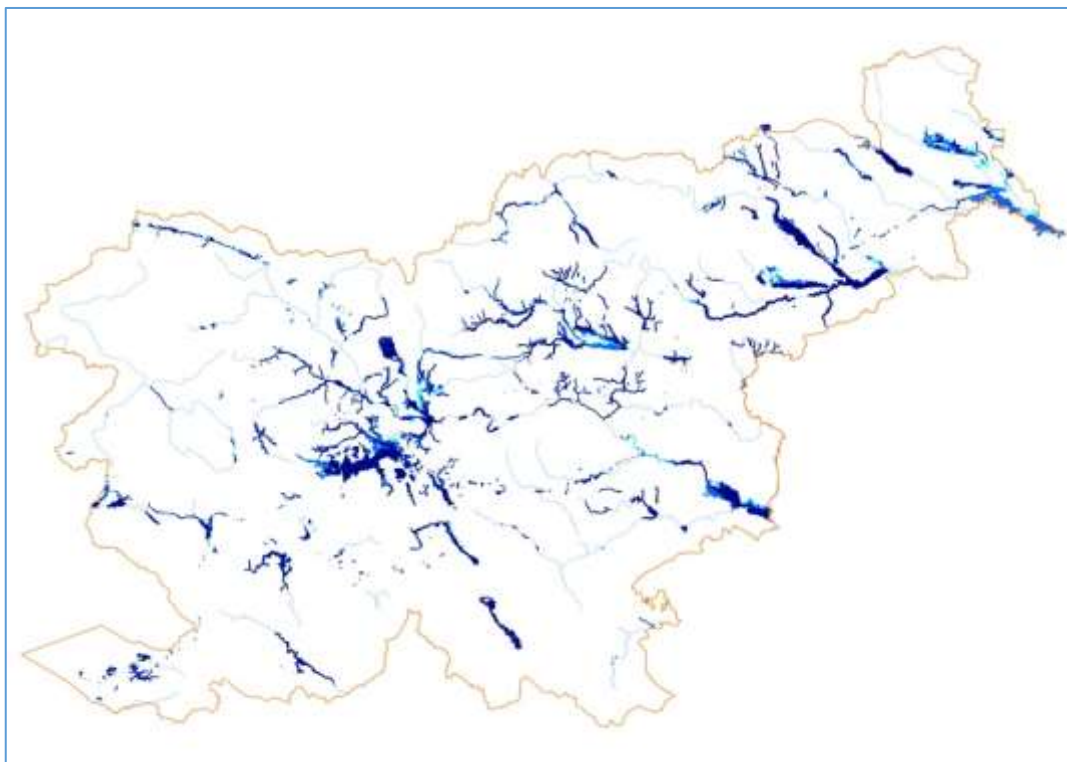
Slika 175. Integralna karta poplavne nevarnosti.
