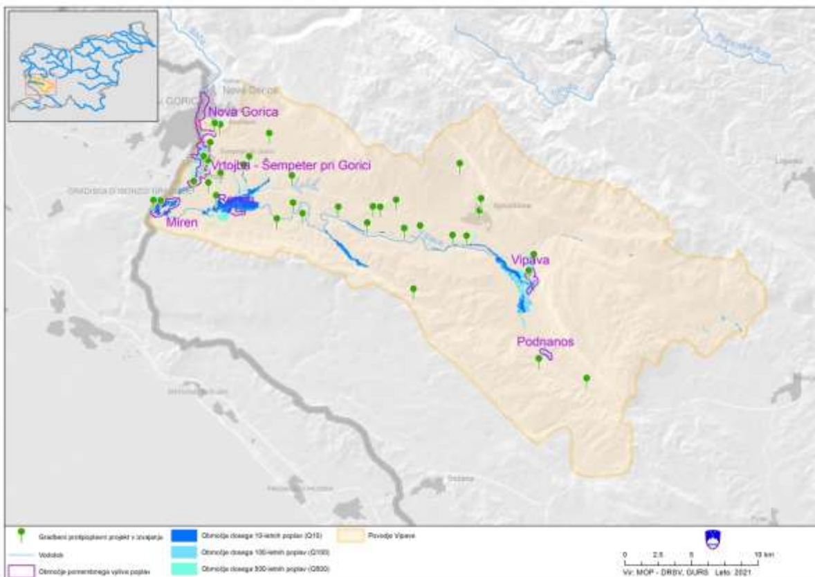
Slika 147. Prikaz porečja Vipave z lokacijami gradbenih protipoplavnih ukrepov (informativni prikaz).
