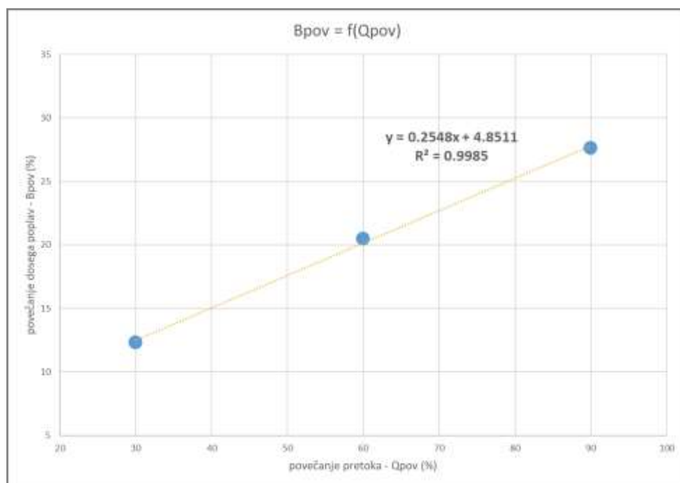
Slika 172. Prikaz odvisnosti povečanja dosega poplav od povečanja pretoka
