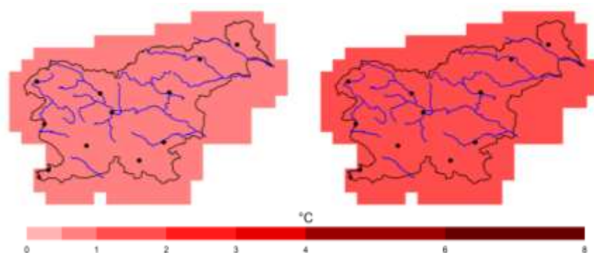
Slika 164. Sprememba temperature zraka v obdobju 2011–2040 (levo) in 2041–2070 (desno) v primerjavi z obdobjem 1981–2010, po scenariju izpustov toplogrednih plinov RCP4.5
