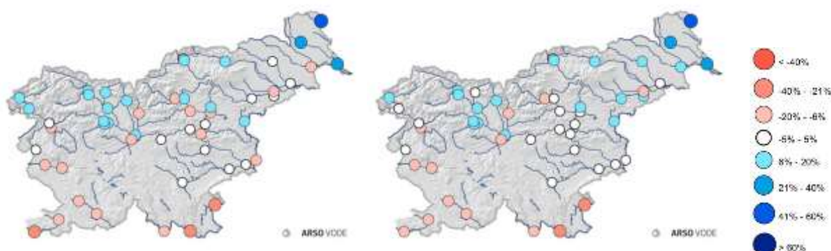
Slika 166. Sprememba srednjih malih letnih pretokov v obdobjih 2011–2040 (levo) in 2041–2070 (desno) v primerjavi z obdobjem 1981–2010, po scenariju izpustov toplogrednih plinov RCP4.5
