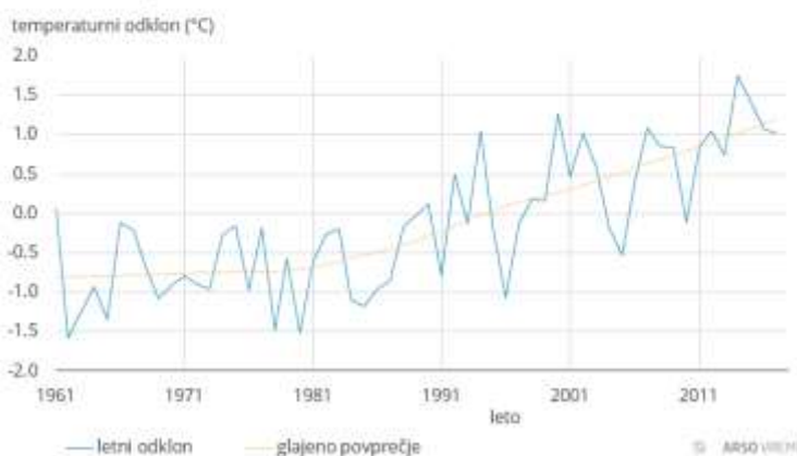
Slika 163. Odklon povprečne temperature zraka od povprečja 1981–2010 na območju Slovenije v času od 1961 do 2017
