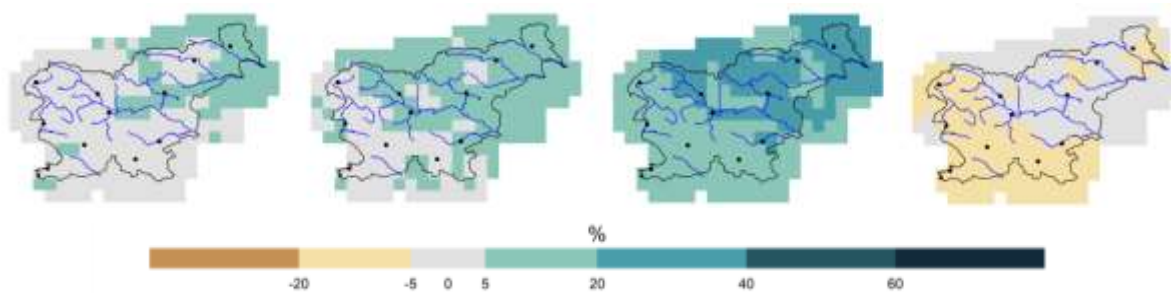
Slika 165. Predvidene spremembe padavin v primerjavi z obdobjem 1981–2010 (od leve proti desni: letne v obdobju 2011–2040, letne v obdobju 2041–2070, zimske v obdobju 2041–2070, poletne v obdobju 2041–2070), po scenariju izpustov toplogrednih plinov RCP4.5
