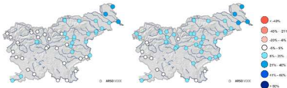
Slika 167. Sprememba srednjih letnih pretokov v obdobjih 2011–2040 (levo) in 2041–2070 (desno) v primerjavi z obdobjem 1981–2010, po scenariju izpustov toplogrednih plinov RCP4.5
