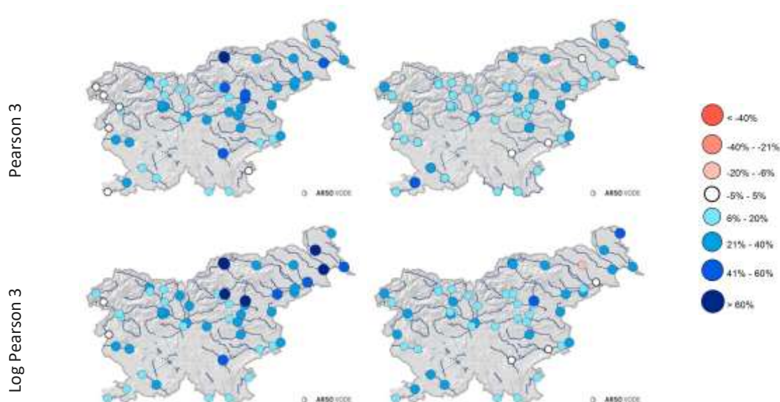
Slika 169. Sprememba pretokov stoletnih (Q100) povratnih dob v obdobjih 2011–2040 (levo) in 2041–2070 (desno) v primerjavi z obdobjem 1981–2010, po scenariju izpustov toplogrednih plinov RCP4.5 za porazdelitvi Pearson 3 (zgoraj) in Log Pearson 3 (spodaj)
