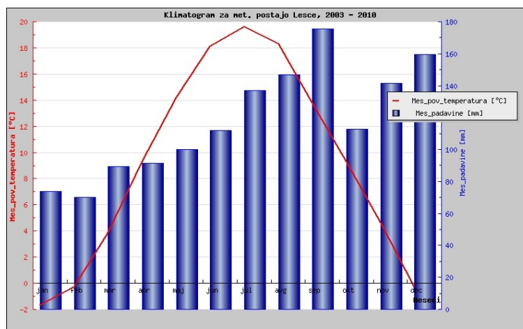
Slika 5 - 1: Klimatogram za opis podnebnih sprememb
