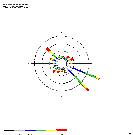
Slika 37 - 2: Vetrovna roža na območju slovenske obale
