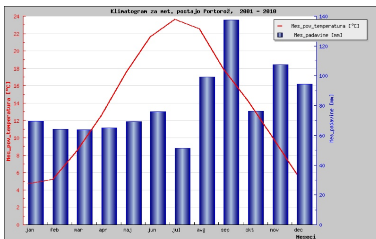
Slika 37 - 1: Klimatogram za opis podnebnih sprememb slovenske obale
