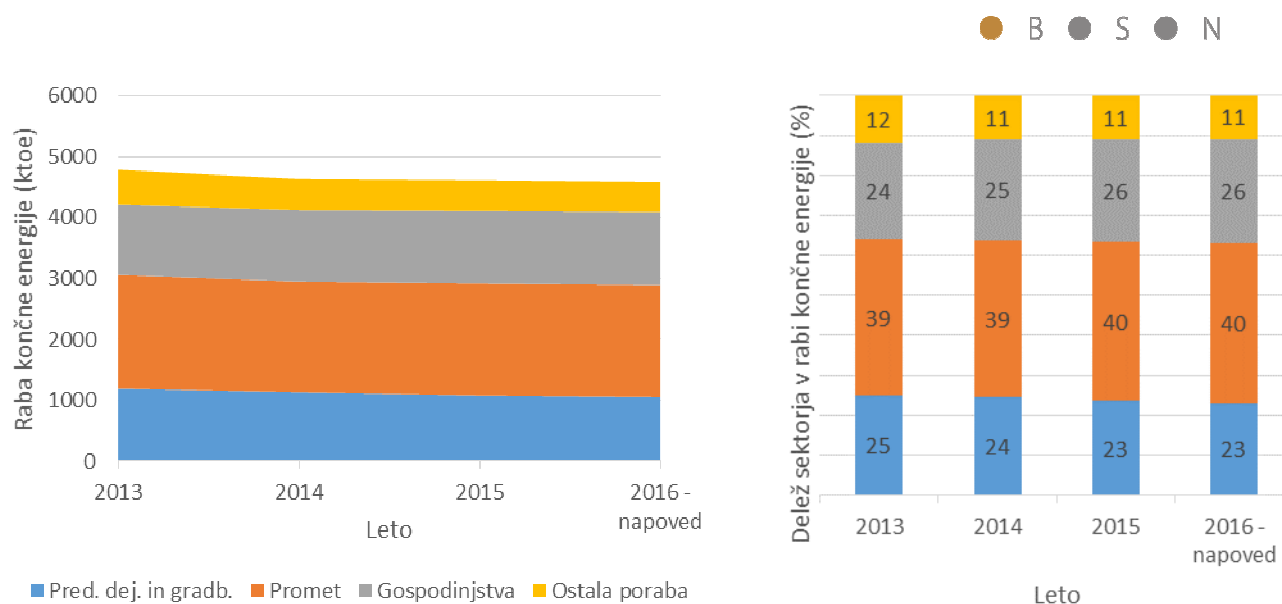
Slika 2: Raba končne energije v obdobju 2013 - 2016, ter delež po sektorjih (vir: EBRŠ, 2015)
