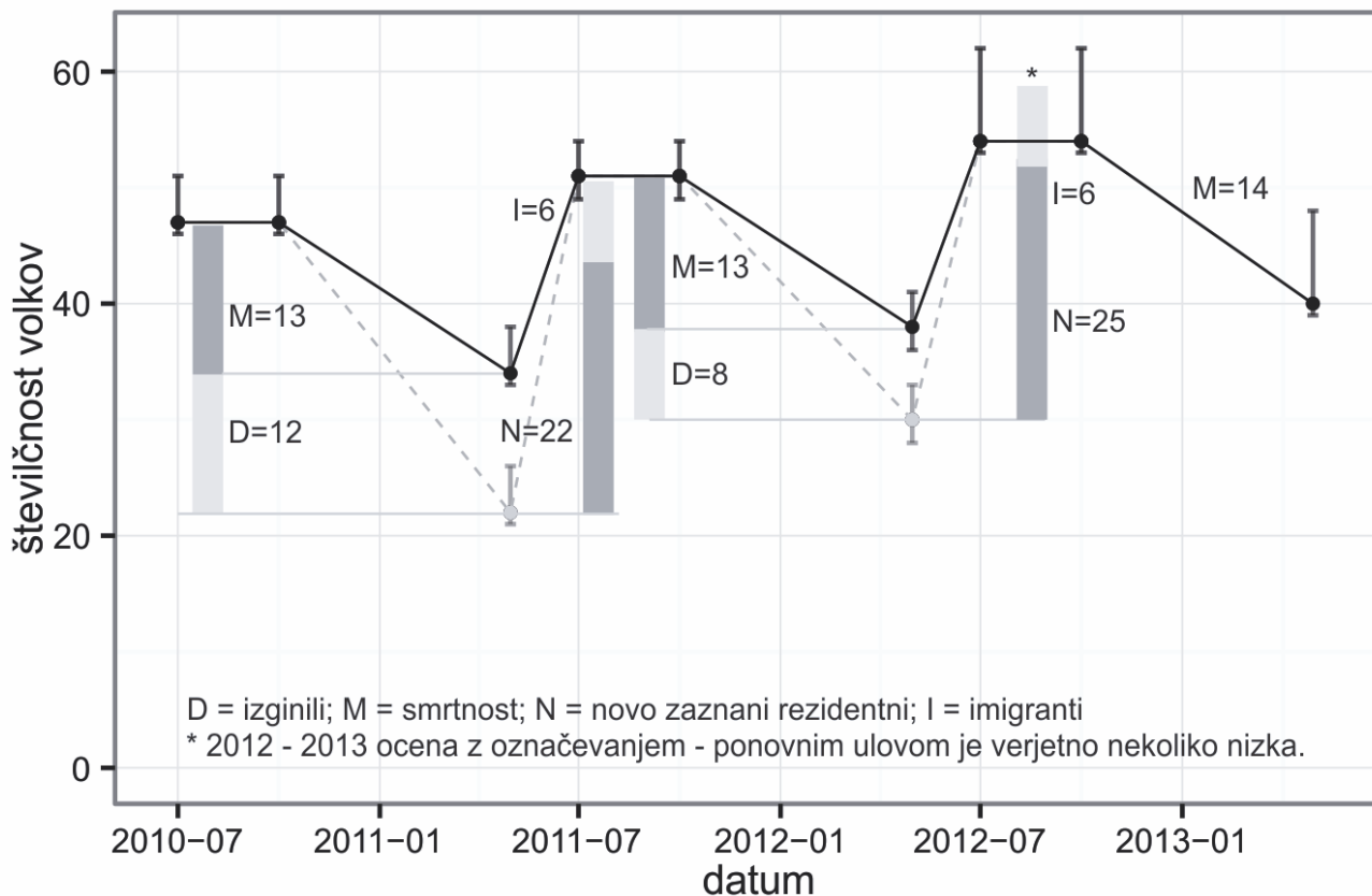
Slika 8: Graf gibanja ocenjene številčnosti volkov za celotno območje vzorčenja (Slovenija + Gorski Kotar, Hrvaška). Letno nihanje populacije je ocenjeno tako, da smo odšteli zaznano smrtnost (polna črta) oziroma »izginule« volkove, ki jih v naslednji sezoni nismo več zaznali (črtkana črta). Glede na to, da smo samo enega volka od 110 najdenih v vzorčenju zaznali prvo in tretjo sezono, drugo pa ne, lahko sklepamo, da je velika večina »izginulih« volkov bodisi umrla ali zapustila območje. Rezidentne volkove in imigrante smo med seboj ločili z analizo starševstva. (Vir: SloWolf).
