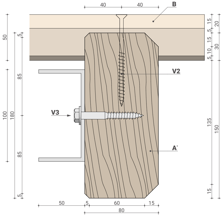
detajl P1, merilo 1:2
