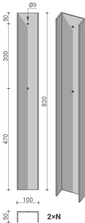
NOGA, merilo 1:10
