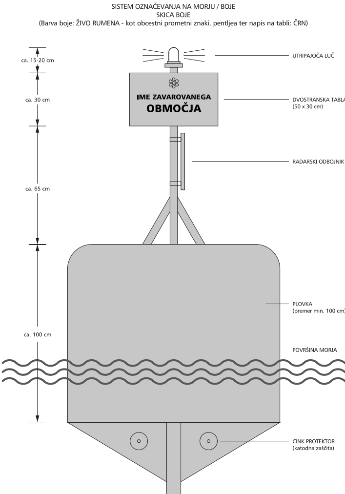
SLIKA V/1
