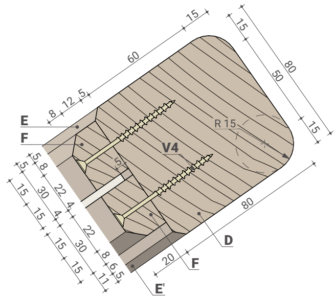
detajl P2, merilo 1:2
