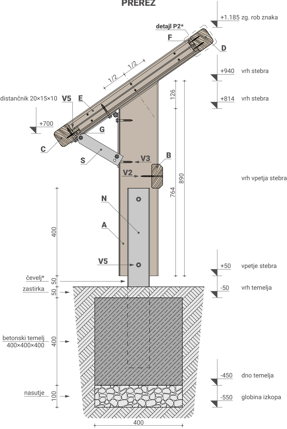
PREREZ
