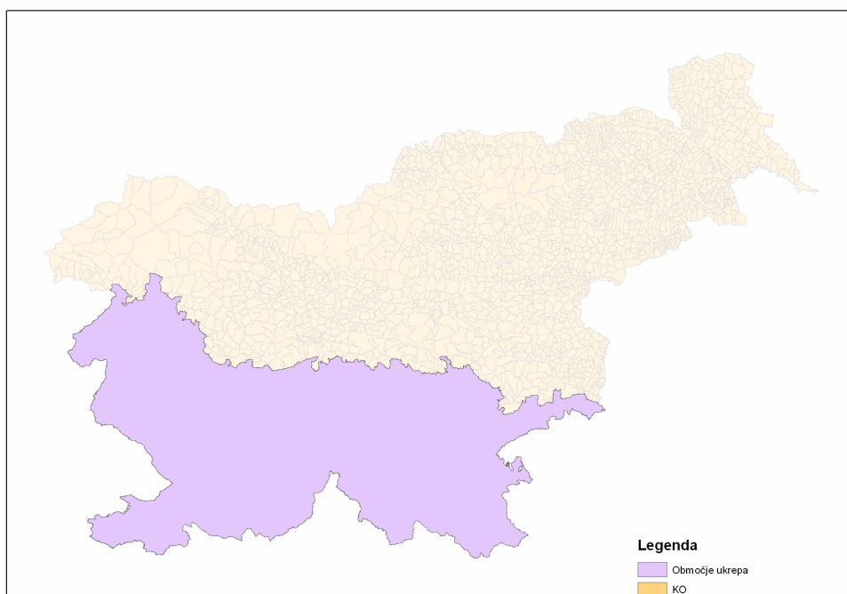
Slika 1: Območja ekstenzivnih kraških pašnikov
