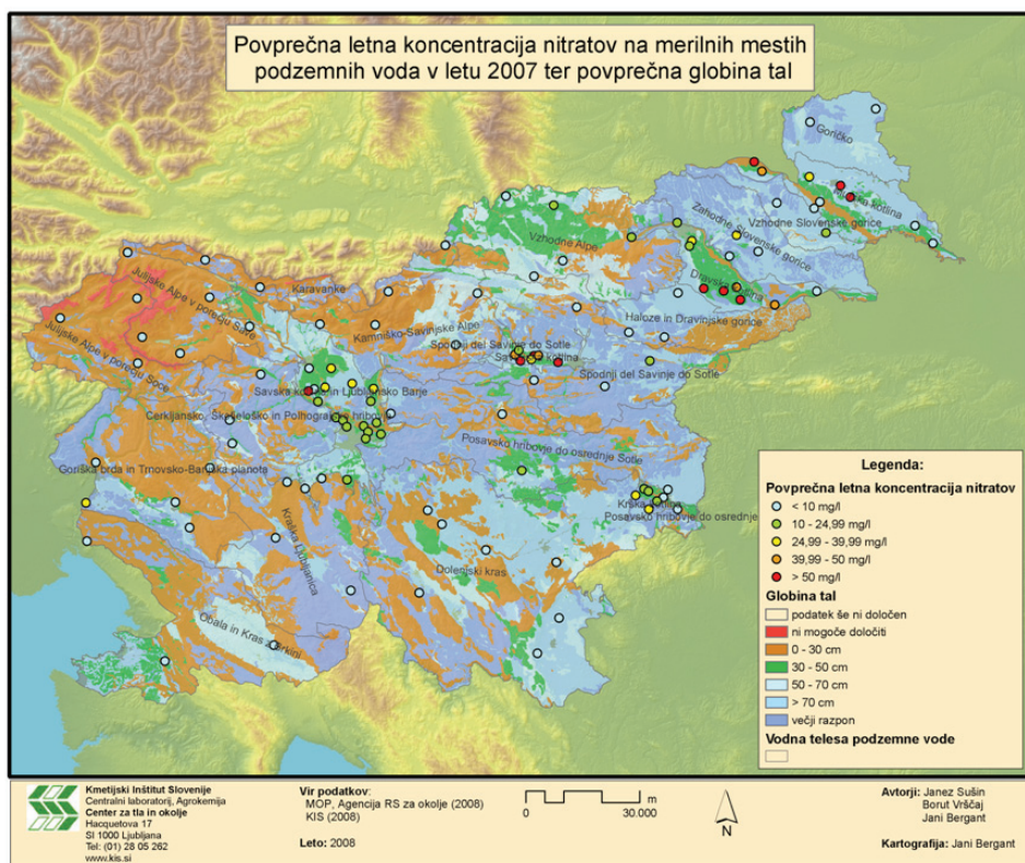
Slika 16: Povprečna koncentracija nitrata v podzemnih vodah v letu 2007 (Sušin in sod., 2008).
