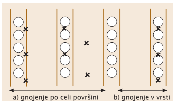
Slika 9: Vzorčenje tal za kontrolo rodovitnosti v trajnih nasadih je odvisno od načina gnojenja (a: povprek po celi površini ali b: samo v vrste, pod drevesne krošnje)
