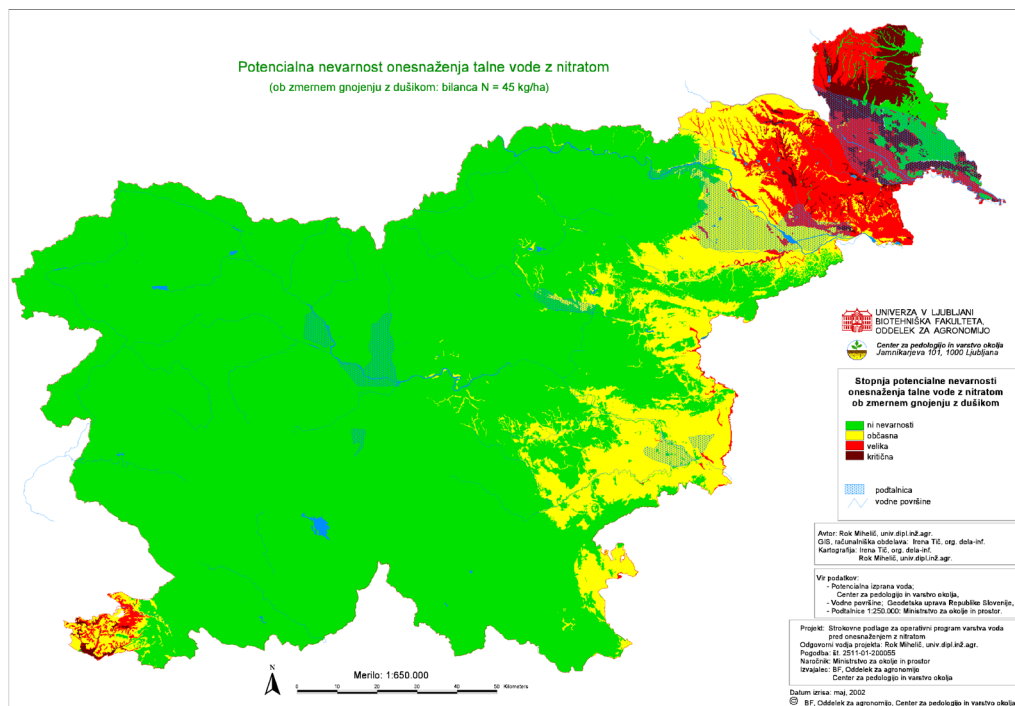
Slika 17: Potencialna nevarnost onesnaženja podtalnic z nitratom iz kmetijskih površin v Sloveniji pri zmernem gnojenju z N (letna bilanca N + 45 kg/ha) (Mihelič in sod., 2002)
