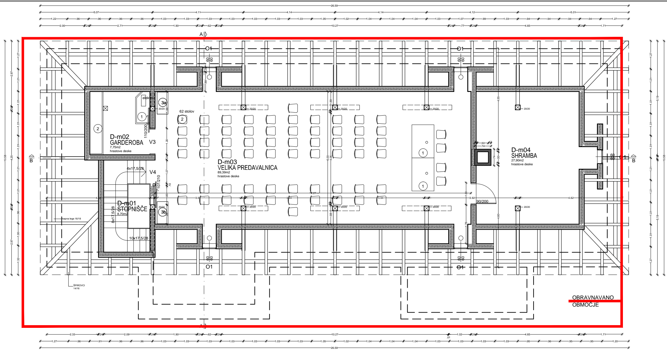
OBJEKT D, TLORIS MANSARDE, m 1:50
