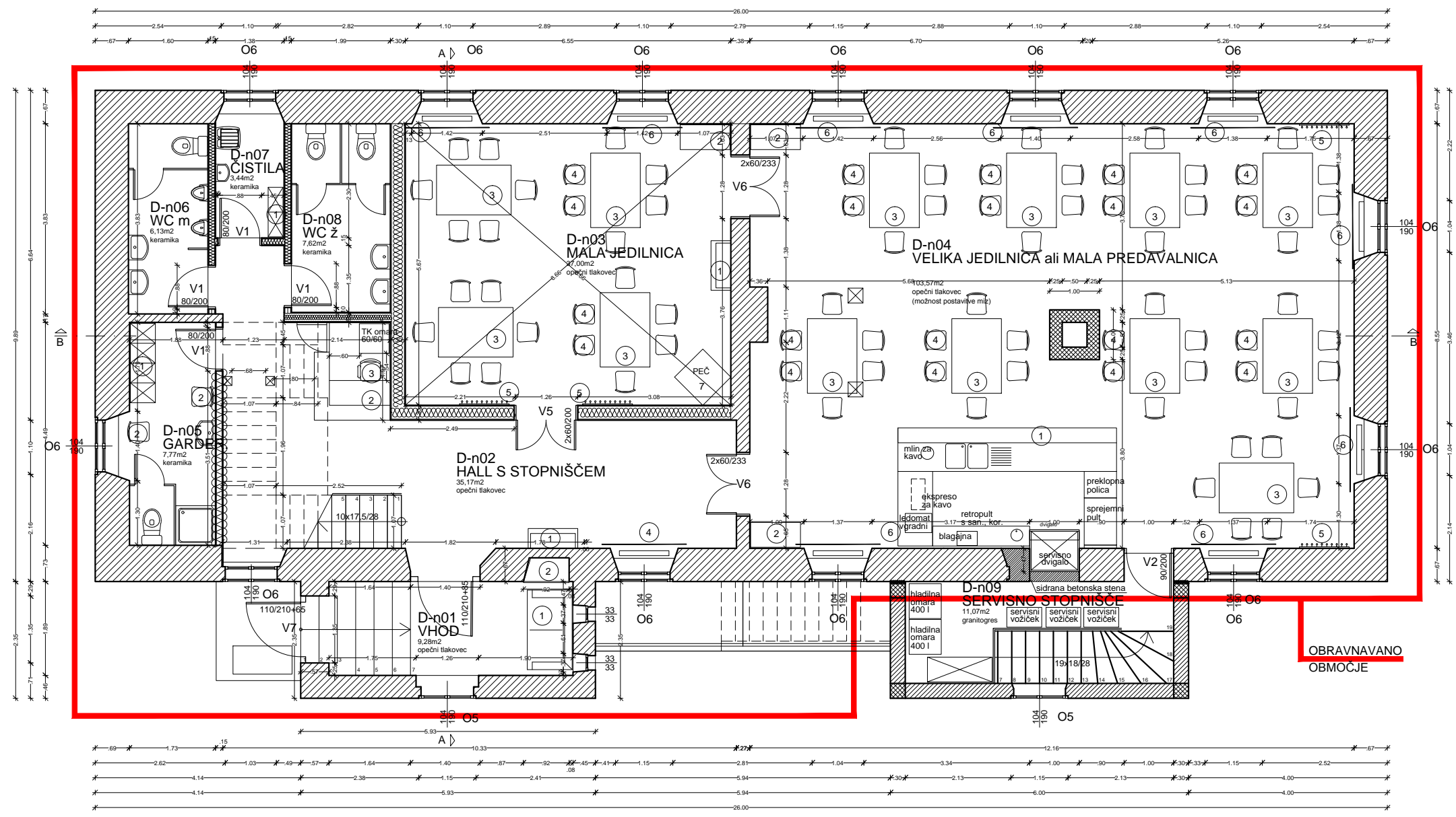
OBJEKT D, TLORIS NADSTROPJA, m 1:50
