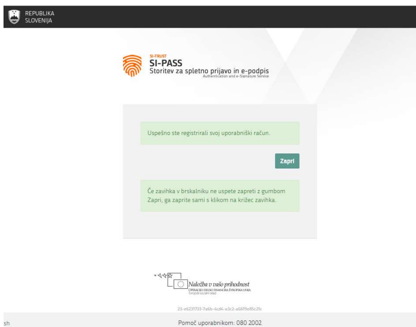
Slika 6: Zaključek registracije
