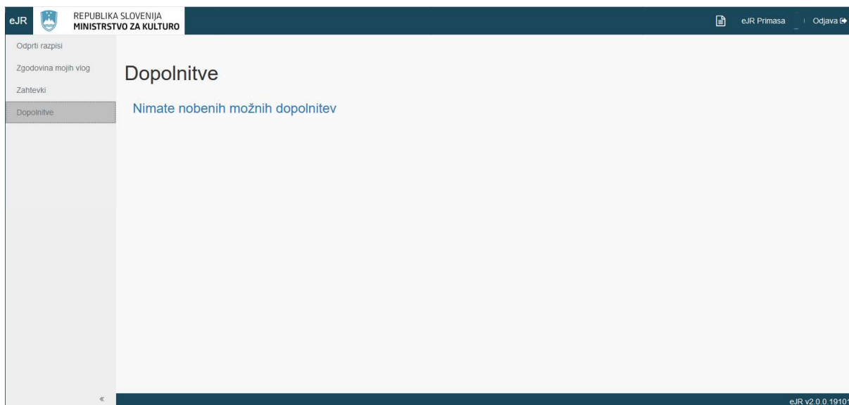
Slika 13: Dopolnitve vlog
