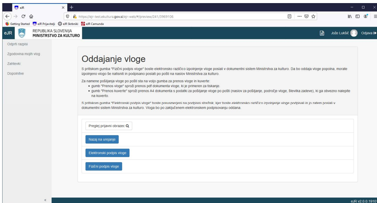
Slika 11: Oddajanje vloge
