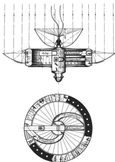
Vizionarska zasnova Hermana Potočnika Noordunga za vrtečo se vesoljsko postajo, ki bi bila sposobna vzdrževati človeško življenje v orbiti, 1928.
