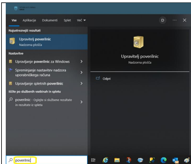
Slika 2 Iskanje poverilnic
