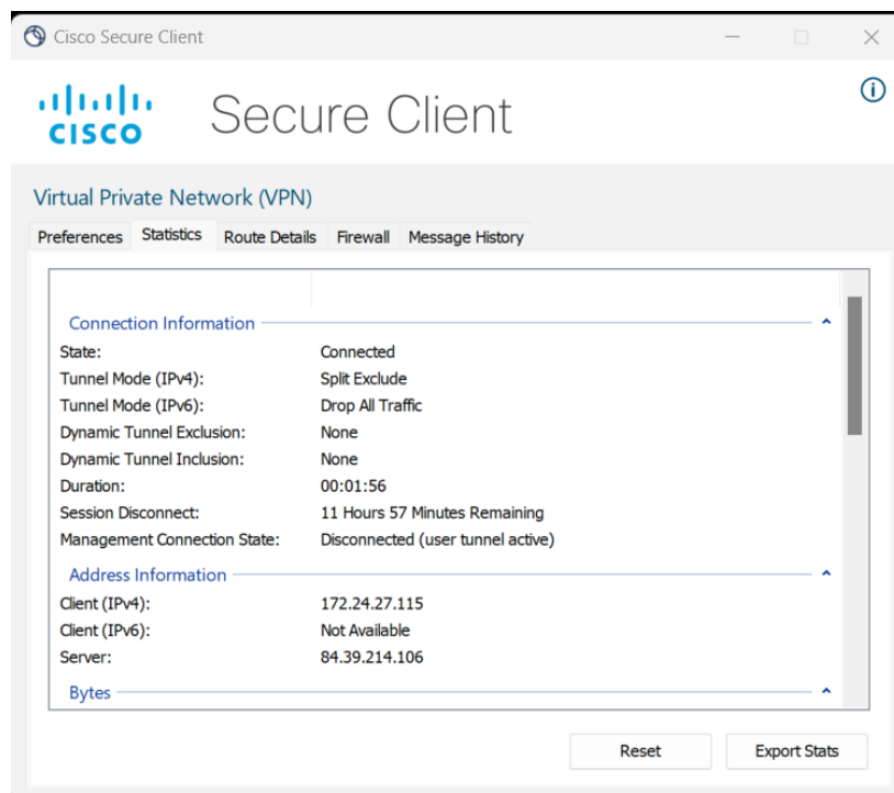
Slika 7: Podatki o vzpostavljeni povezavi
