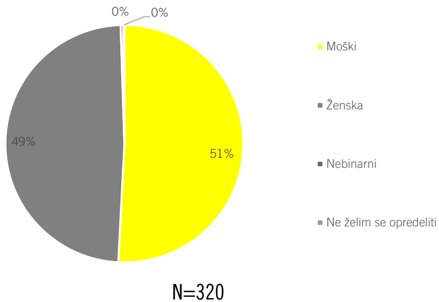
Slika 1: Spol
