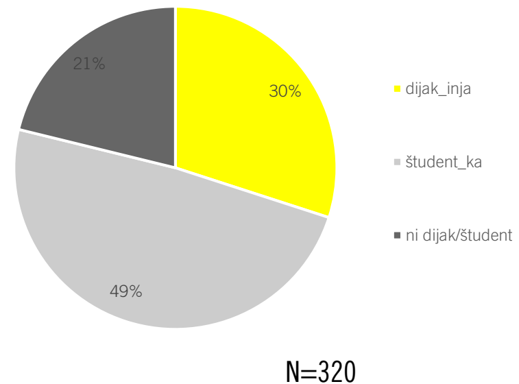
Slika 2: Status
